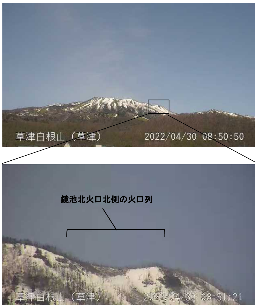
図8 草津白根山（本白根山） 本白根山付近の状況（草津監視カメラ）
