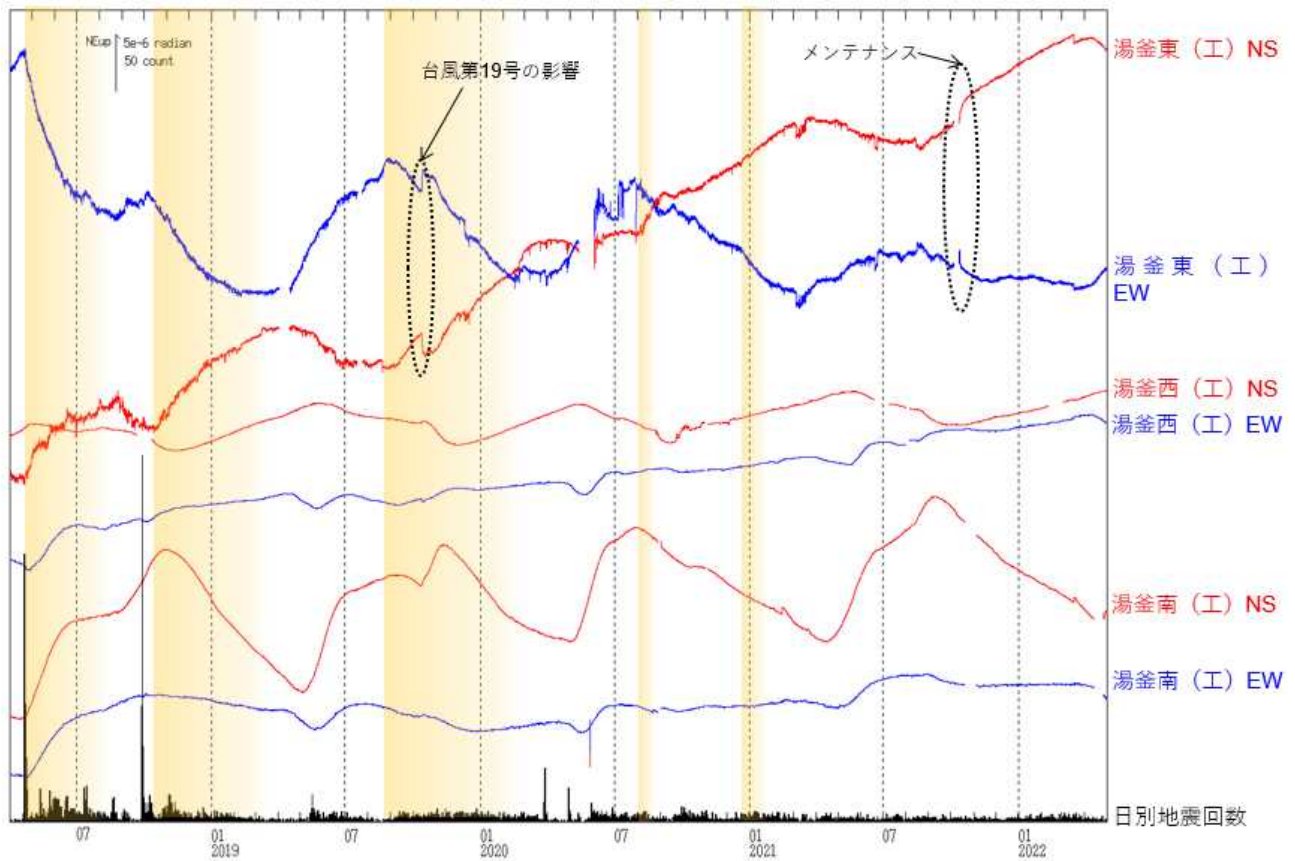
図5 草津白根山（白根山（湯釜付近）） 傾斜変動（2018年4月1日～2022年4月30日）
