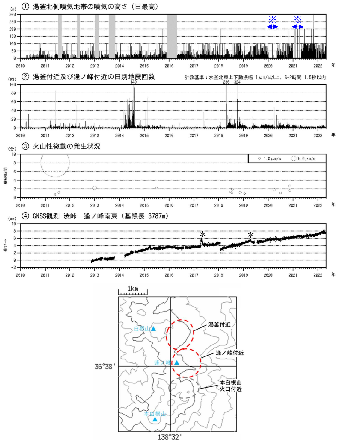
図3 草津白根山（白根山（湯釜付近）） 火山活動経過図（2010年1月1日～2022年4月30日）
