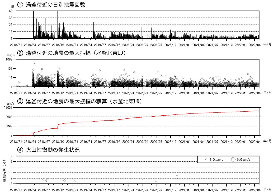
図1 草津白根山（白根山（湯釜付近）） 湯釜付近の地震活動及び火山性微動の発生状況 （2018年1月1日～2022年4月30日）
