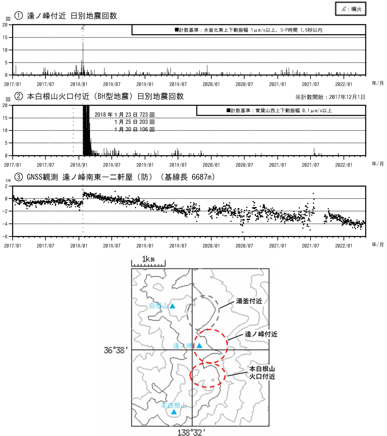
図9 草津白根山（本白根山） 火山活動経過図（2017年1月1日～2022年4月30日）
