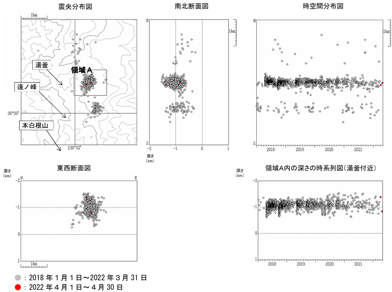
図4 草津白根山 震源分布図（2018年1月1日～2022年4月30日）
