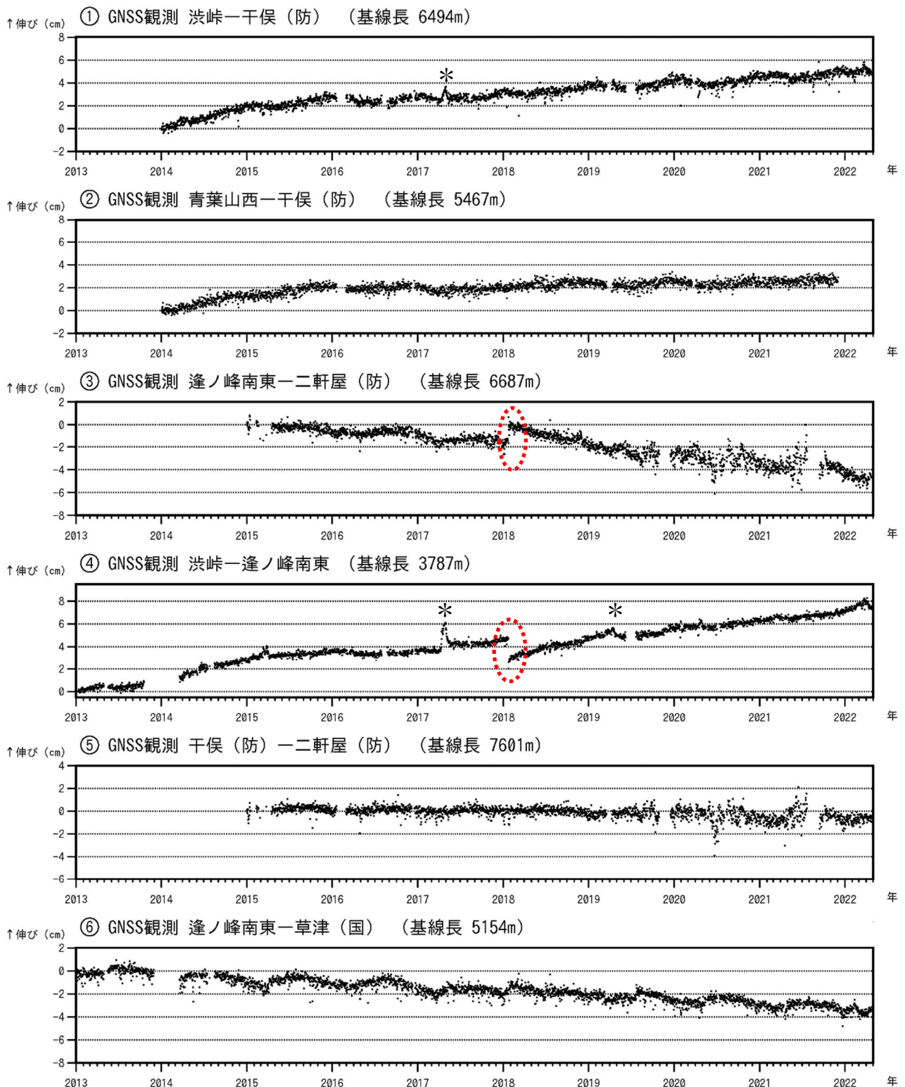
図6 草津白根山 GNSS 連続観測の結果 (2013 年 1 月 1 日～2022 年 4 月 30 日)
