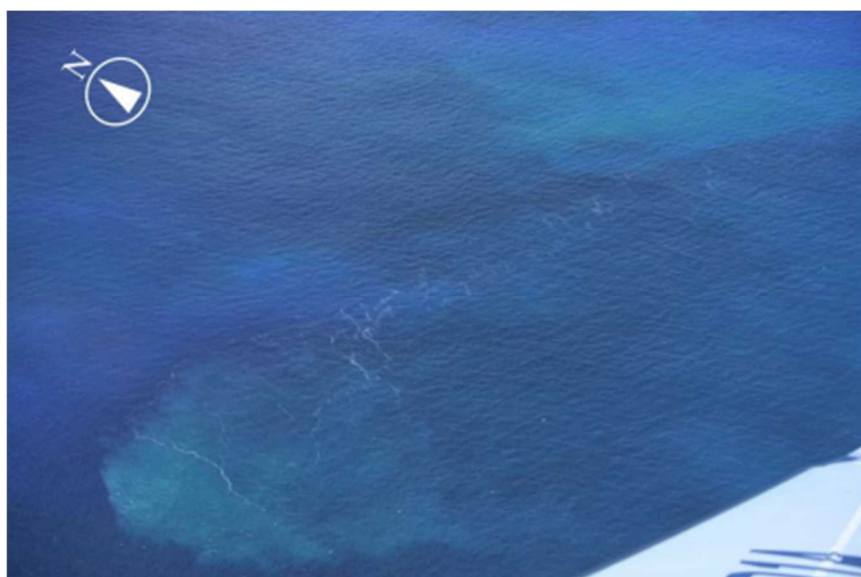
図1 福德岡ノ場 火口直上の状況（5月16日）
