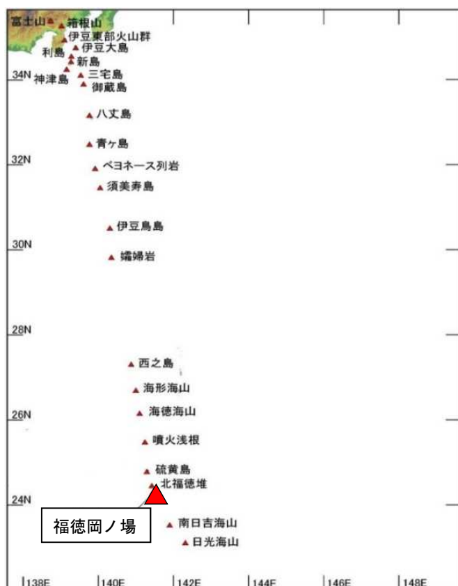
図3 福德岡ノ場 伊豆・小笠原諸島の 活火山分布と福德岡ノ場 地図は、日本活火山総覧（第4版）から引用。
