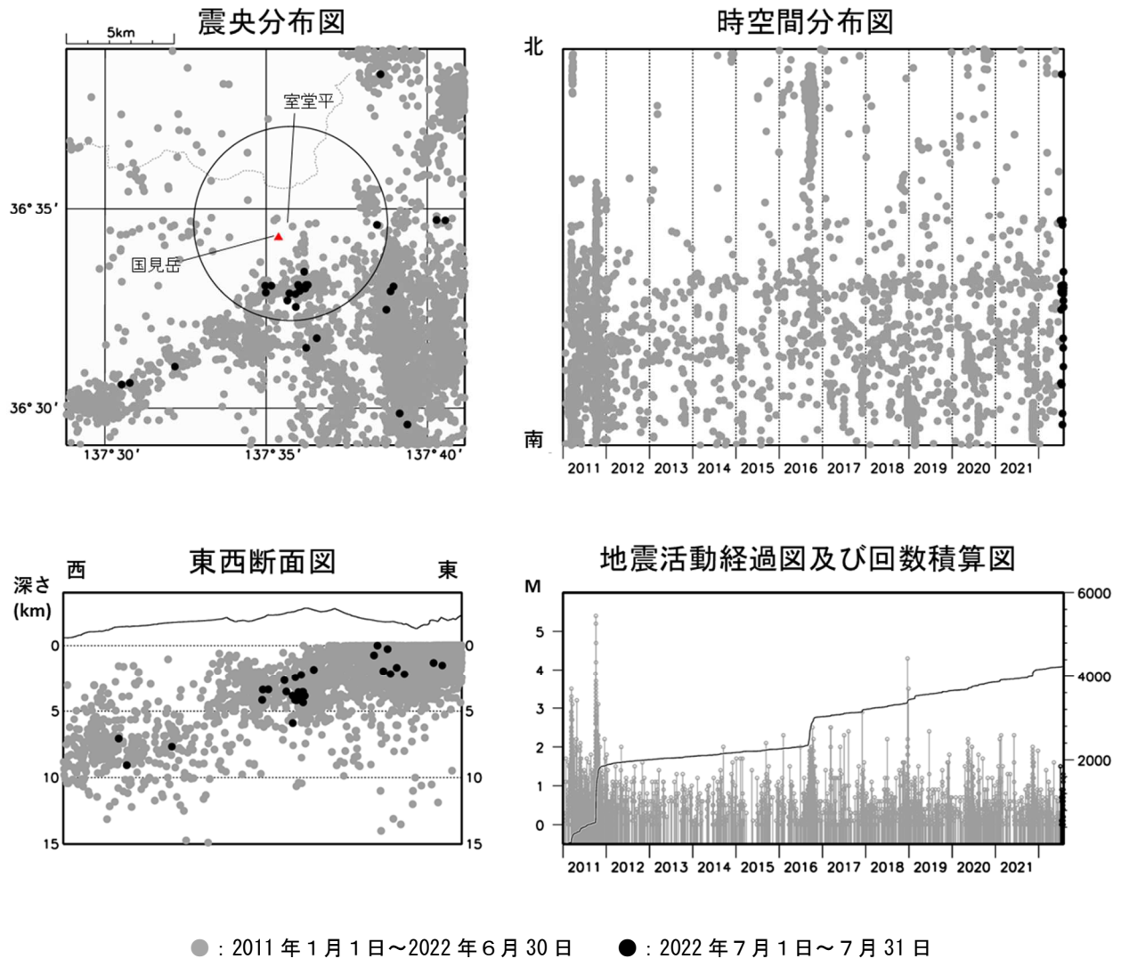
図2 弥陀ヶ原 広域地震観測網による山体・周辺の地震活動（2011 年 1 月 1 日～2022 年 7 月 31 日） 震央分布図中の円は弥陀ヶ原の計数対象地震（室堂平で S-P 時間 1 秒以内）のおよその範囲を示しています。 広域地震観測網により震源決定したもので、深さは全て海面以下として決定しています。 図中の震源要素は一部暫定値が含まれており、後日変更することがあります。 この図では、関係機関の地震波形を一元的に処理し、地震観測点の標高を考慮する等した手法で得られた震源を用いています（ただし、2020 年 8 月以前の地震については火山活動評価のための参考震源です）。
