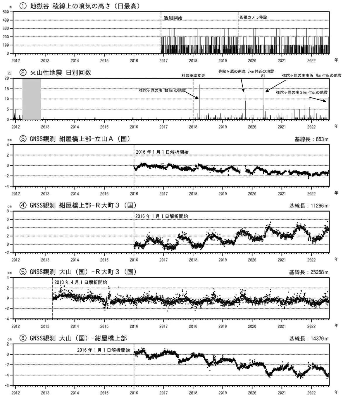
図3 弥陀ヶ原 火山活動経過図（2011年12月1日～2022年7月31日）
