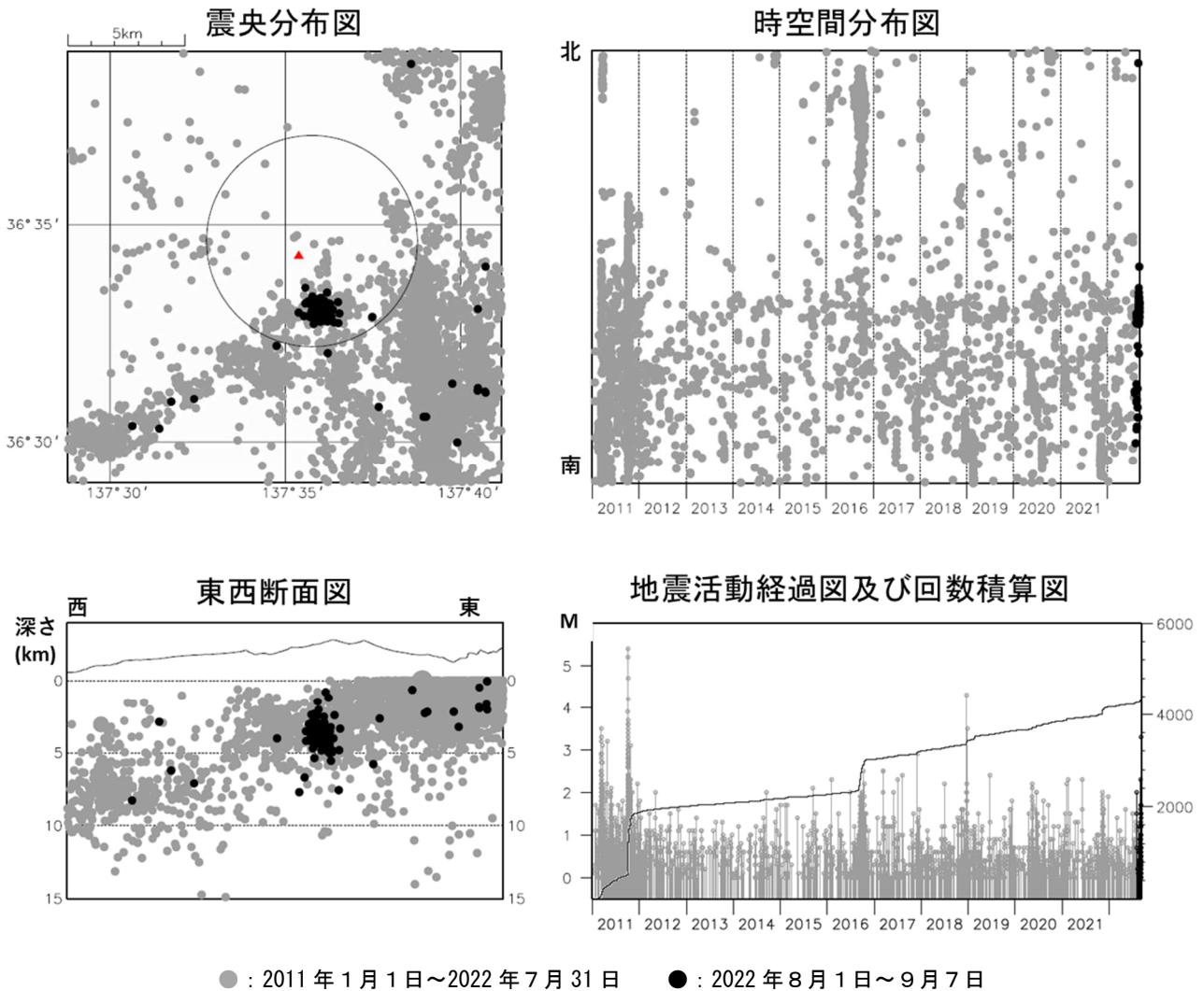
図2 弥陀ヶ原 広域地震観測網による山体・周辺の地震活動（2011 年 1 月 1 日～2022 年 9 月 7 日） 震央分布図中の円は弥陀ヶ原の計数対象地震（室堂平で S-P 時間 1 秒以内）のおよその範囲を示しています。 広域地震観測網により震源決定したもので、深さは全て海面以下として決定しています。 図中の震源要素は一部暫定値が含まれており、後日変更することがあります。 この図では、関係機関の地震波形を一元的に処理し、地震観測点の標高を考慮する等した手法で得られた震源を用いています（ただし、2020 年 8 月以前の地震については火山活動評価のための参考震源です）。
