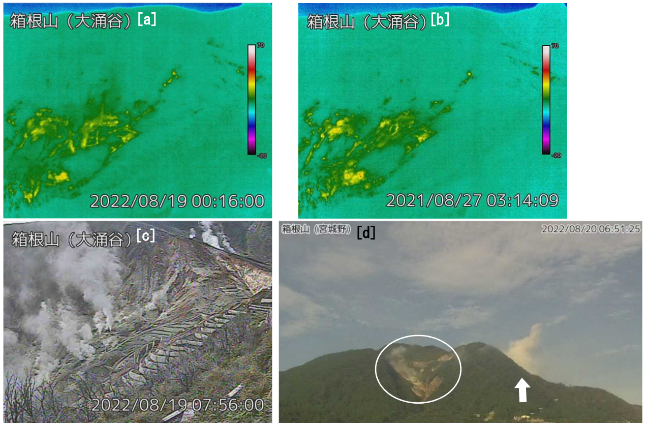
図1 箱根山 大涌谷及び早雲地獄の状況（a～c:大涌谷監視カメラによる、d:宮城野監視カメラによる） 円内は早雲地獄からの噴気の状況。
