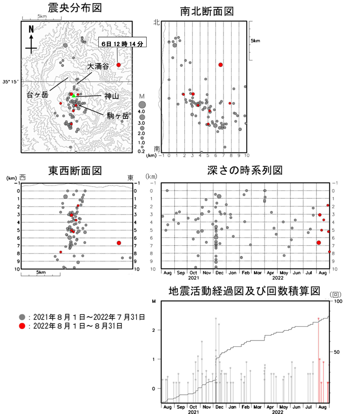
図4 箱根山 広域地震観測網による山体周辺の震源分布図（2021年8月1日～2022年8月31日）
