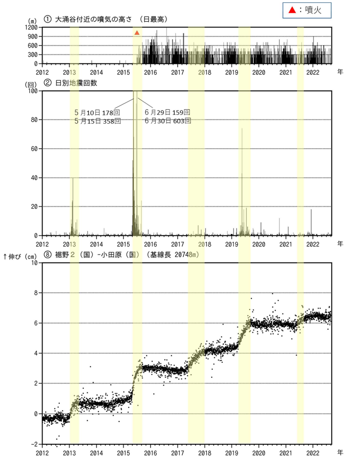
図3-1 箱根山 火山活動経過図（2012年1月1日～2022年8月31日）
