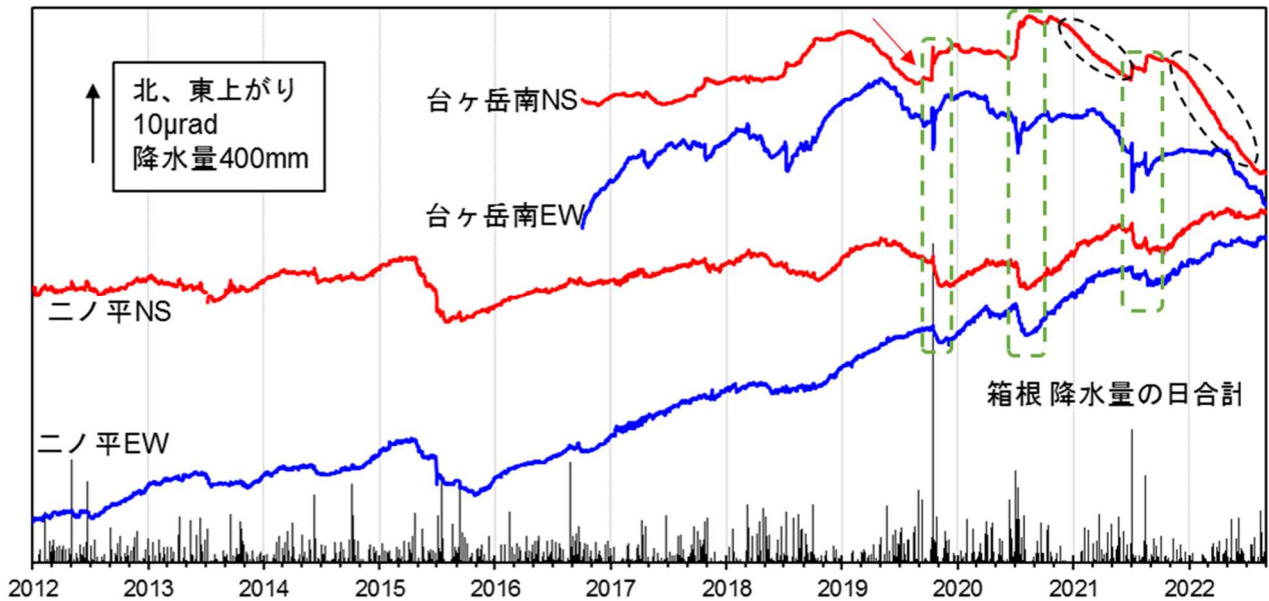
図5 箱根山 傾斜データ（2012年1月1日～2022年8月31日）
