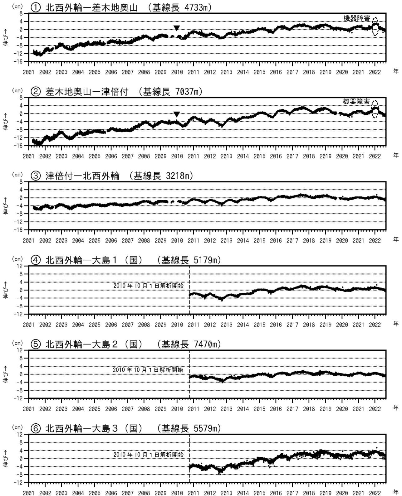
図3-1 伊豆大島 GNSS 連続観測による基線長変化(2001年1月～2022年8月31日)
