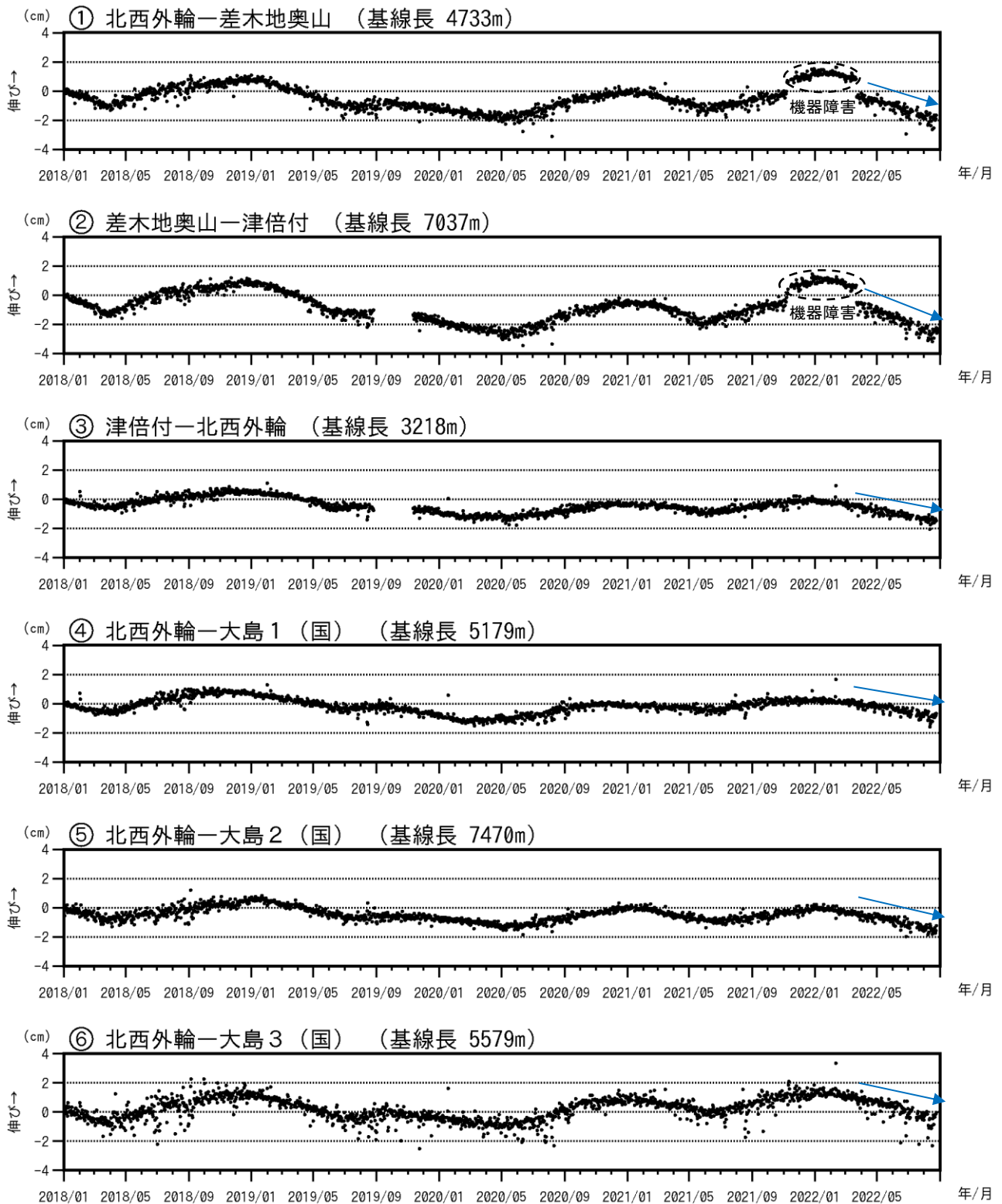
図3-2 伊豆大島 GNSS連続観測による基線長変化(2018年1月～2022年8月31日)
