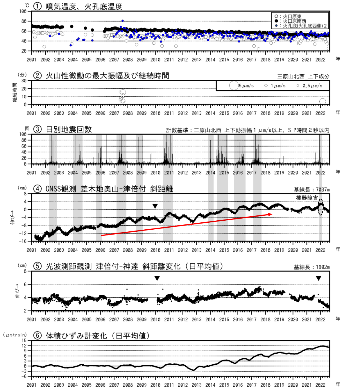
図2 伊豆大島 最近の火山活動経過図（2001年1月～2022年8月31日）
