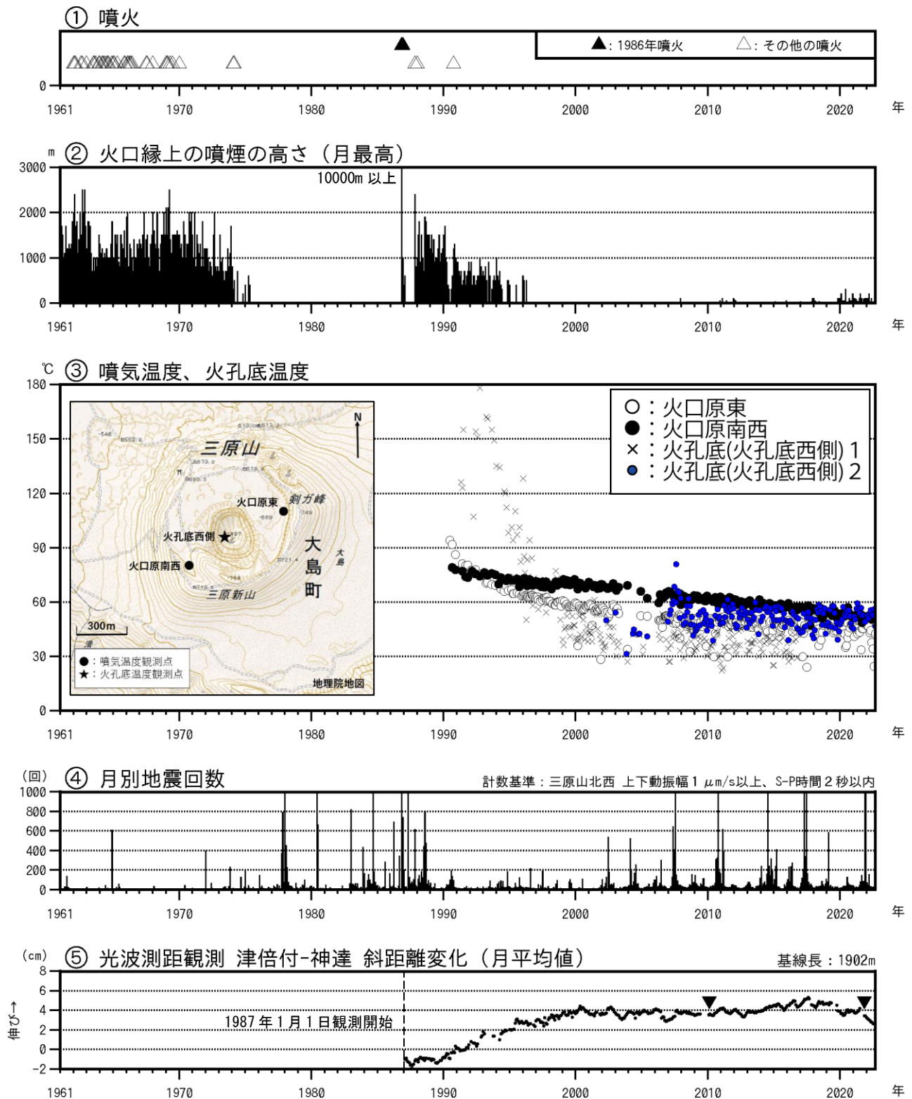
図1 伊豆大島 長期間の火山活動経過図（1961年1月～2022年8月31日）
