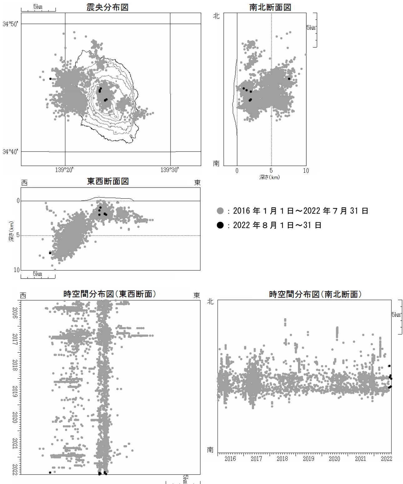
図4 伊豆大島 震源分布図（2016 年 1 月 1 日～2022 年 8 月 31 日）
