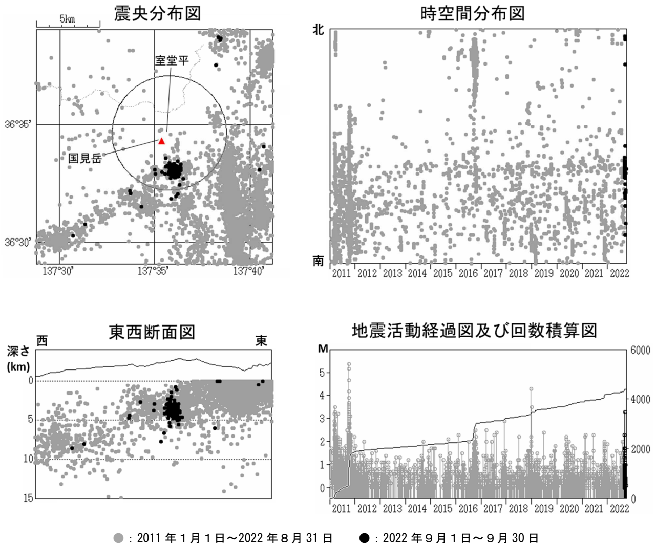
図2 弥陀ヶ原 広域地震観測網による山体・周辺の地震活動（2011 年 1 月 1 日～2022 年 9 月 30 日） 震央分布図中の円は弥陀ヶ原の計数対象地震（室堂平で S-P 時間 1 秒以内）のおよその範囲を示しています。 広域地震観測網により震源決定したもので、深さは全て海面以下として決定しています。 図中の震源要素は一部暫定値が含まれており、後日変更することがあります。 この図では、関係機関の地震波形を一元的に処理し、地震観測点の標高を考慮する等した手法で得られた震源を用いています（ただし、2020 年 8 月以前の地震については火山活動評価のための参考震源です）。
