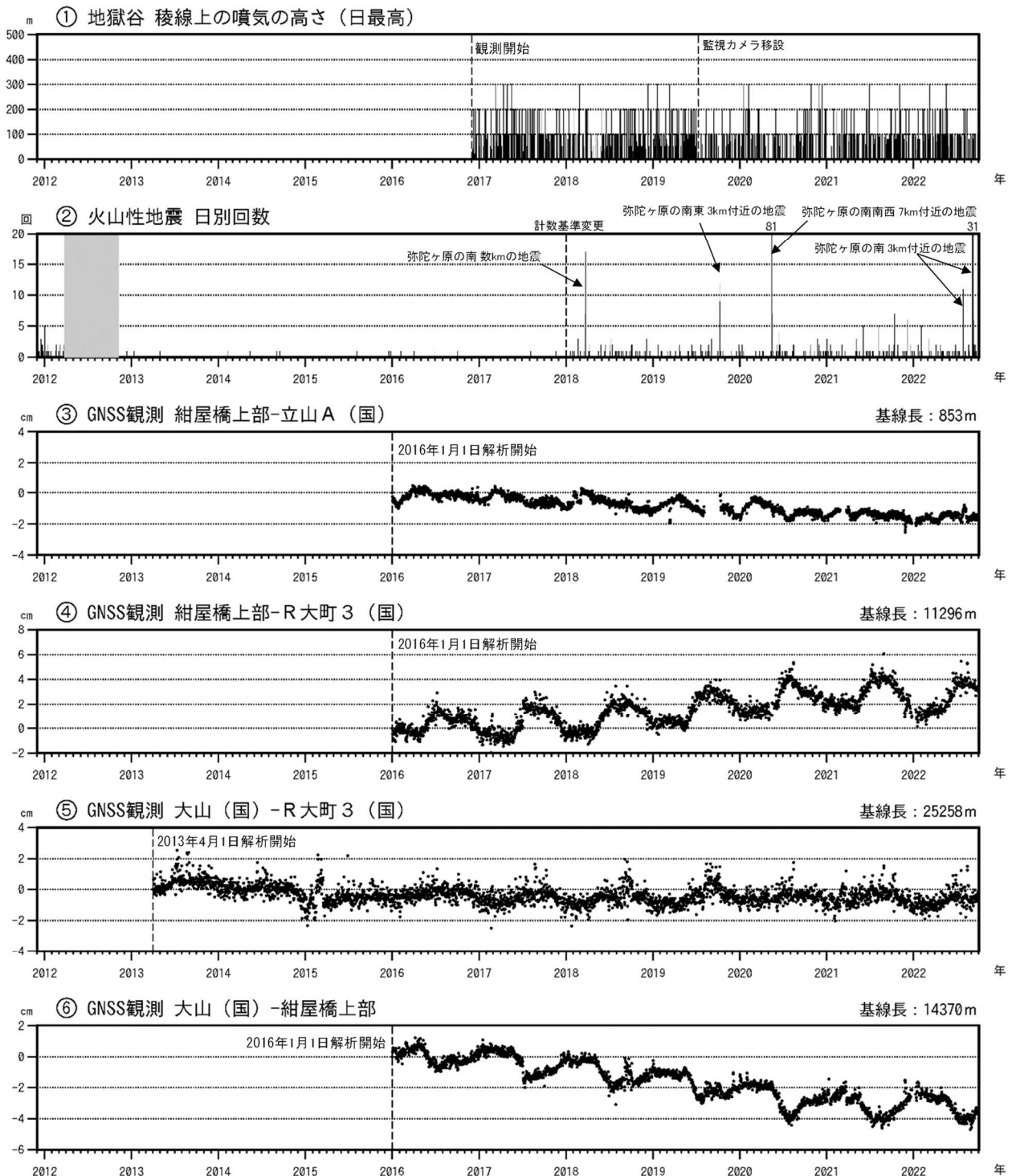
図3 弥陀ヶ原 火山活動経過図（2011年12月1日～2022年9月30日）
