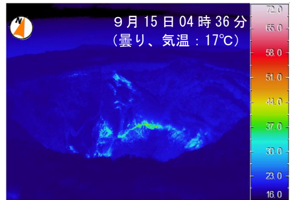
図5 伊豆大島 三原山山頂部及び山頂火口の状況（撮影方向は図8参照）
