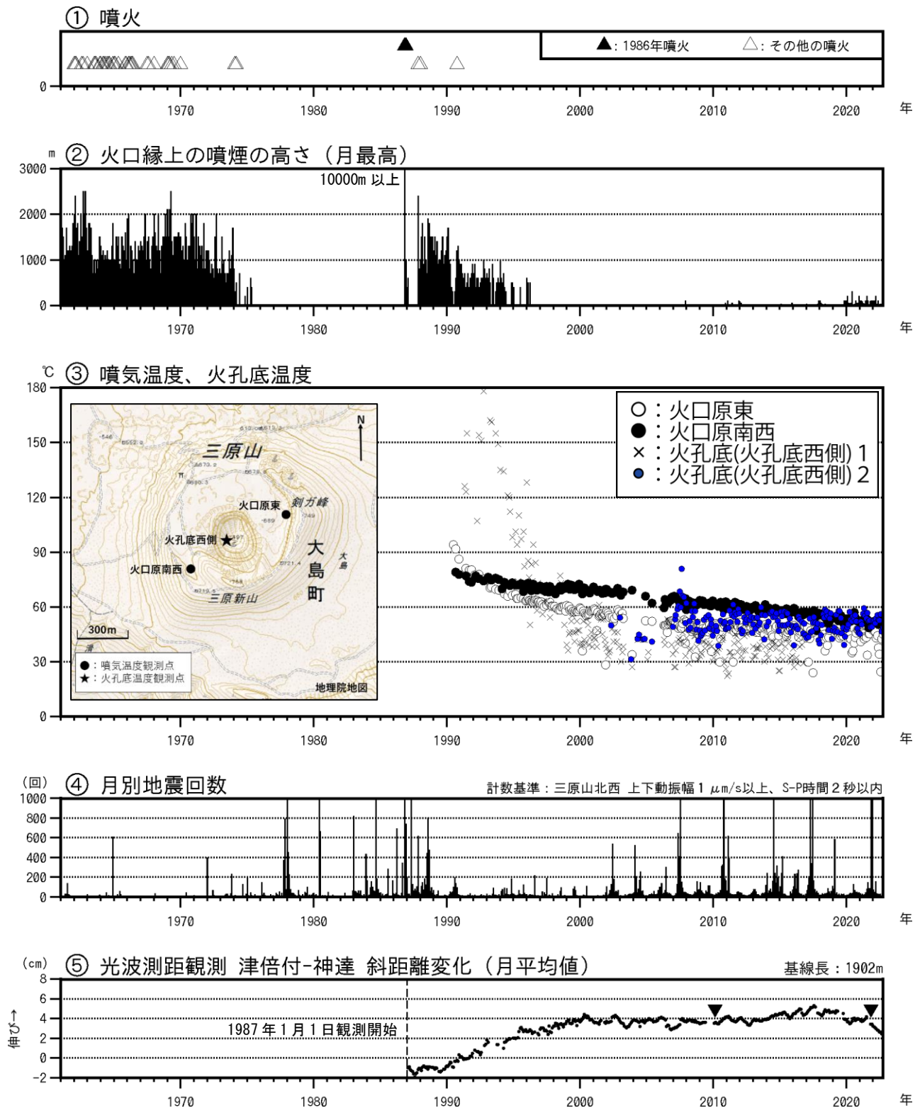
図1 伊豆大島 長期間の火山活動経過図（1961年1月～2022年9月30日）
