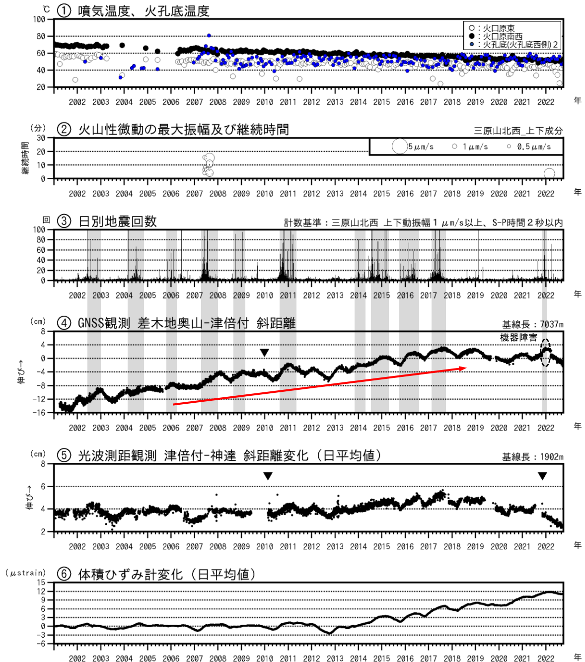
図2 伊豆大島 最近の火山活動経過図（2001年1月～2022年9月30日）
