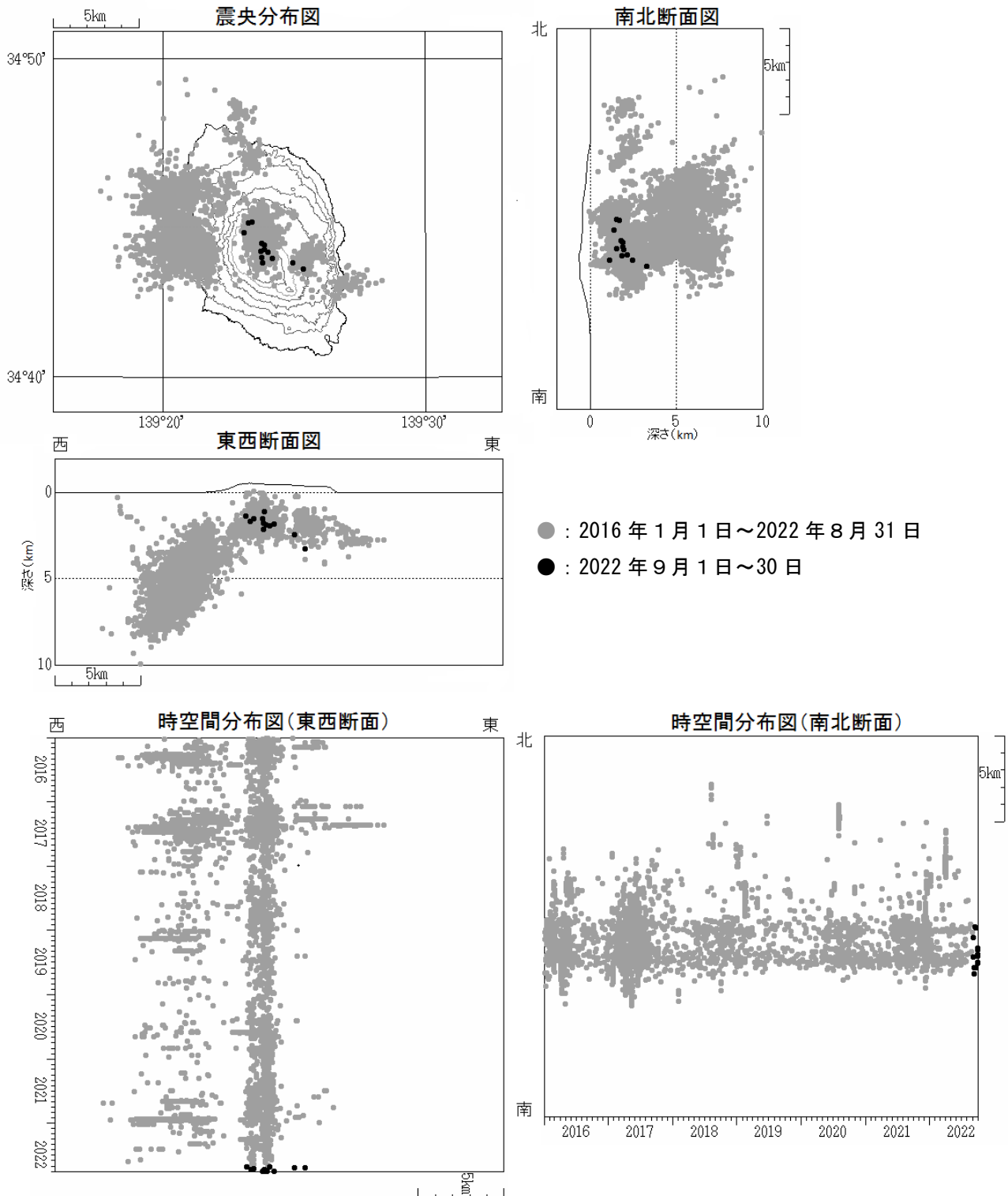
図4 伊豆大島 震源分布図（2016 年 1 月 1 日～2022 年 9 月 30 日）
