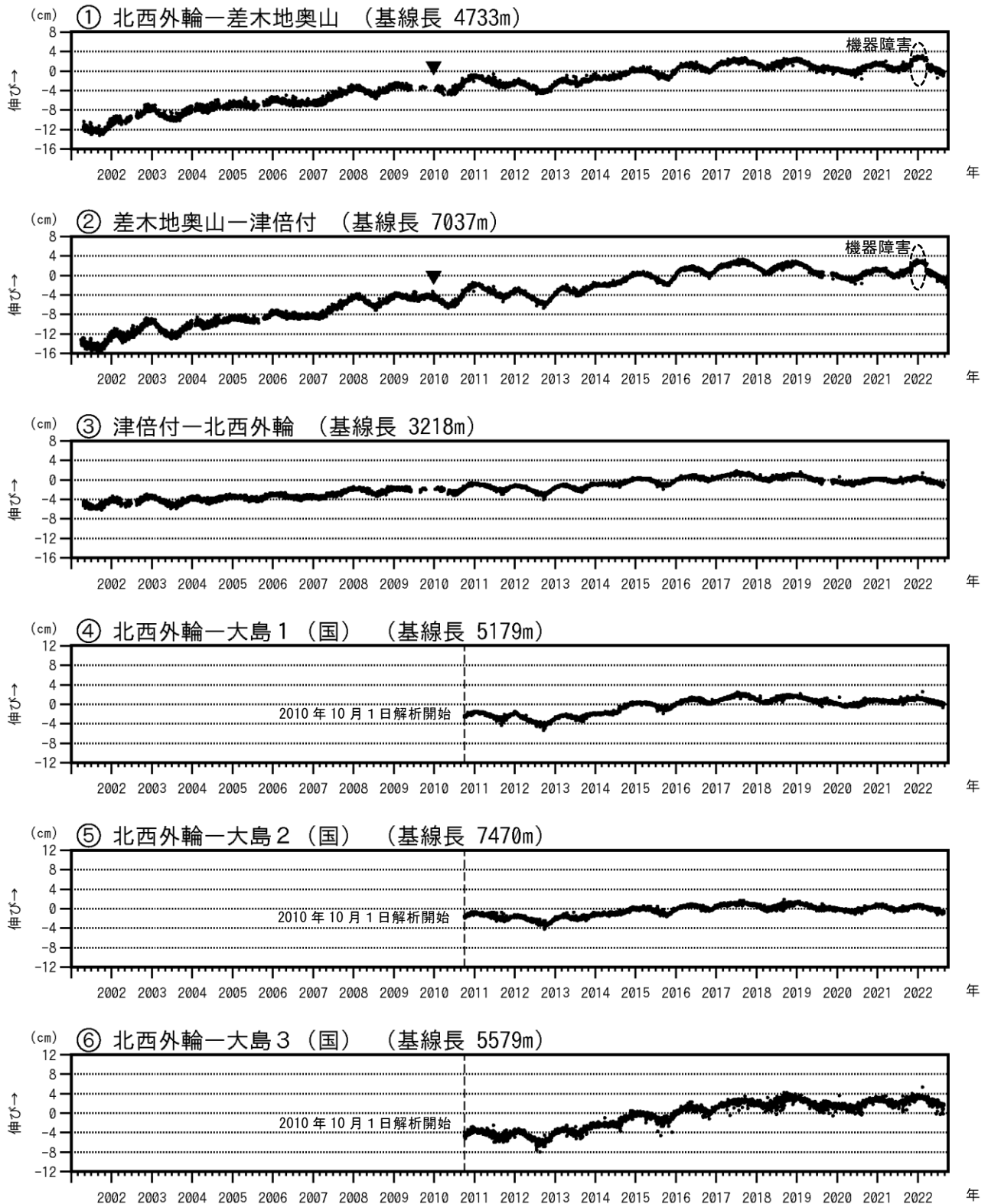
図3-1 伊豆大島 GNSS 連続観測による基線長変化(2001年1月～2022年9月30日)
