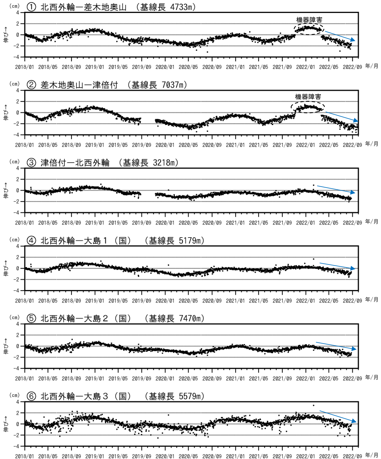
図3-2 伊豆大島 GNSS 連続観測による基線長変化(2018年1月～2022年9月30日)
