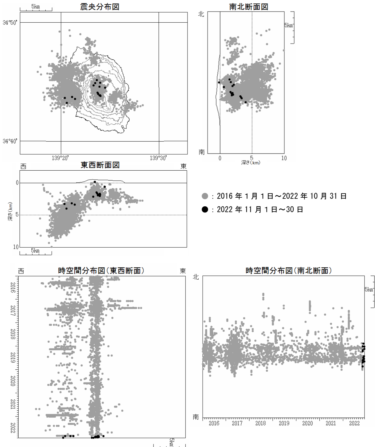
図4 伊豆大島 震源分布図（2016 年 1 月 1 日～2022 年 11 月 30 日）
