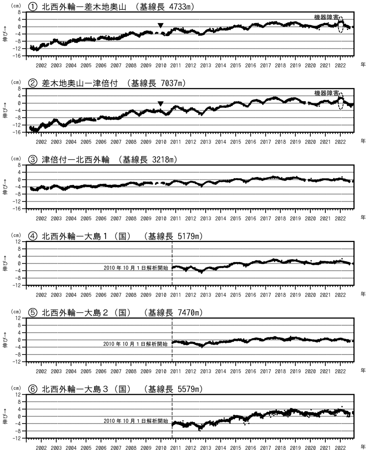
図3-1 伊豆大島 GNSS 連続観測による基線長変化(2001年1月～2022年11月30日)
