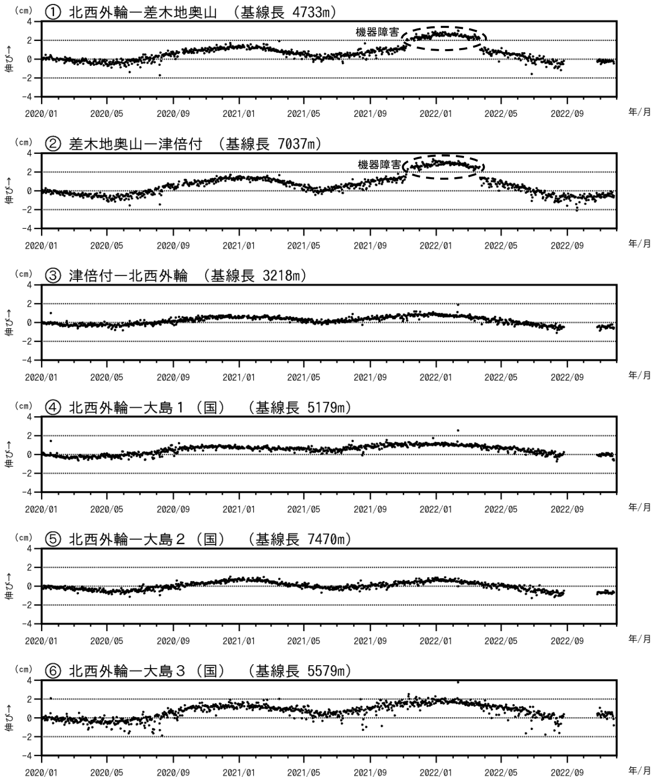
図3-2 伊豆大島 GNSS 連続観測による基線長変化(2020年1月～2022年11月30日)
