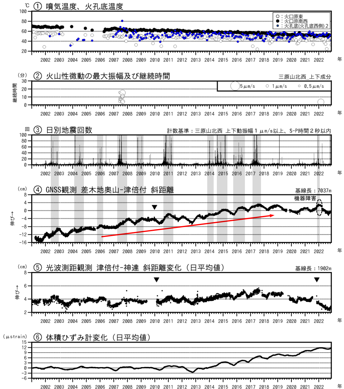
図2 伊豆大島 最近の火山活動経過図（2001年1月～2022年11月30日）
