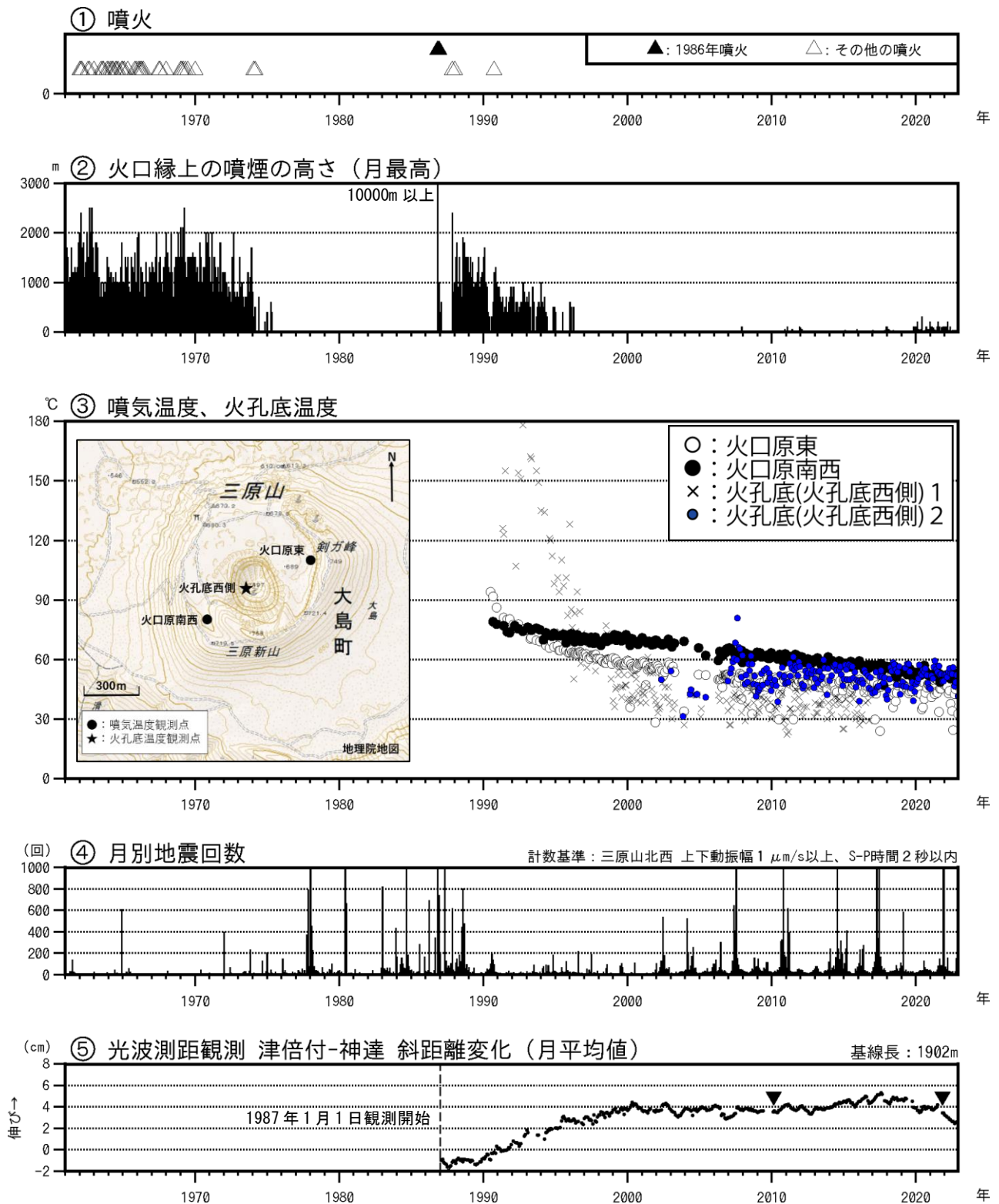
図1 伊豆大島 長期間の火山活動経過図（1961年1月～2022年11月30日）
