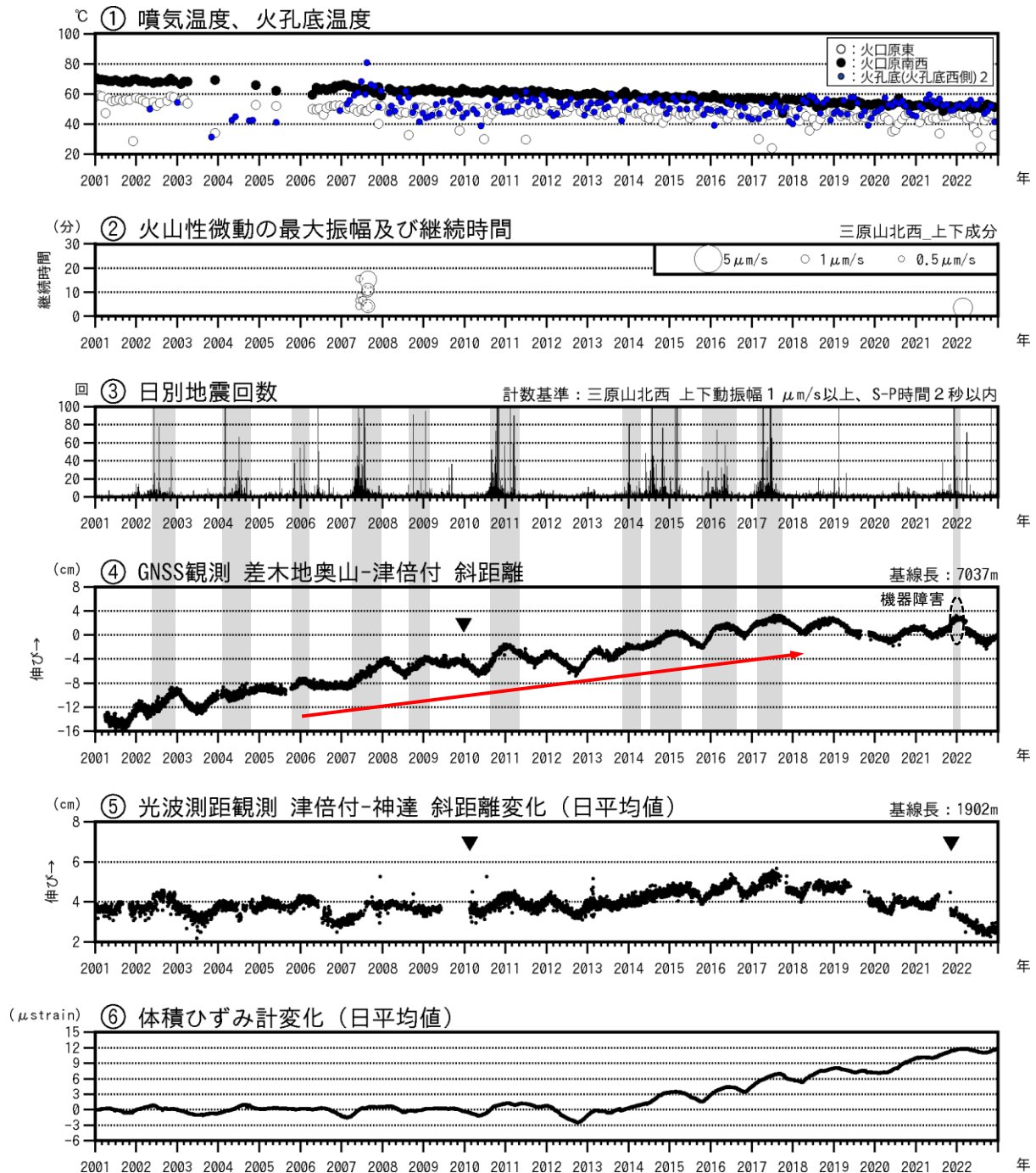
図2 伊豆大島 最近の火山活動経過図（2001年1月～2022年12月31日）
