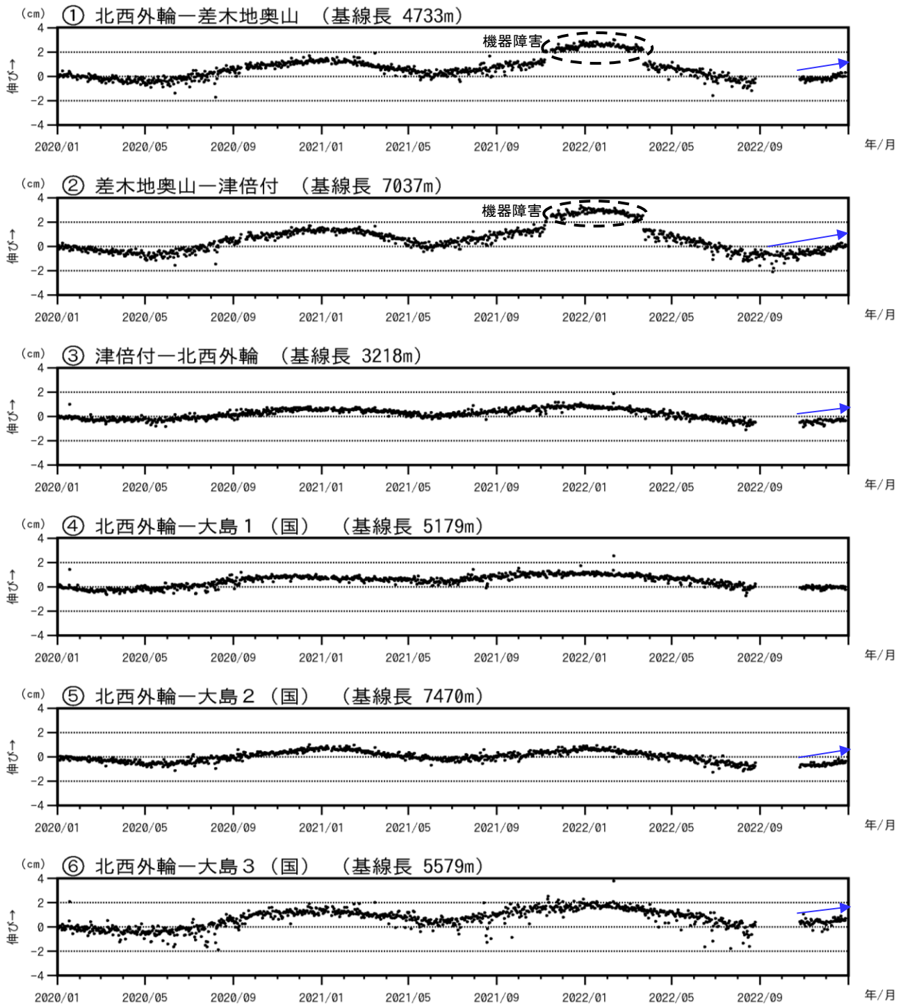
図3-2 伊豆大島 GNSS 連続観測による基線長変化(2020年1月～2022年12月31日)
