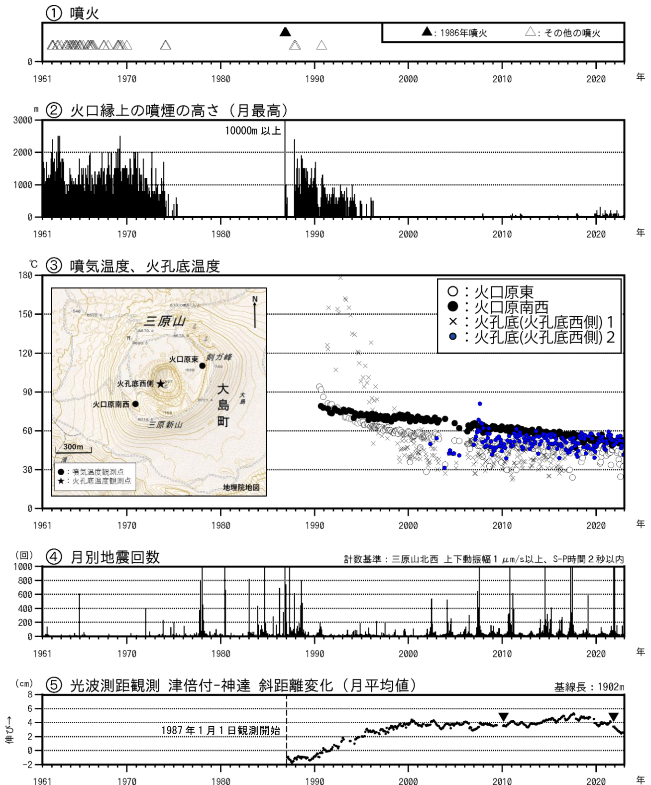
図1 伊豆大島 長期間の火山活動経過図（1961年1月～2022年12月31日）
