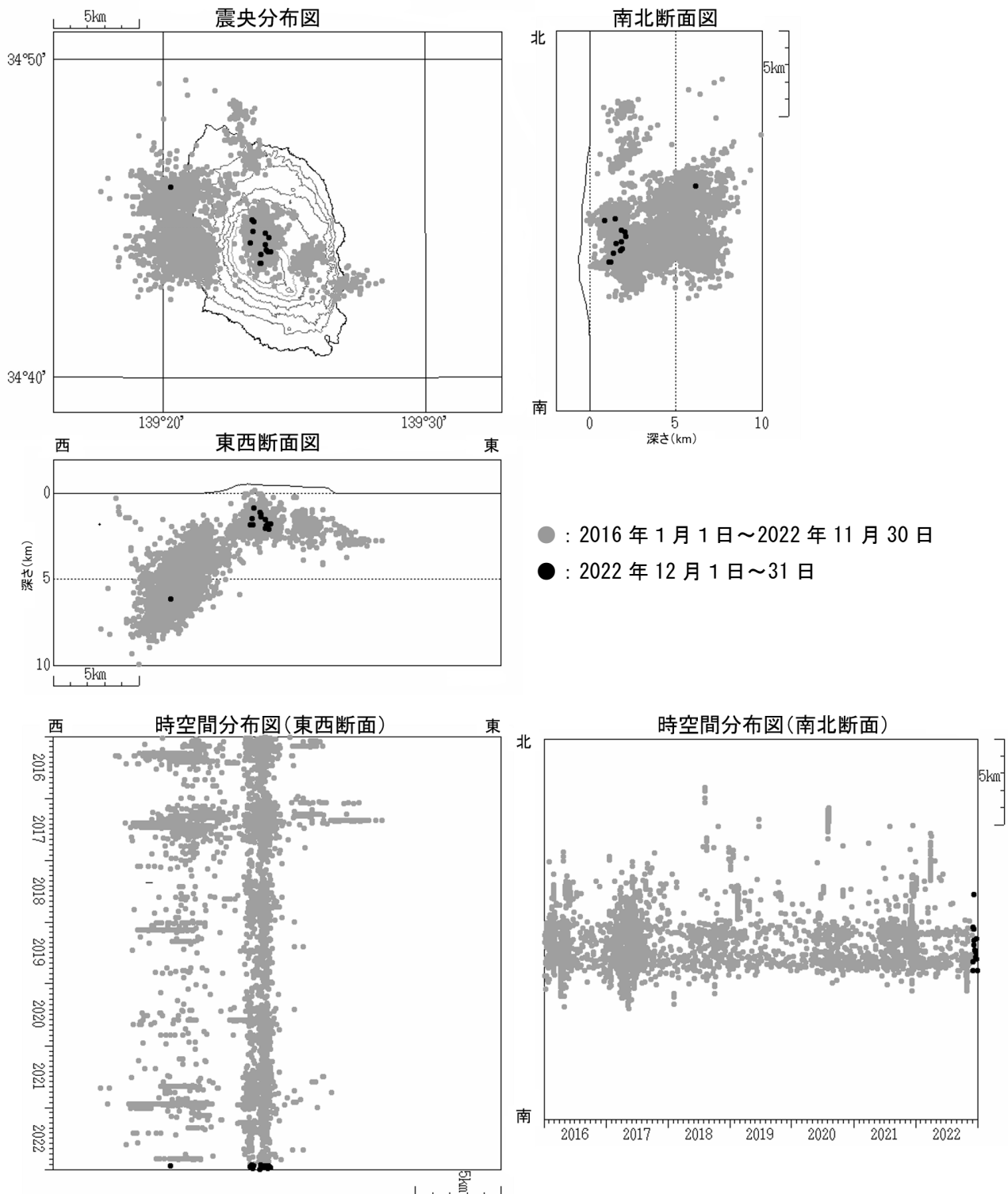
図4 伊豆大島 震源分布図（2016 年 1 月 1 日～2022 年 12 月 31 日）
