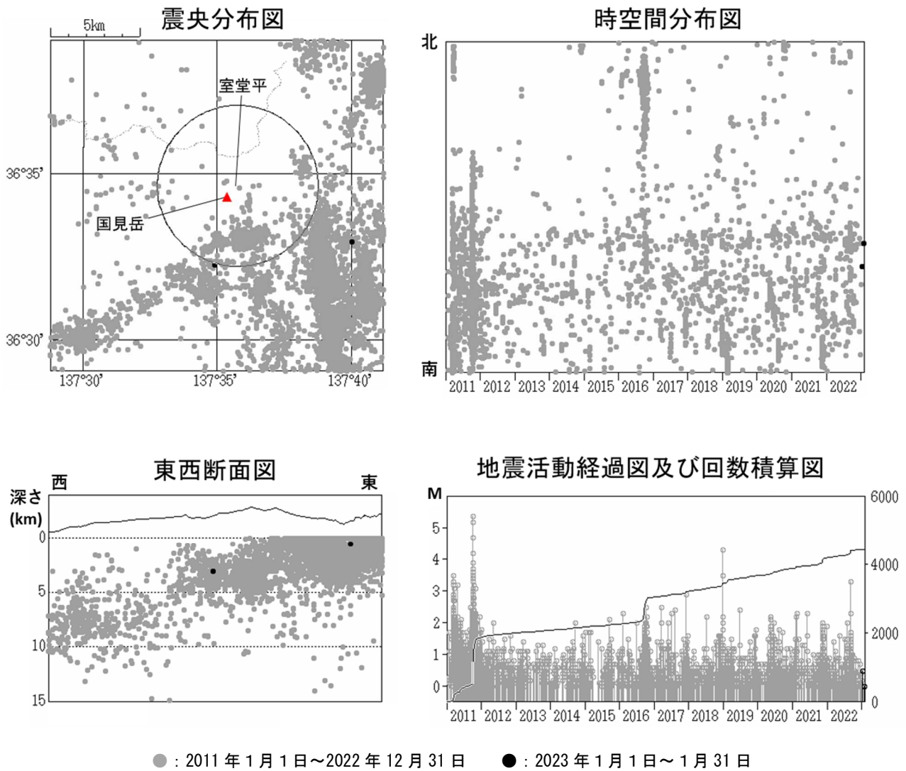
図2 弥陀ヶ原 広域地震観測網による山体・周辺の地震活動（2011年1月1日～2023年1月31日） 震央分布図中の円は弥陀ヶ原の計数対象地震（室堂平でS-P時間1秒以内）のおよその範囲を示しています。 広域地震観測網により震源決定したもので、深さは全て海面以下として決定しています。 図中の震源要素は一部暫定値が含まれており、後日変更することがあります。 この図では、関係機関の地震波形を一元的に処理し、地震観測点の標高を考慮する等した手法で得られた震源を用いています（ただし、2020年8月以前の地震については火山活動評価のための参考震源です）。
