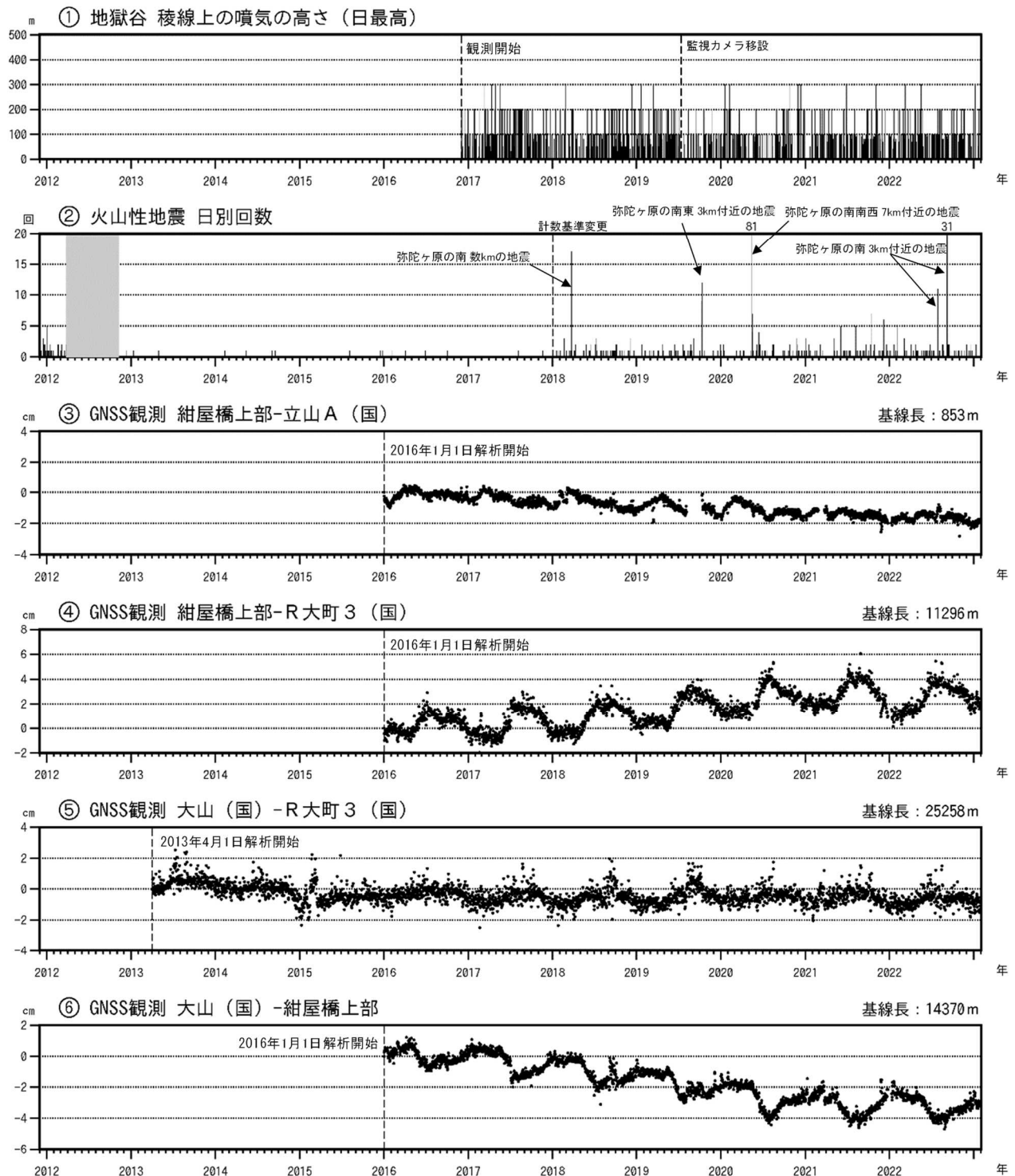
図3 弥陀ヶ原 火山活動経過図（2011年12月1日～2023年1月31日）
