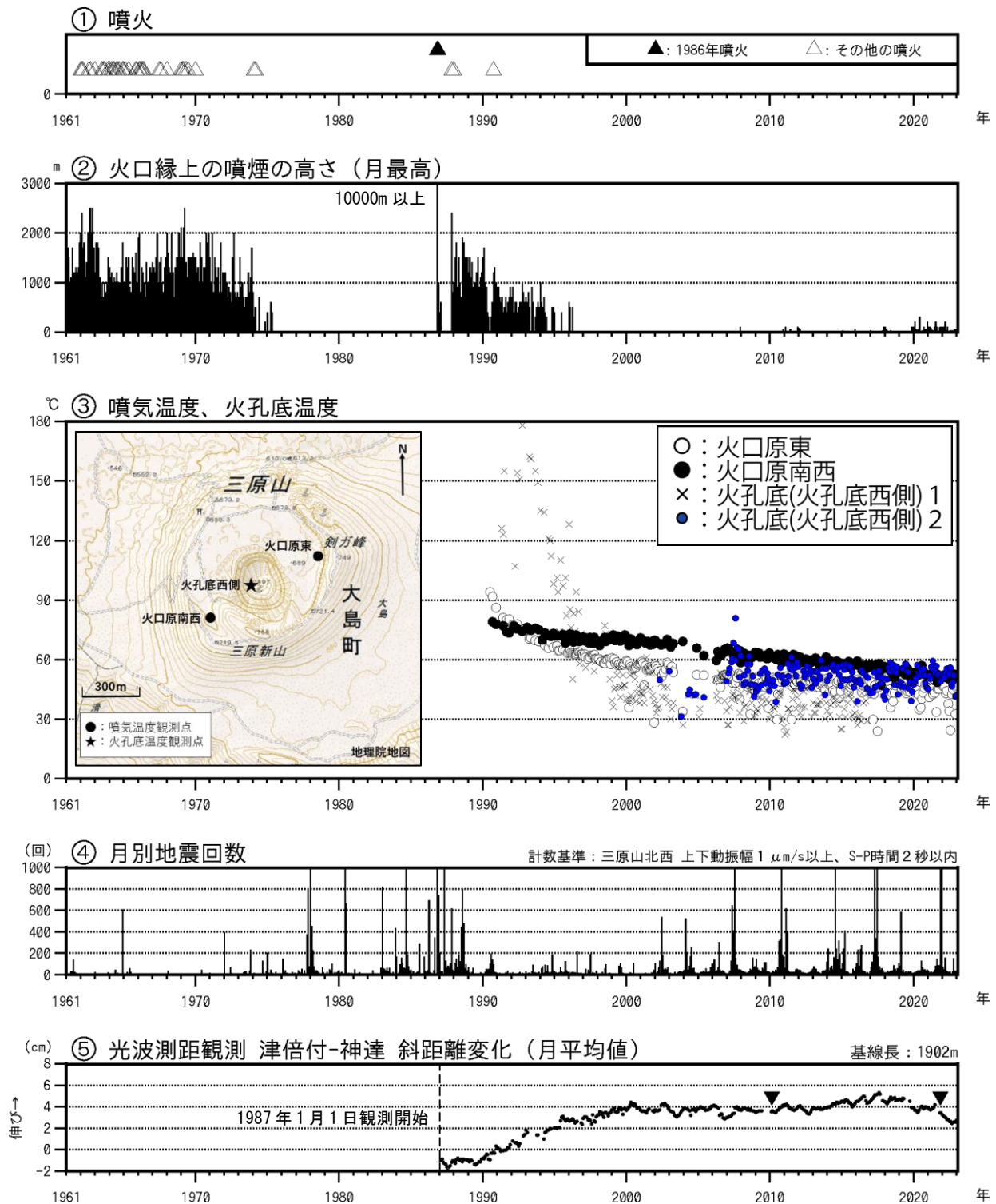
図1 伊豆大島 長期間の火山活動経過図（1961年1月～2023年1月31日）
