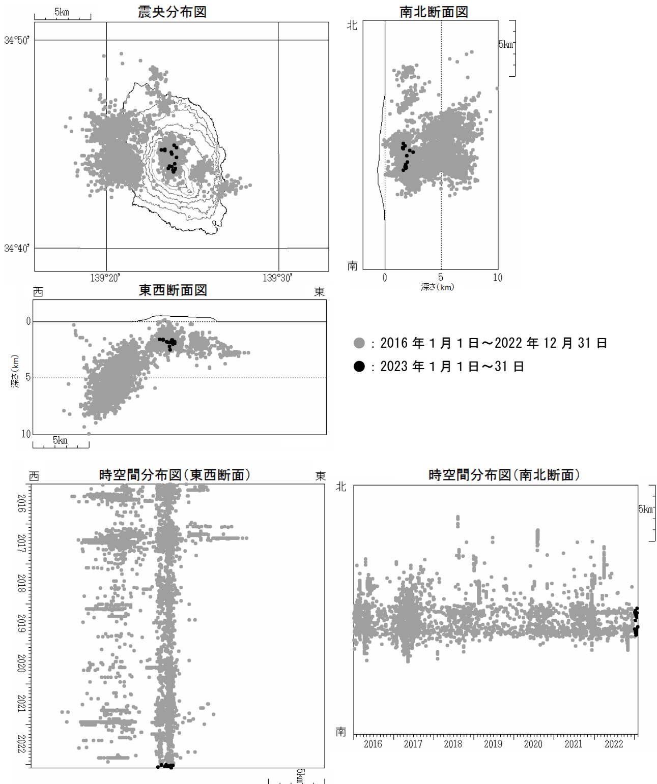
図4 伊豆大島 震源分布図（2016 年 1 月 1 日～2023 年 1 月 31 日）
