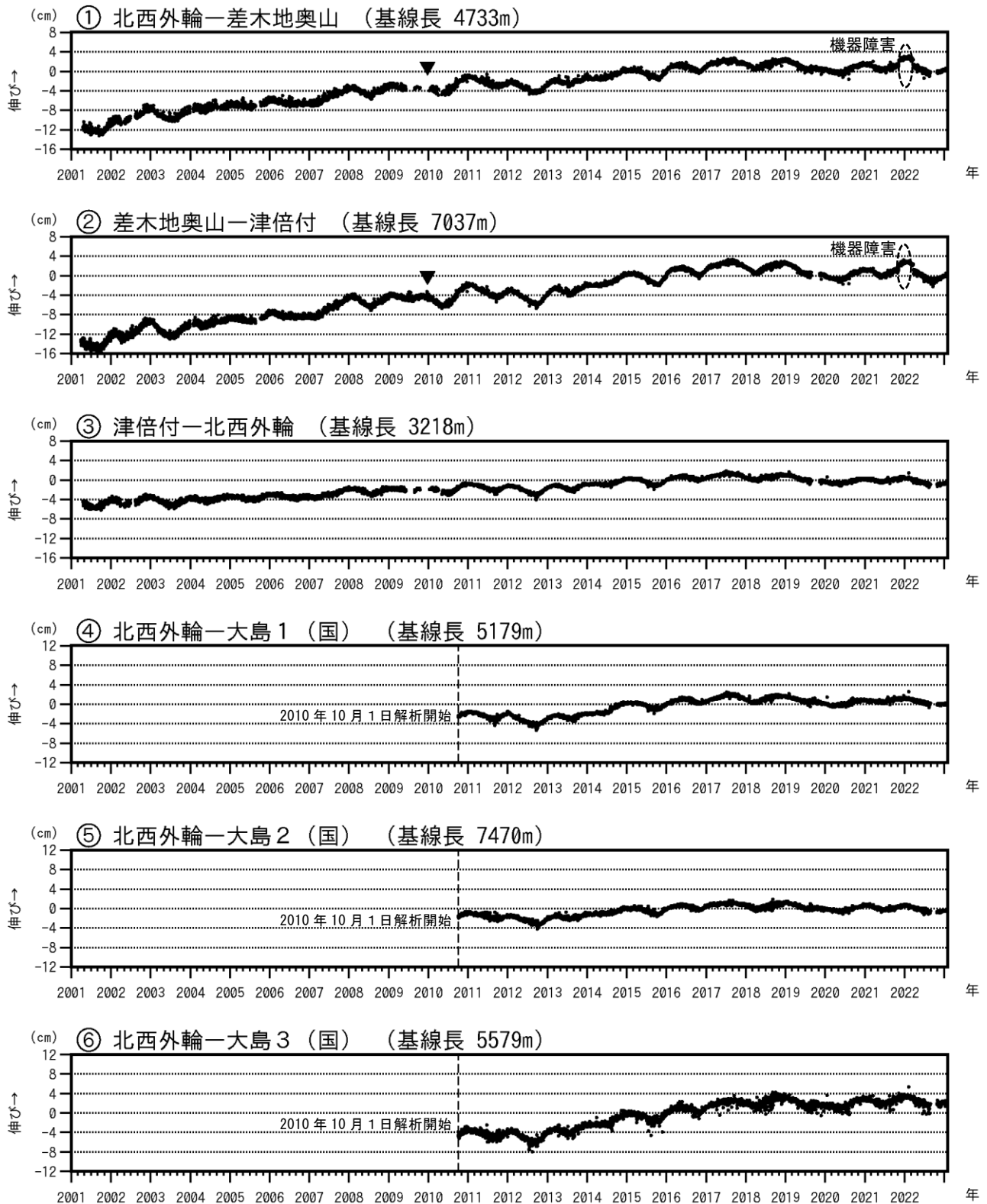
図3-1 伊豆大島 GNSS 連続観測による基線長変化(2001年1月～2023年1月31日)
