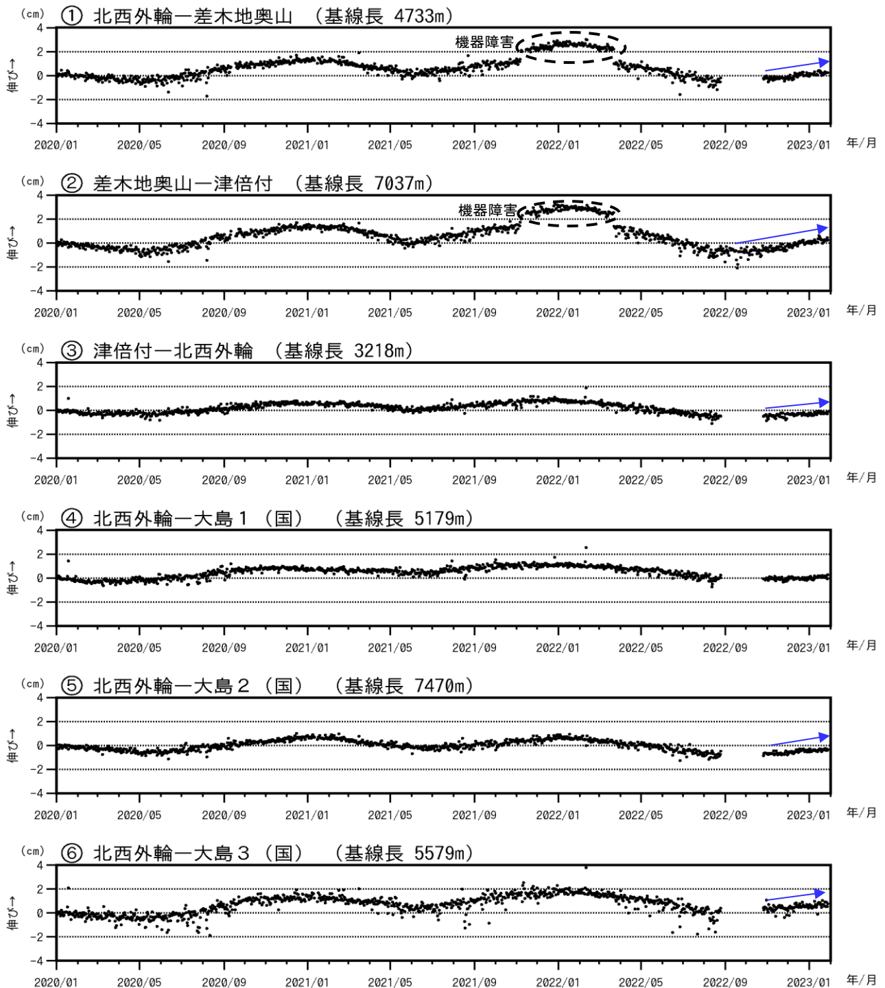
図3-2 伊豆大島 GNSS 連続観測による基線長変化(2020年1月～2023年1月31日)
