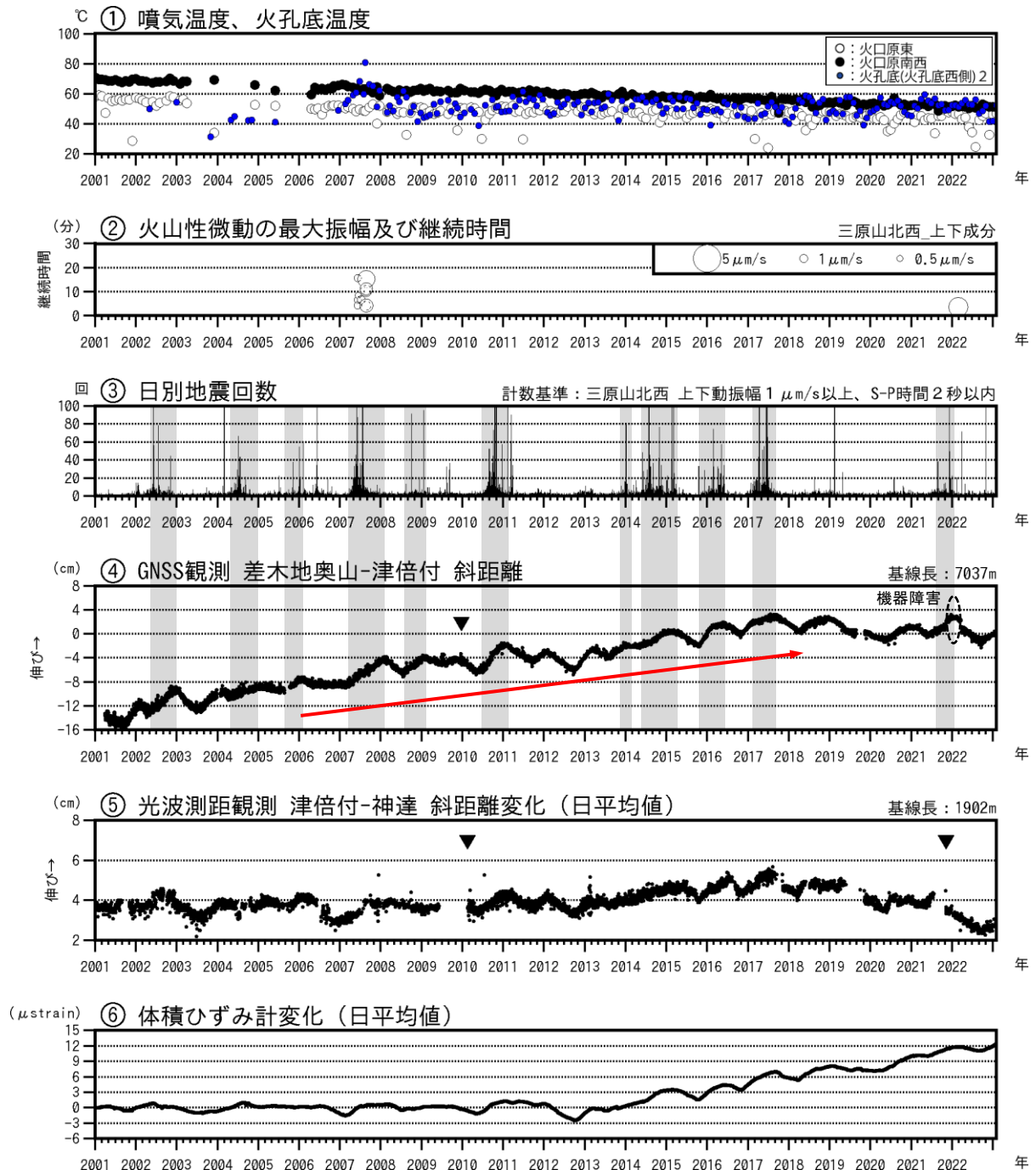
図2 伊豆大島 最近の火山活動経過図（2001年1月～2023年1月31日）
