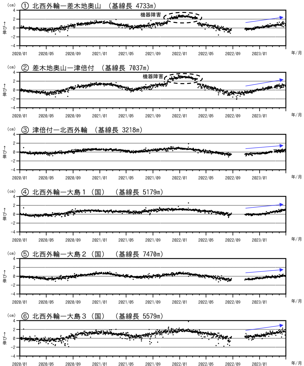
図3-2 伊豆大島 GNSS 連続観測による基線長変化(2020年1月～2023年4月30日)
