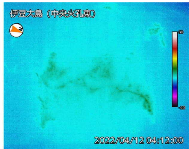
2022年4月12日 中央火孔東監視カメラによる
