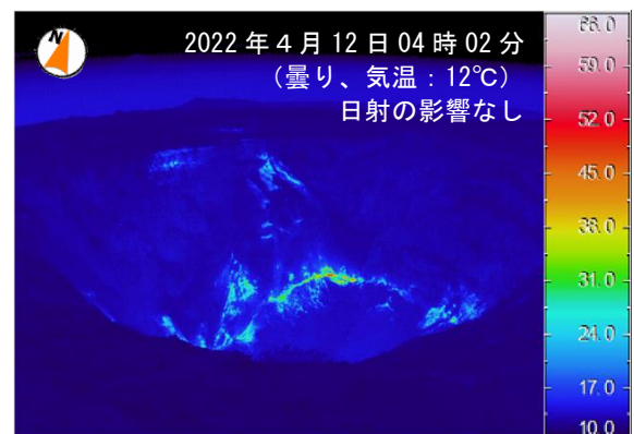
図6 伊豆大島 中央火口内の状況（撮影方向は図8参照）
