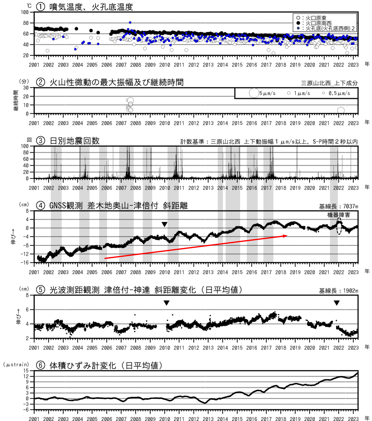
図2 伊豆大島 最近の火山活動経過図（2001年1月～2023年4月30日）
