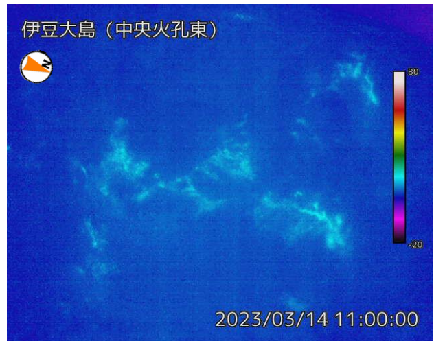
3月14日 中央火孔東監視カメラによる
