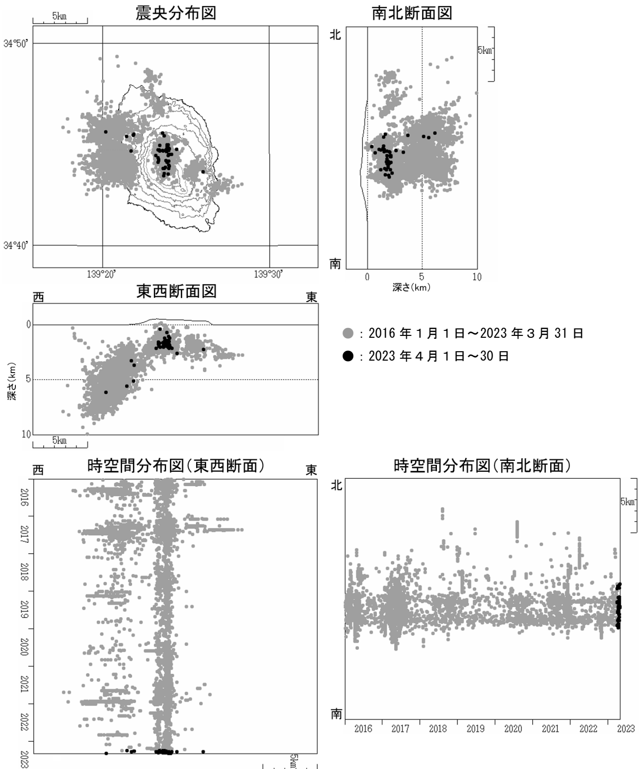
図4 伊豆大島 震源分布図（2016 年 1 月 1 日～2023 年 4 月 30 日）
