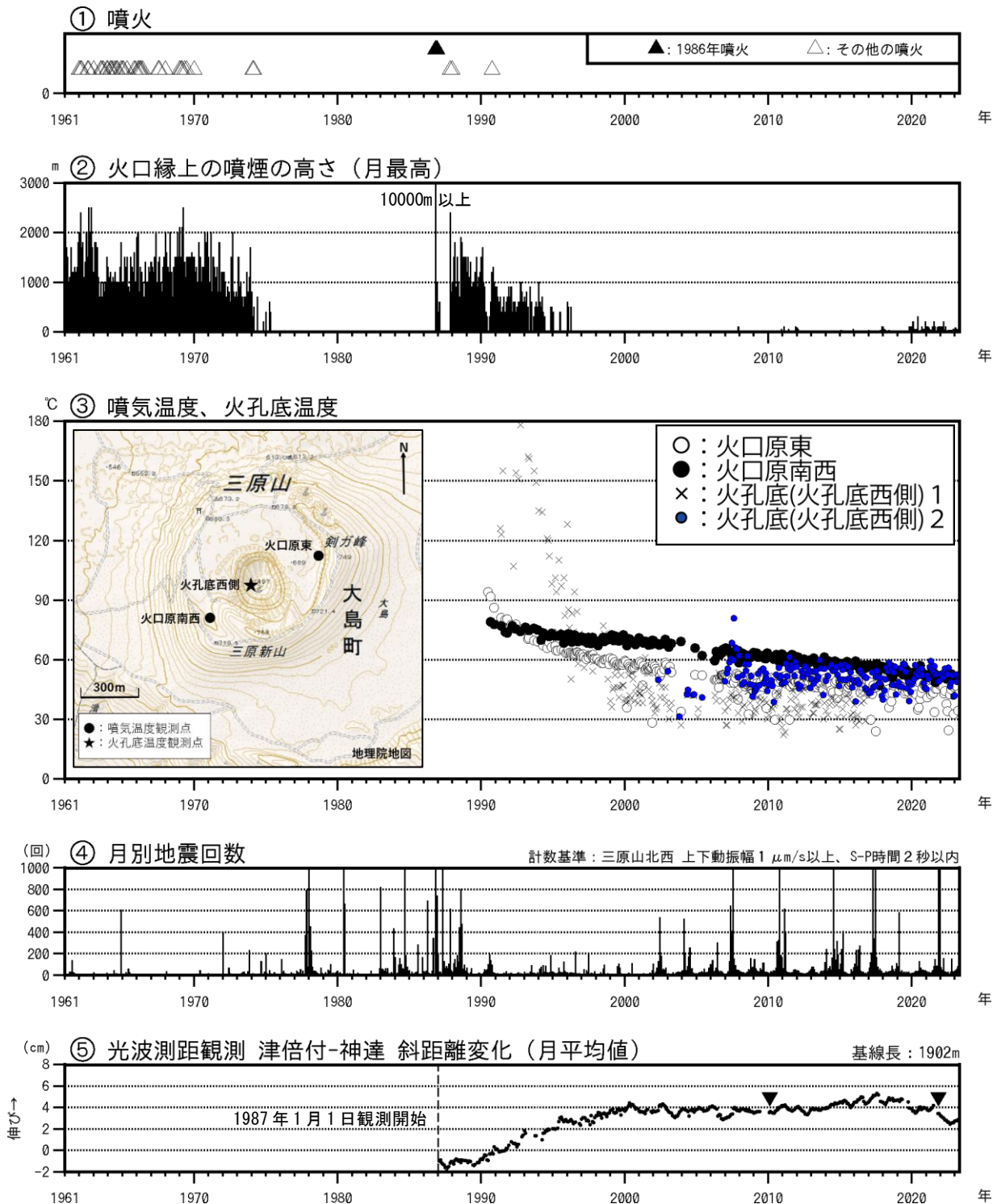
図1 伊豆大島 長期間の火山活動経過図（1961年1月～2023年4月30日）
