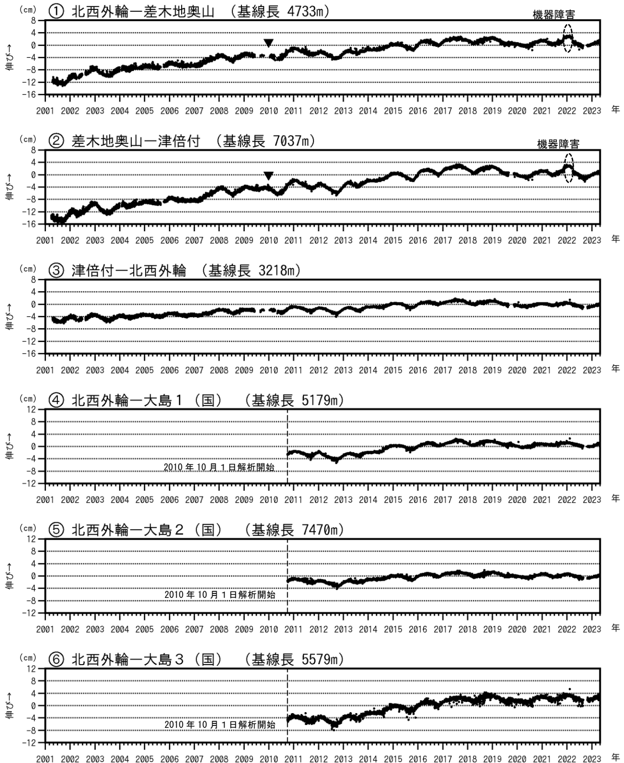
図3-1 伊豆大島 GNSS 連続観測による基線長変化(2001年1月～2023年4月30日)
