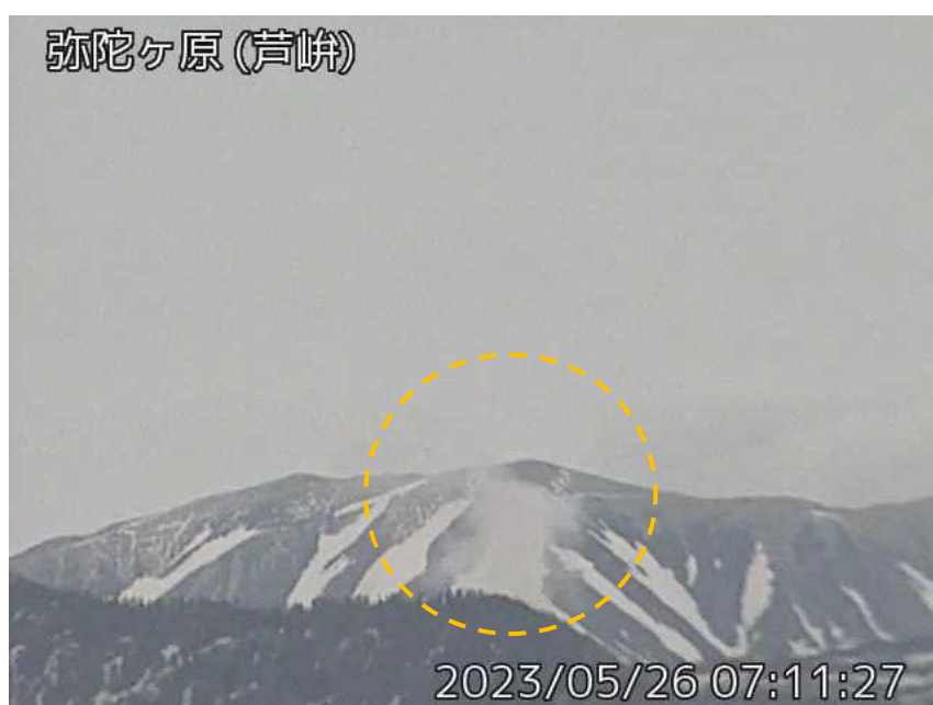
図1 弥陀ヶ原 地獄谷からの噴気の様（橙丸）（5月26日、芦峠監視カメラによる）
