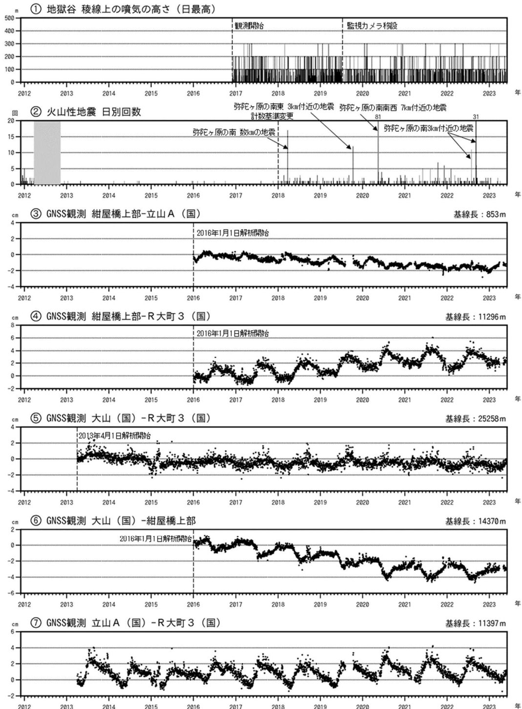
図3 弥陀ヶ原 火山活動経過図（2011年12月1日～2023年5月31日）
