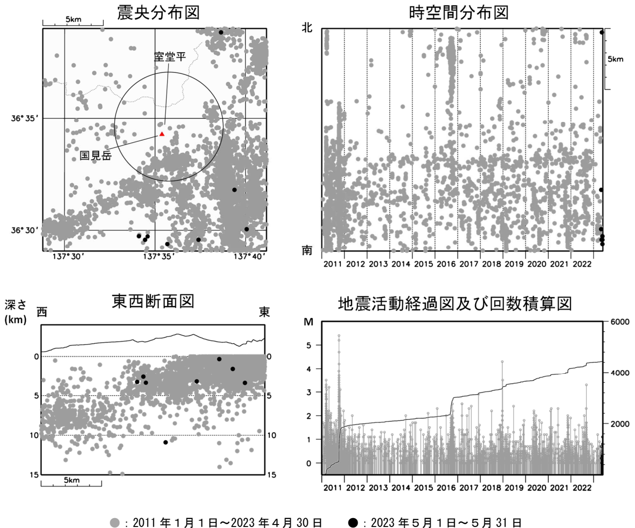
図2 弥陀ヶ原 広域地震観測網による山体・周辺の地震活動（2011年1月1日～2023年5月31日） 震央分布図中の円は弥陀ヶ原の計数対象地震（室堂平でS-P時間1秒以内）のおよその範囲を示しています。 広域地震観測網により震源決定したもので、深さは全て海面以下として決定しています。 図中の震源要素は一部暫定値が含まれており、後日変更することがあります。 この図では、関係機関の地震波形を一元的に処理し、地震観測点の標高を考慮する等した手法で得られた震源を用いています（ただし、2020年8月以前の地震については火山活動評価のための参考震源です）。
