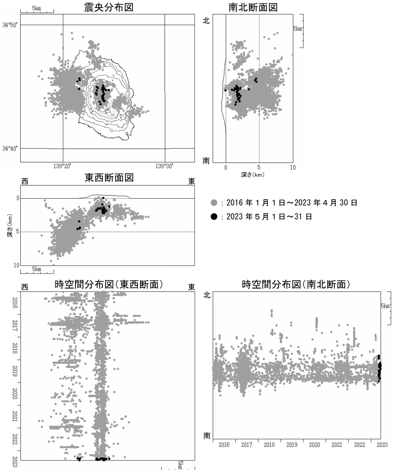
図4 伊豆大島 震源分布図（2016 年 1 月 1 日～2023 年 5 月 31 日）
