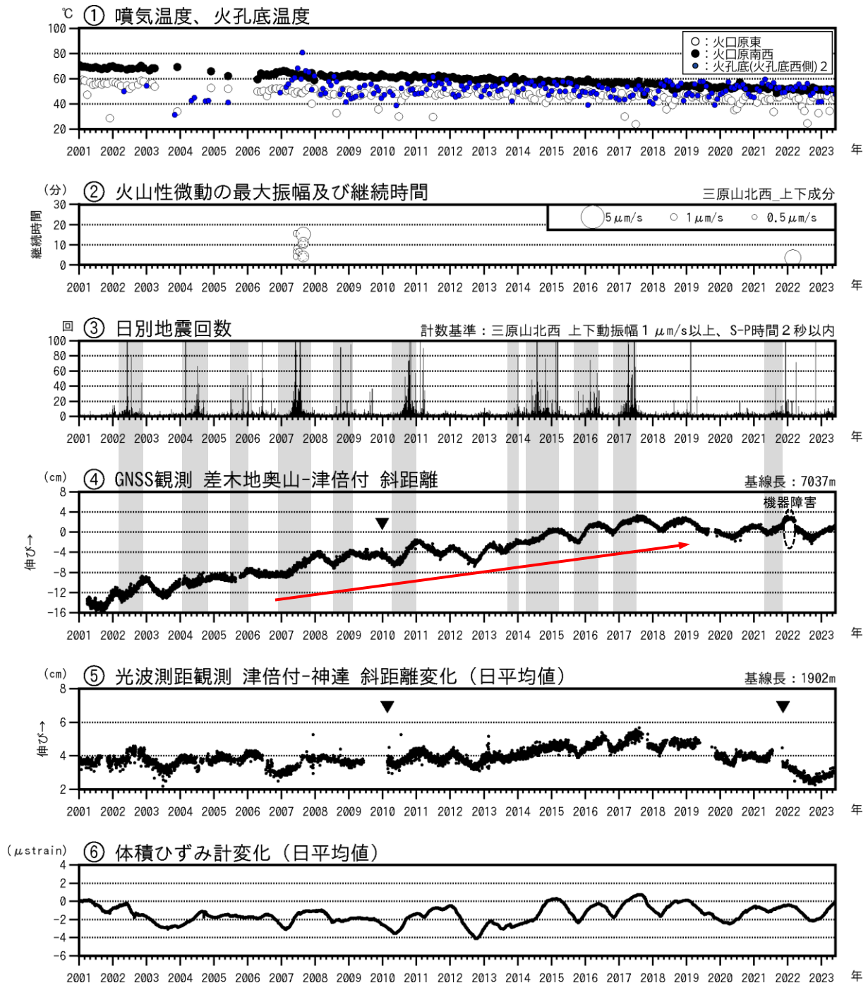
図2 伊豆大島 最近の火山活動経過図（2001年1月～2023年5月31日）
