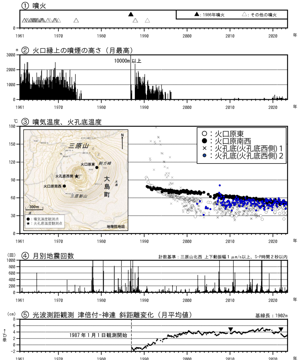
図1 伊豆大島 長期間の火山活動経過図 (1961年1月～2023年5月31日)
