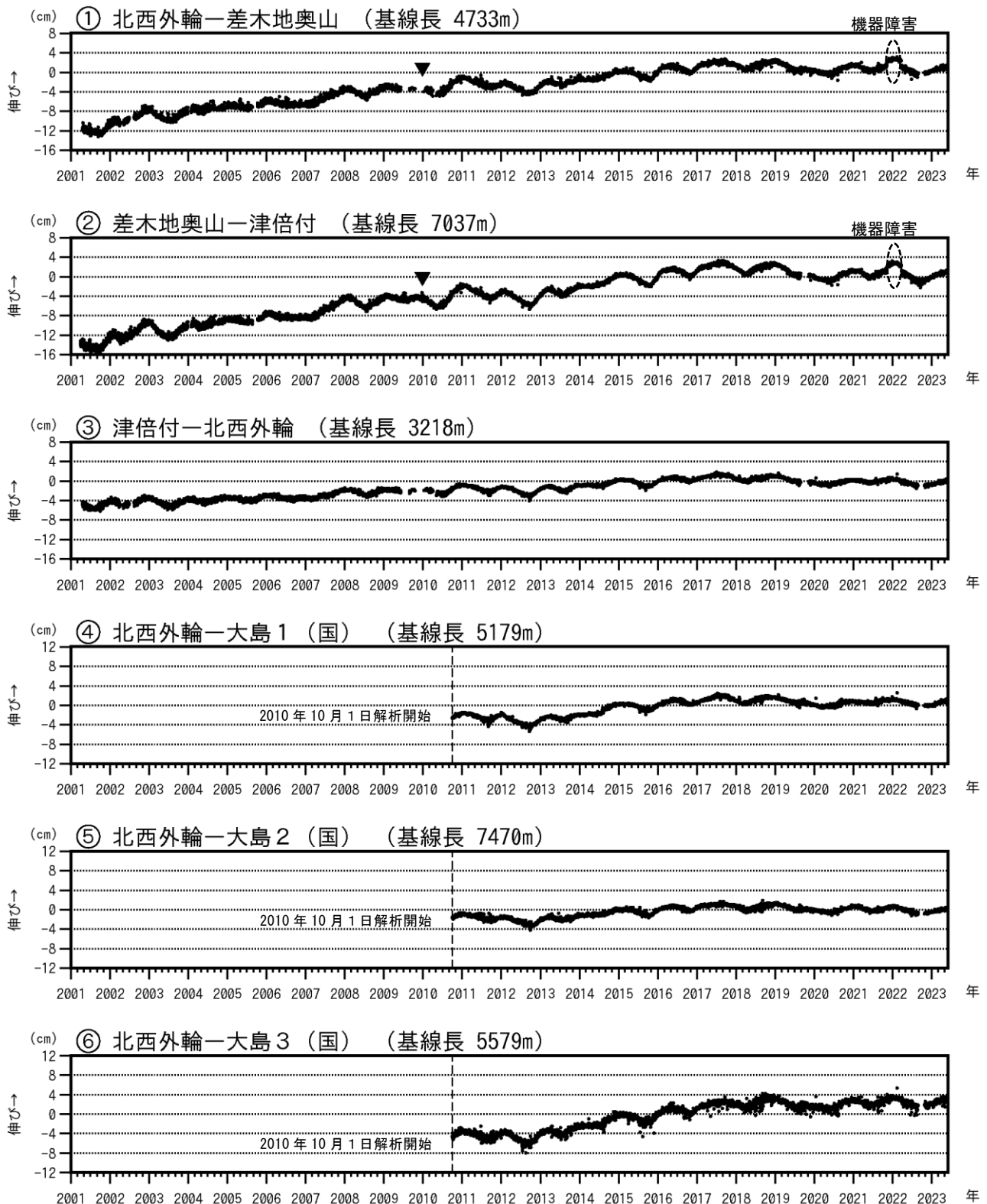
図3-1 伊豆大島 GNSS 連続観測による基線長変化(2001年1月～2023年5月31日)
