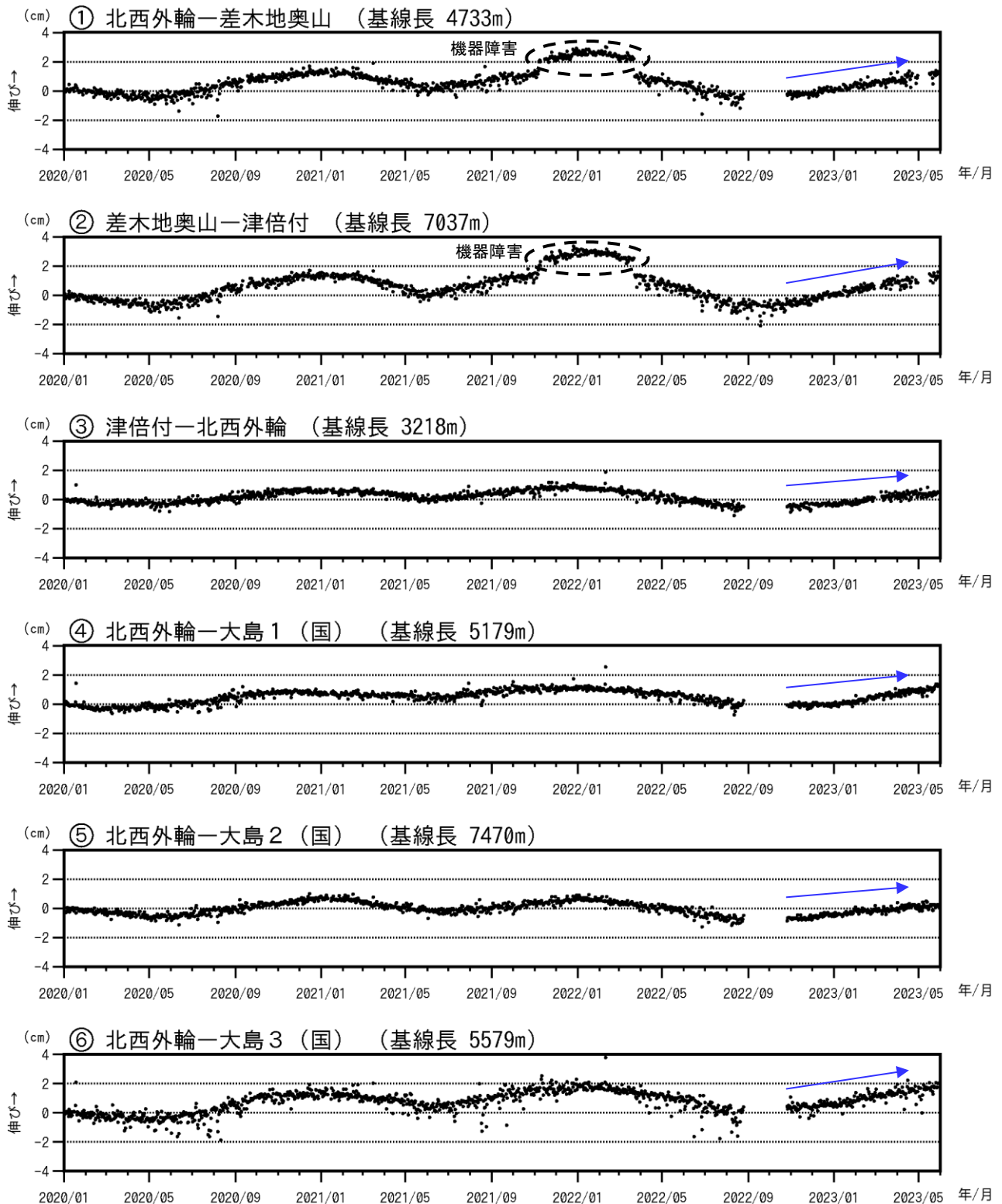
図3-2 伊豆大島 GNSS 連続観測による基線長変化(2020年1月～2023年5月31日)
