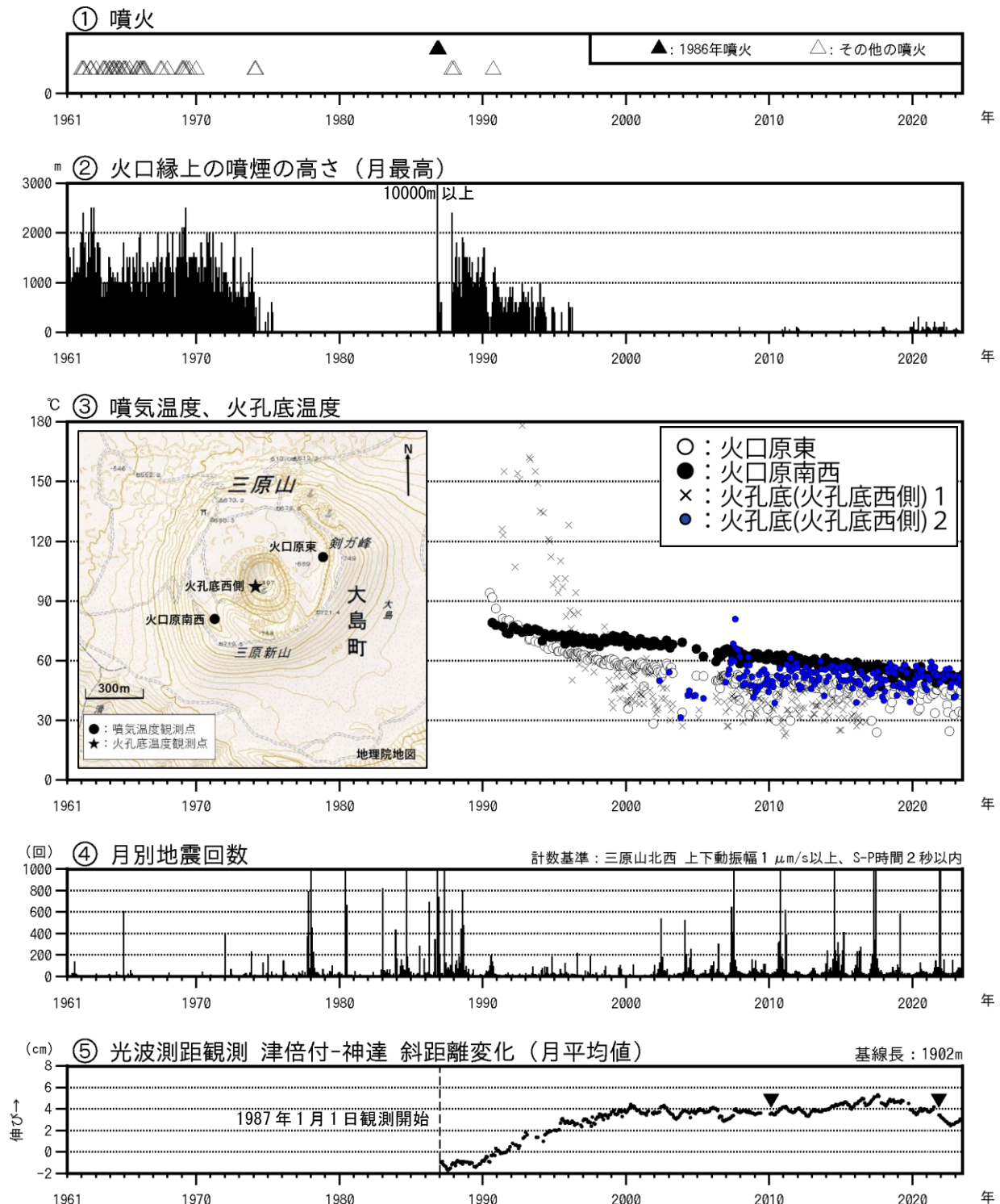
図1 伊豆大島 長期間の火山活動経過図 (1961 年 1 月～2023 年 6 月 30 日)
