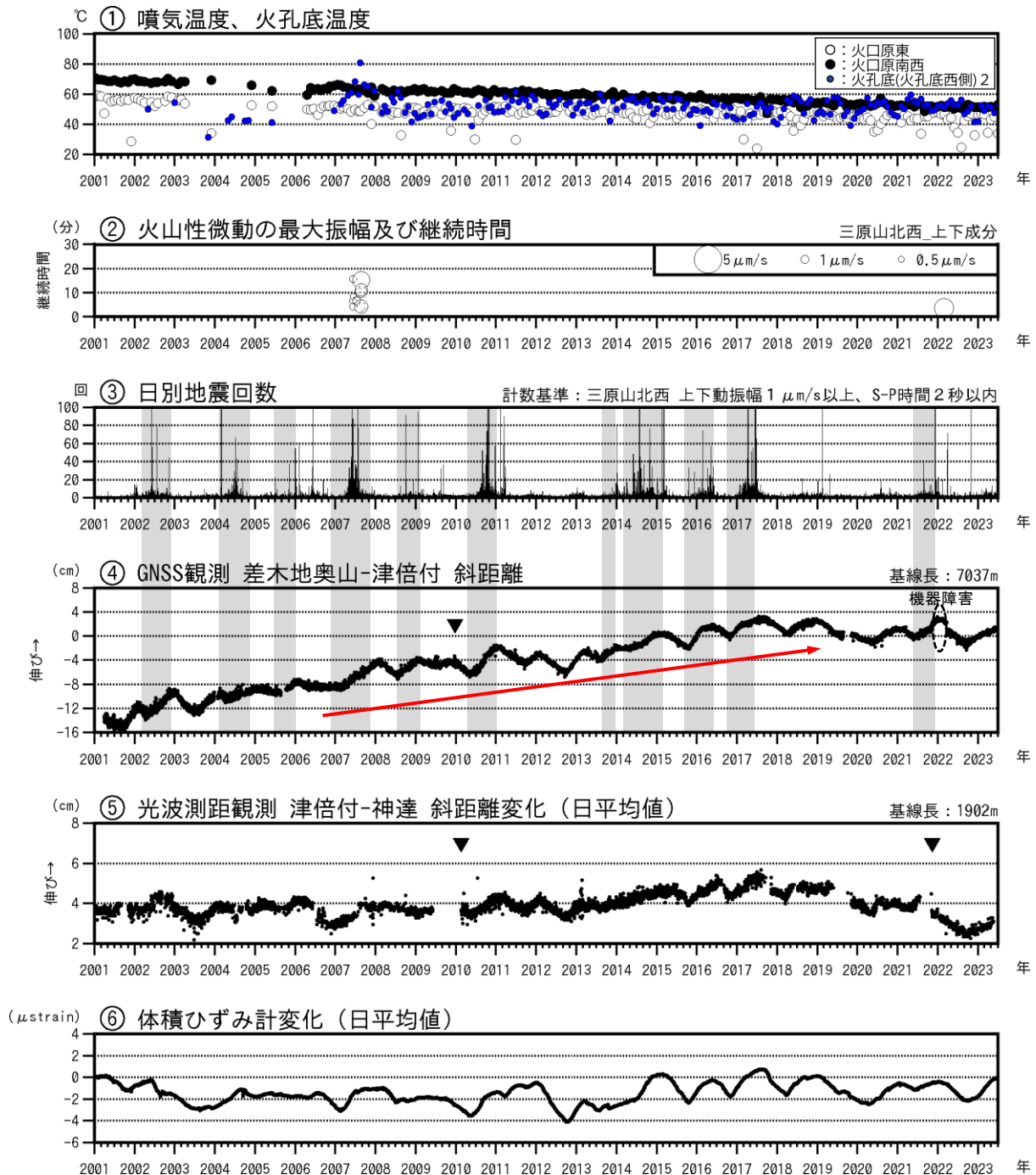
図2 伊豆大島 最近の火山活動経過図（2001年1月～2023年6月30日）
