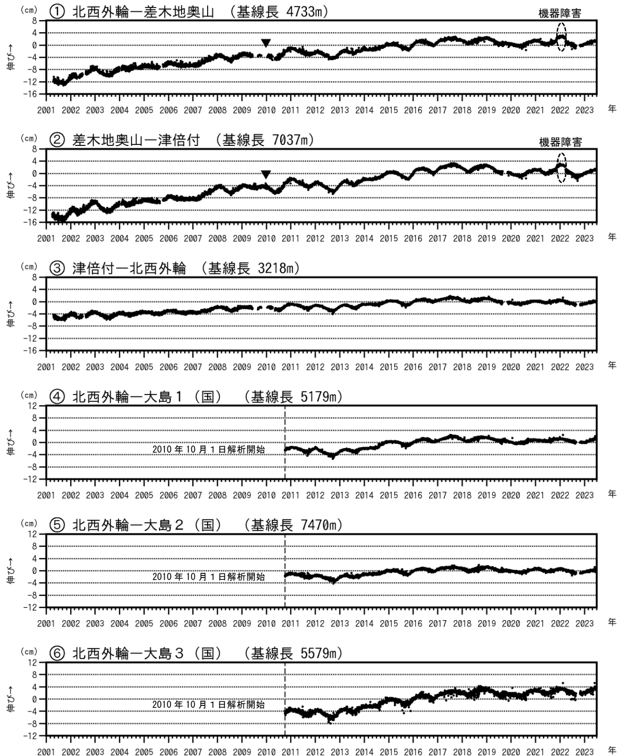
図3-1 伊豆大島 GNSS 連続観測による基線長変化(2001年1月～2023年6月30日)
