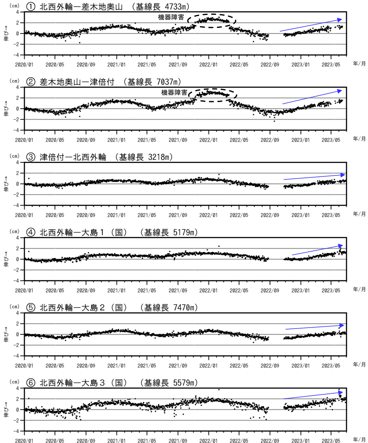
図3-2 伊豆大島 GNSS 連続観測による基線長変化(2020年1月～2023年6月30日)
