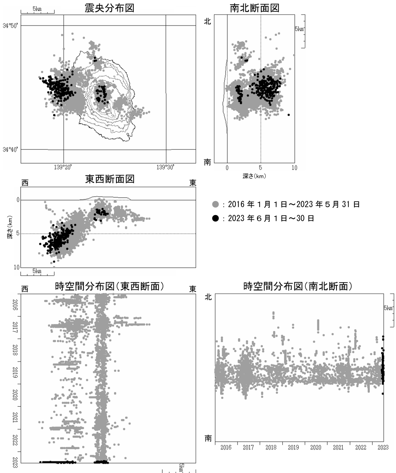
図4 伊豆大島 震源分布図（2016 年 1 月 1 日～2023 年 6 月 30 日）
