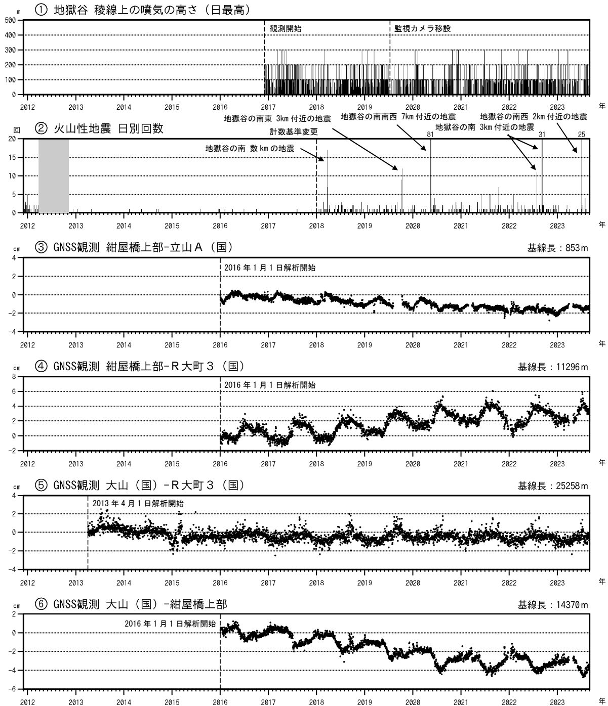
図3 弥陀ヶ原 火山活動経過図（2011年12月1日～2023年8月31日）
