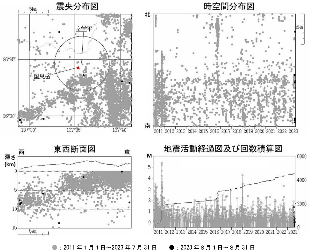
図2 弥陀ヶ原 広域地震観測網による山体・周辺の地震活動（2011 年 1 月 1 日～2023 年 8 月 31 日） 震央分布図中の円は弥陀ヶ原の計数対象地震（室堂平で S-P 時間 1 秒以内）のおよその範囲を示しています。 広域地震観測網により震源決定したもので、深さは全て海面以下として決定しています。 図中の震源要素は一部暫定値が含まれており、後日変更することがあります。 この図では、関係機関の地震波形を一元的に処理し、地震観測点の標高を考慮する等した手法で得られた震源を用いています（ただし、2020 年 8 月以前の地震については火山活動評価のための参考震源です）。
