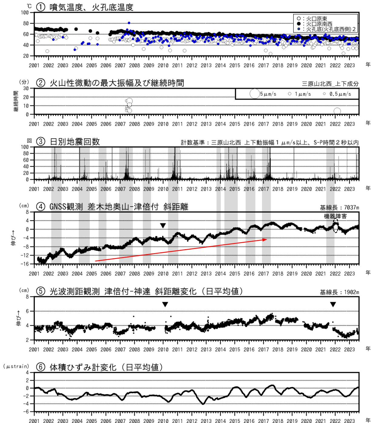
図2 伊豆大島 最近の火山活動経過図（2001年1月～2023年8月31日）
