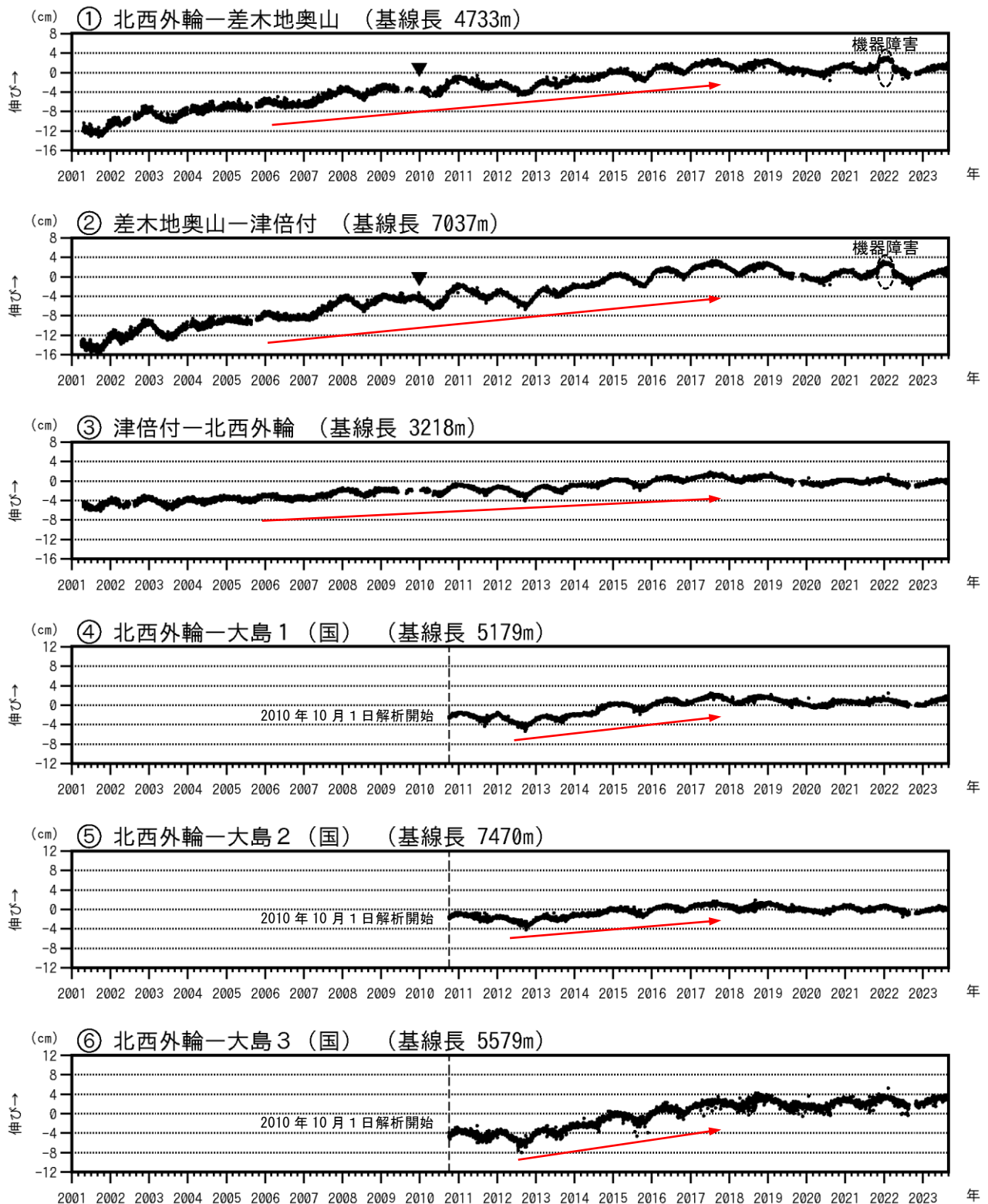
図3-1 伊豆大島 GNSS 連続観測による基線長変化(2001年1月～2023年8月31日)
