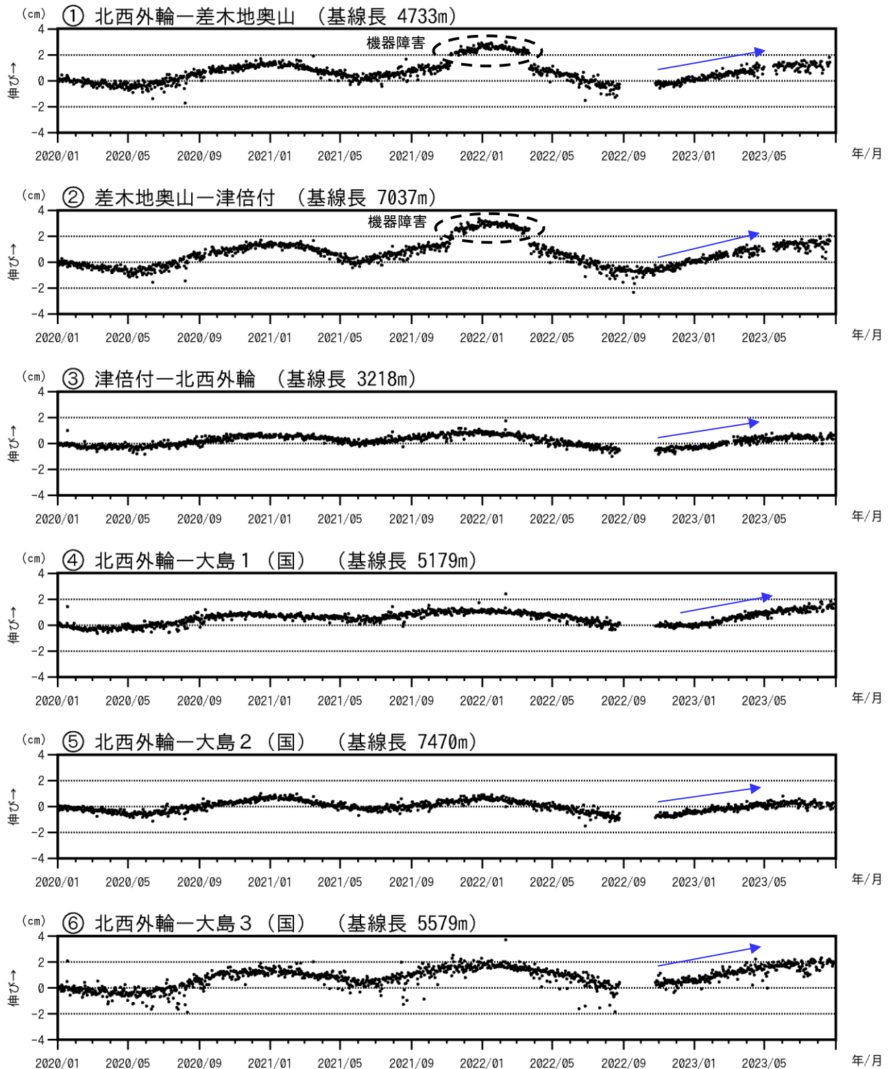
図3-2 伊豆大島 GNSS 連続観測による基線長変化(2020年1月～2023年8月31日)
