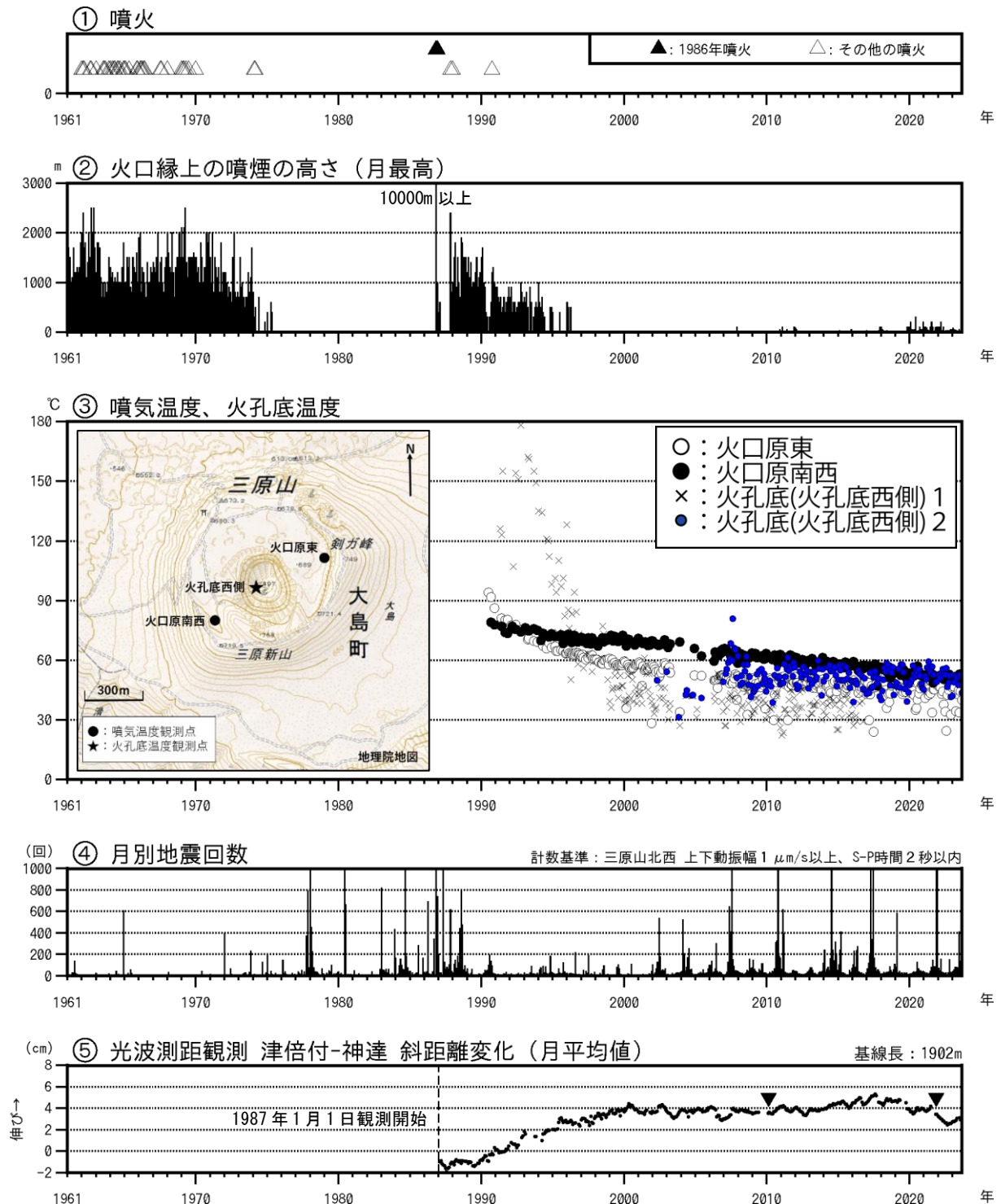
図1 伊豆大島 長期間の火山活動経過図（1961年1月～2023年8月31日）
