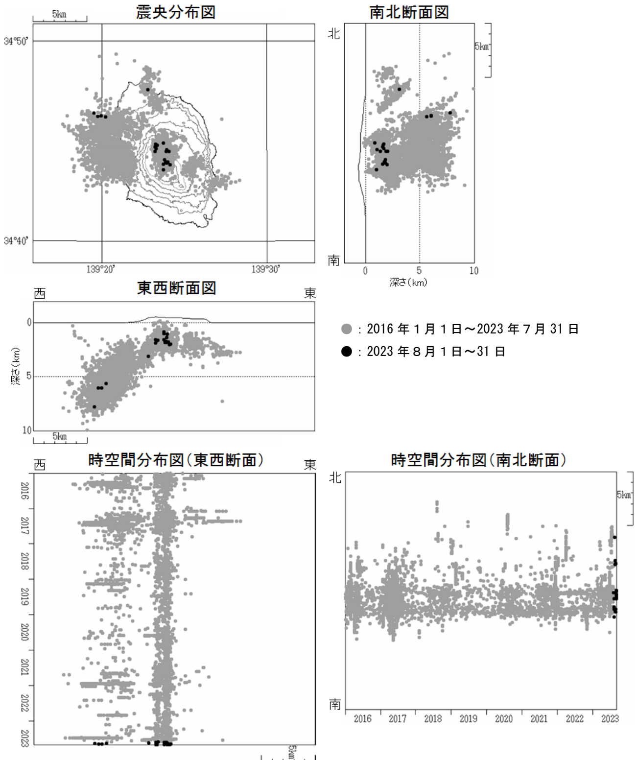
図4 伊豆大島 震源分布図（2016 年 1 月 1 日～2023 年 8 月 31 日）
