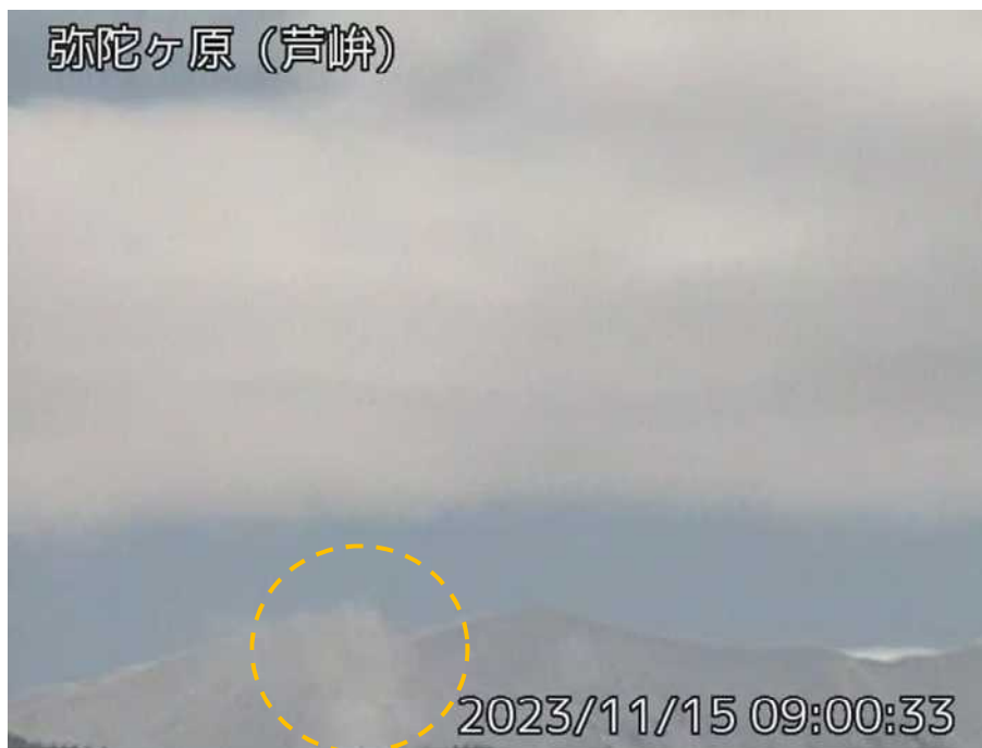
図1 弥陀ヶ原 地獄谷からの噴気の状況（橙丸）（11月15日、芦峠監視カメラによる）
