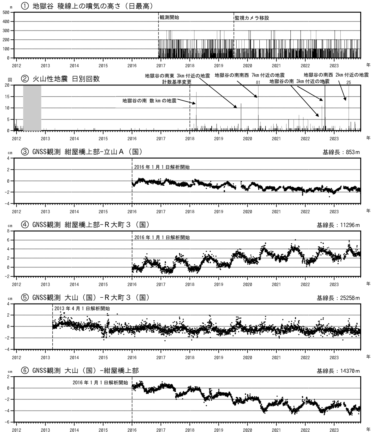
図 3 弥陀ヶ原 火山活動経過図（2011 年 12 月 1 日～2023 年 11 月 30 日）
