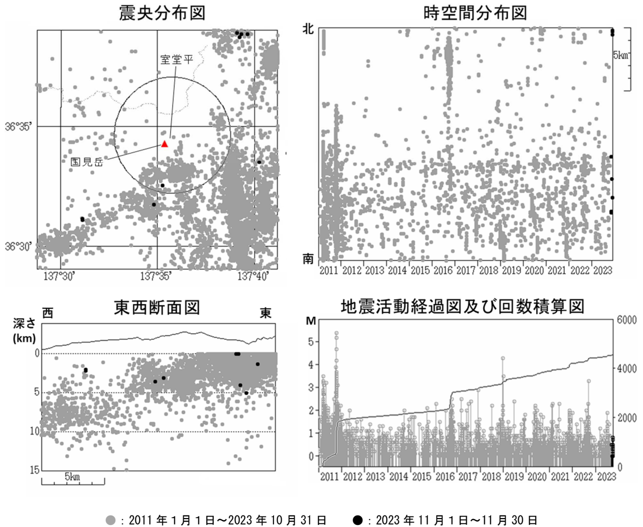
図2 弥陀ヶ原 広域地震観測網による山体・周辺の地震活動（2011 年 1 月 1 日～2023 年 11 月 30 日） 震央分布図中の円は弥陀ヶ原の計数対象地震（室堂平で S-P 時間 1 秒以内）のおよその範囲を示しています。 広域地震観測網により震源決定したもので、深さは全て海面以下として決定しています。 図中の震源要素は一部暫定値が含まれており、後日変更することがあります。 この図では、関係機関の地震波形を一元的に処理し、地震観測点の標高を考慮する等した手法で得られた震源を用いています（ただし、2020 年 8 月以前の地震については火山活動評価のための参考震源です）。
