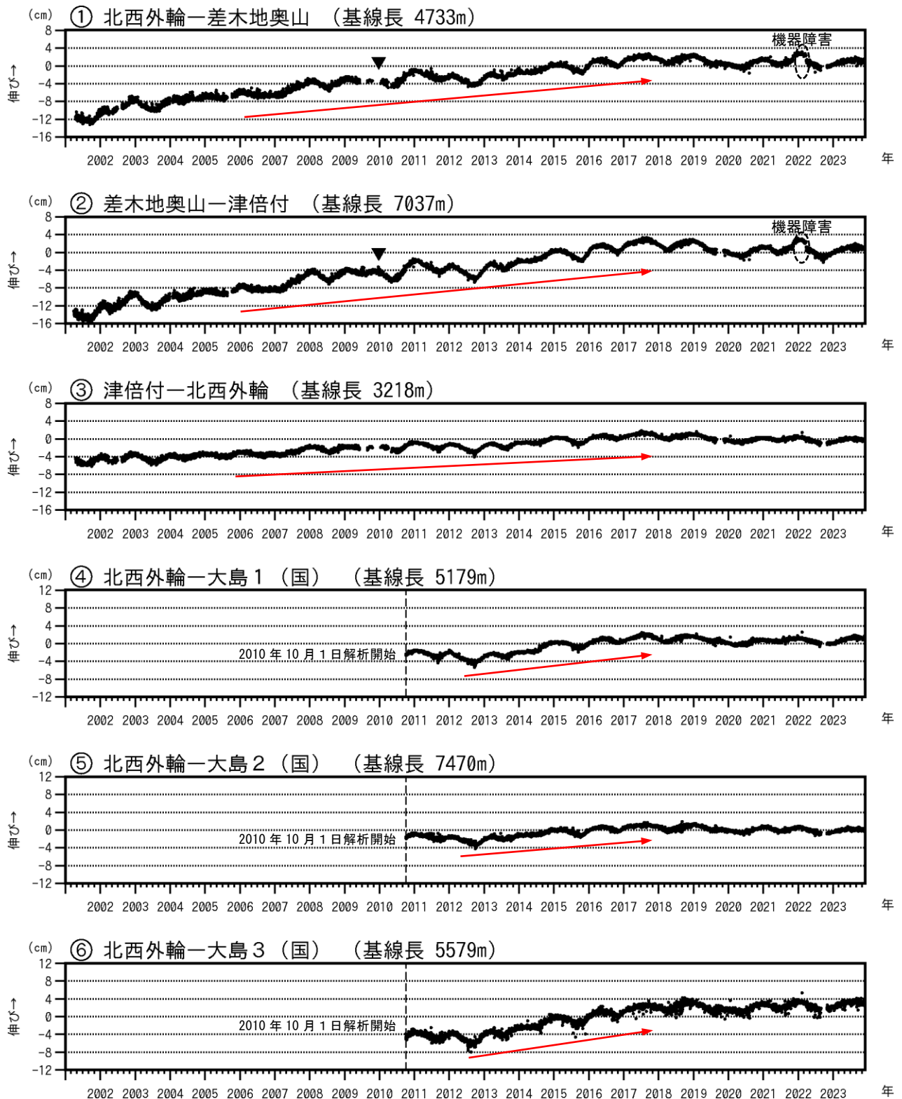
図3-1 伊豆大島 GNSS 連続観測による基線長変化(2001年1月～2023年11月30日)
