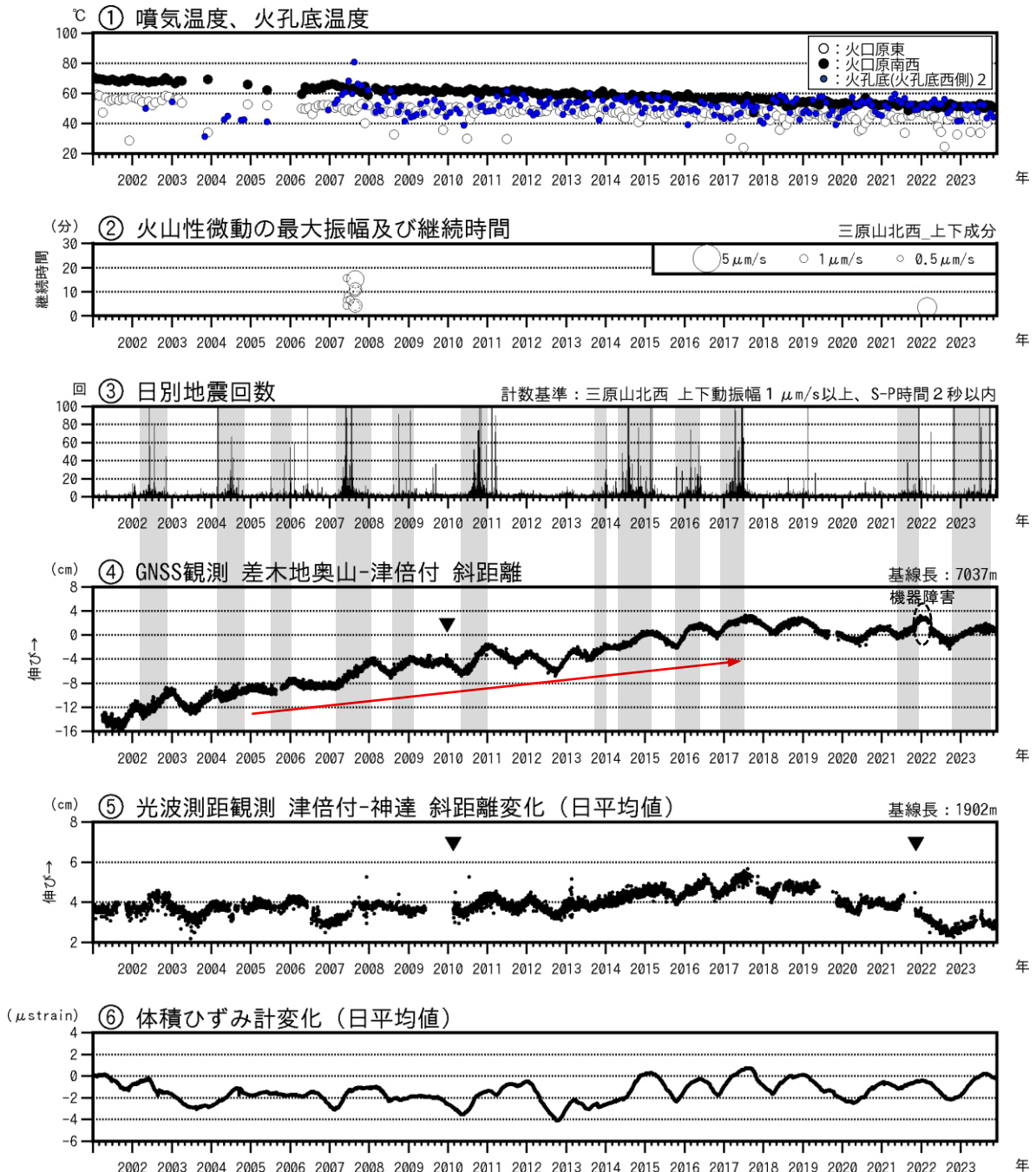
図2 伊豆大島 最近の火山活動経過図（2001年1月～2023年11月30日）
