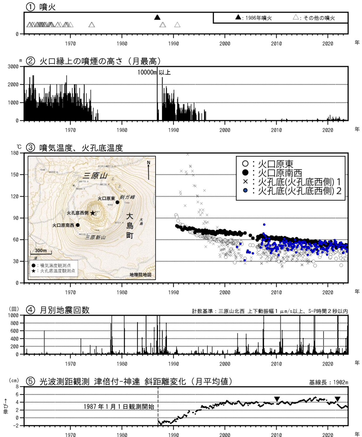
図1 伊豆大島 長期間の火山活動経過図（1961年1月～2023年11月30日）
