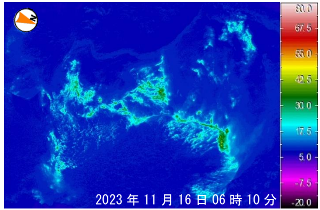
中央火孔東カメラ位置からの熱画像 (11月16日 現地調査時に撮影)
