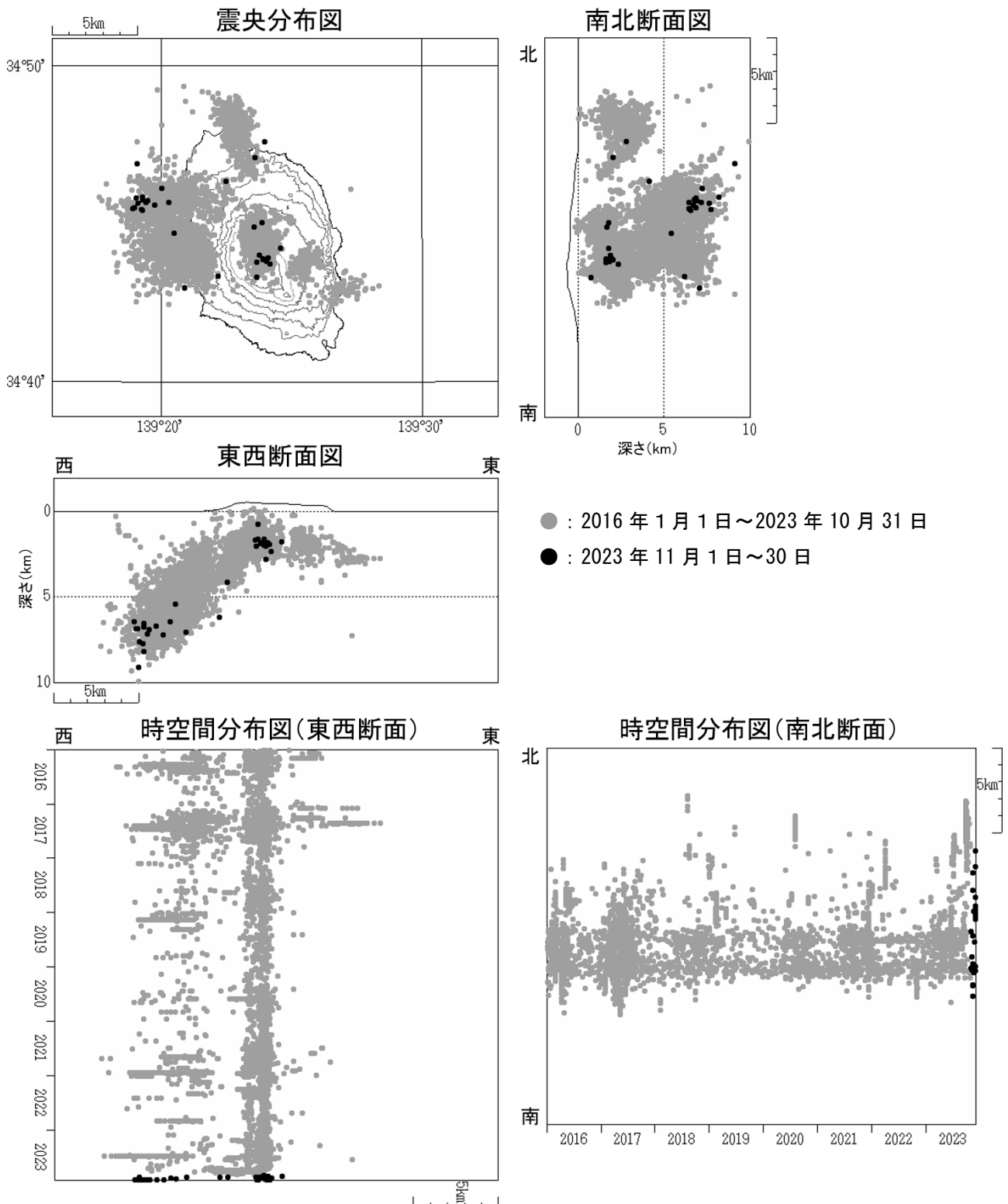
図4 伊豆大島 震源分布図（2016 年 1 月 1 日～2023 年 11 月 30 日）
