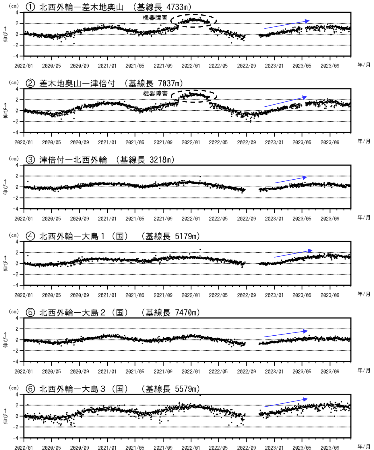
図3-2 伊豆大島 GNSS 連続観測による基線長変化(2020年1月～2023年11月30日)
