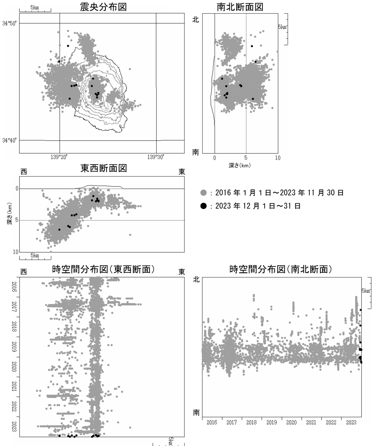
図4 伊豆大島 震源分布図（2016 年 1 月 1 日～2023 年 12 月 31 日）
