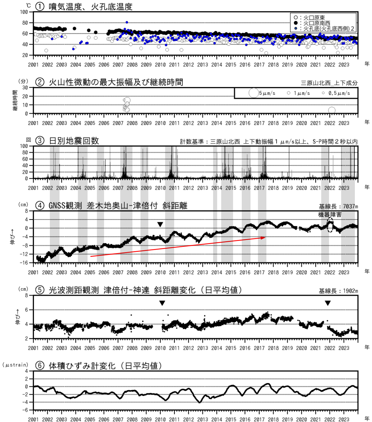
図2 伊豆大島 最近の火山活動経過図（2001年1月～2023年12月31日）
