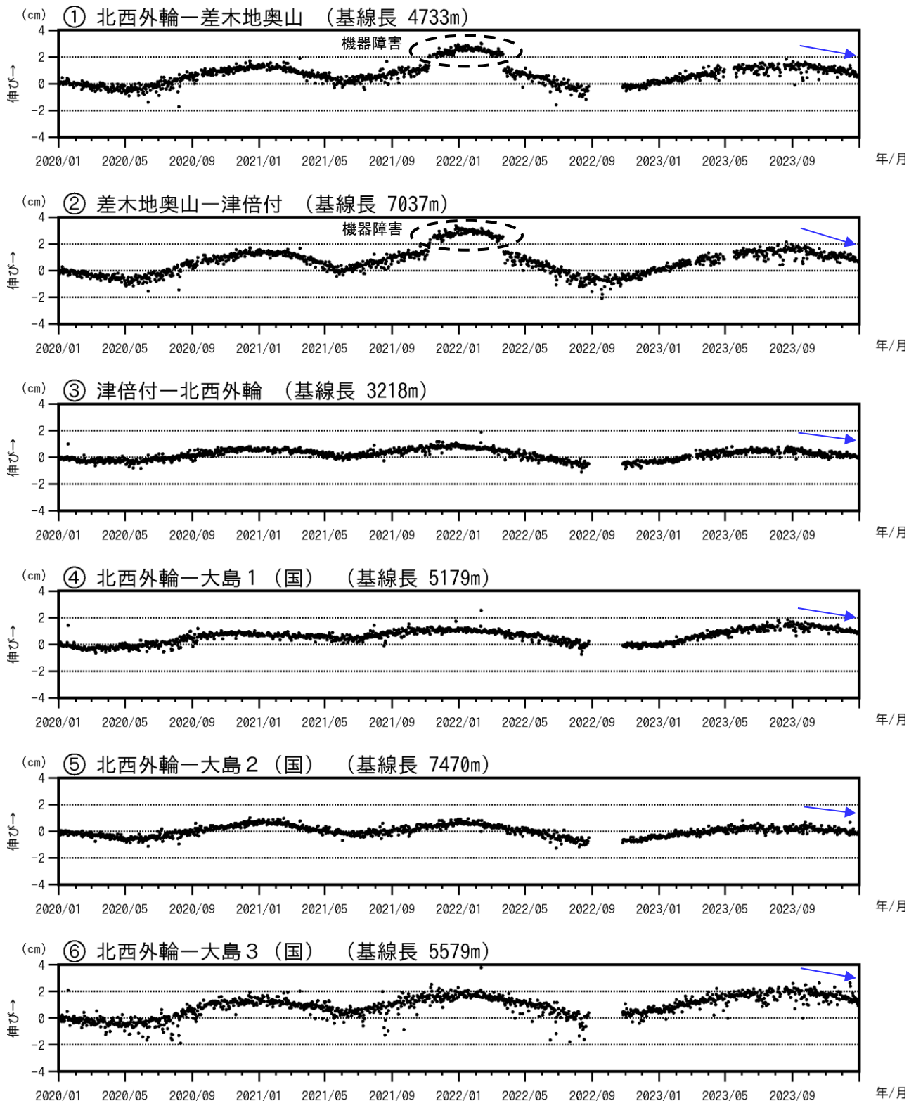
図 3-2 伊豆大島 GNSS 連続観測による基線長変化(2020 年 1 月～2023 年 12 月 31 日)
