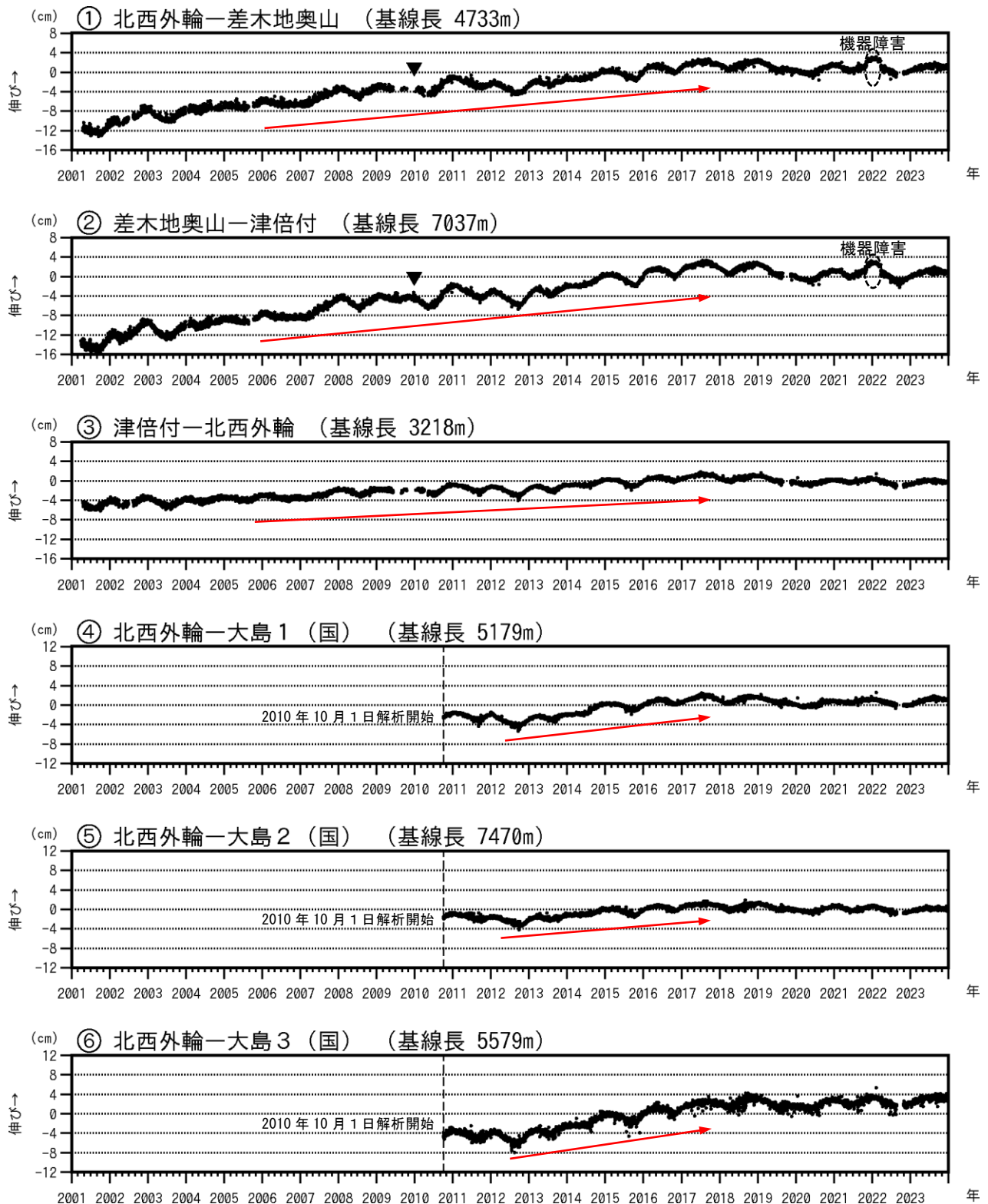
図3-1 伊豆大島 GNSS 連続観測による基線長変化(2001年1月～2023年12月31日)
