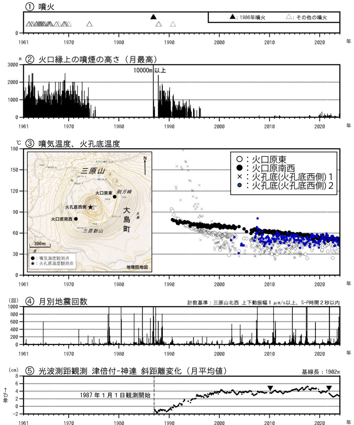
図1 伊豆大島 長期間の火山活動経過図（1961年1月～2023年12月31日）
