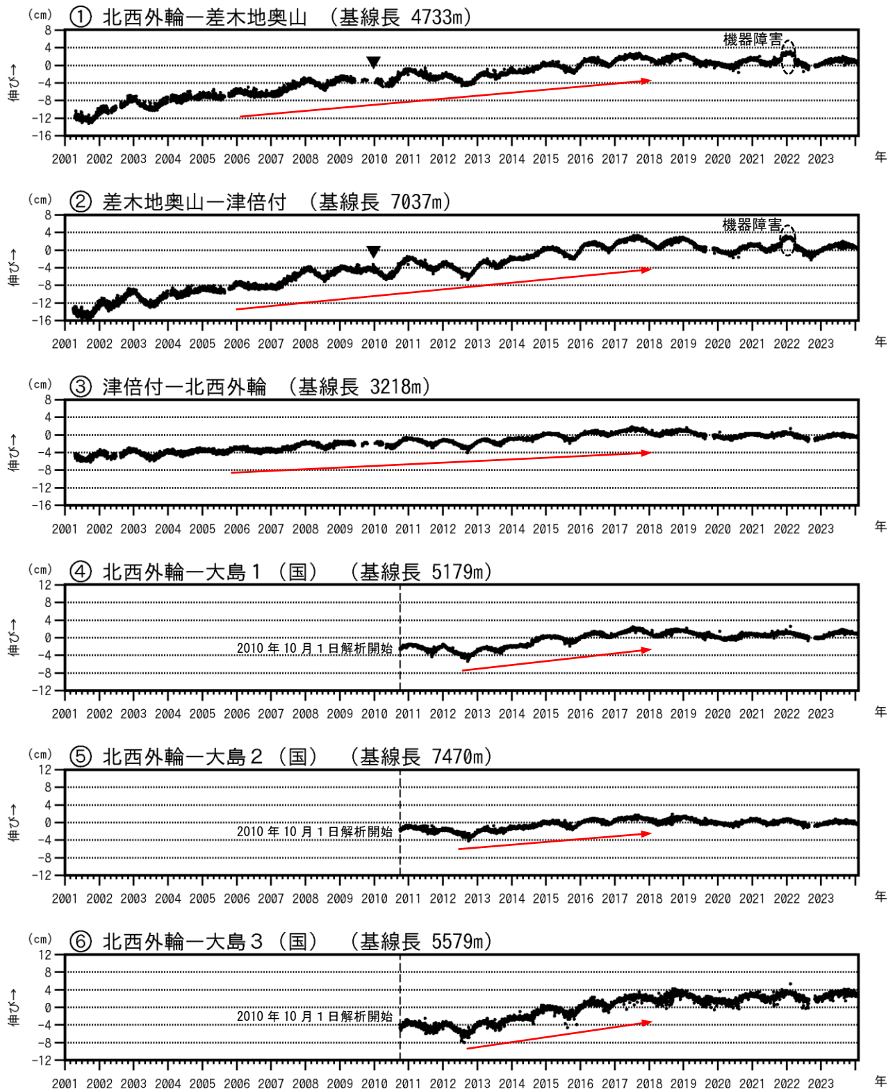
図3-1 伊豆大島 GNSS 連続観測による基線長変化(2001年1月～2024年1月31日)
