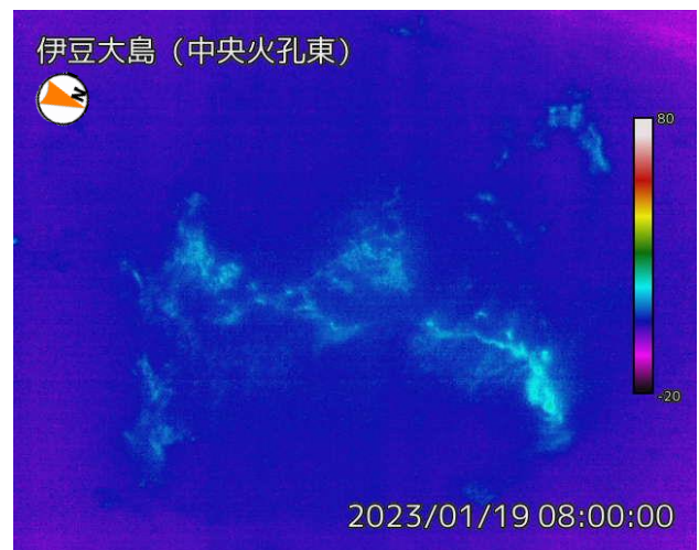
2023年1月19日 中央火孔東監視カメラによる
