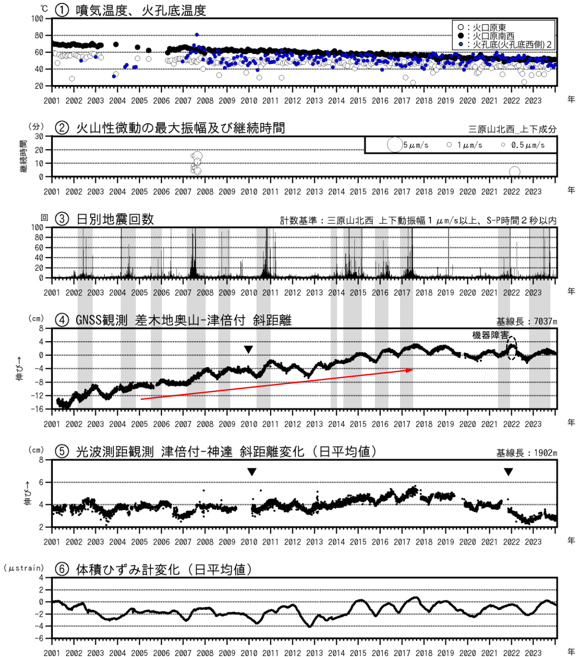
図2 伊豆大島 最近の火山活動経過図（2001年1月～2024年1月31日）
