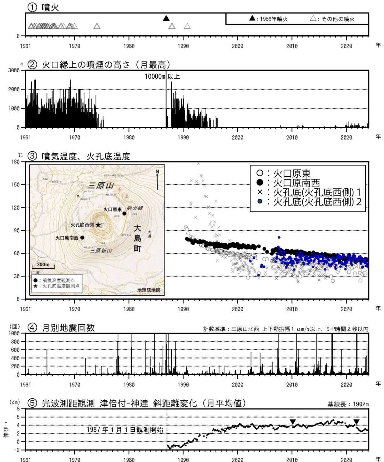
図1 伊豆大島 長期間の火山活動経過図（1961年1月～2024年1月31日）
