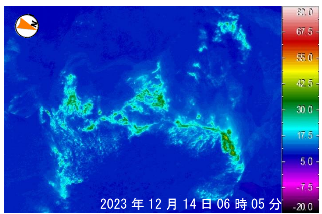
中央火孔東カメラ位置からの熱画像 (2023年12月14日 現地調査時に撮影)
