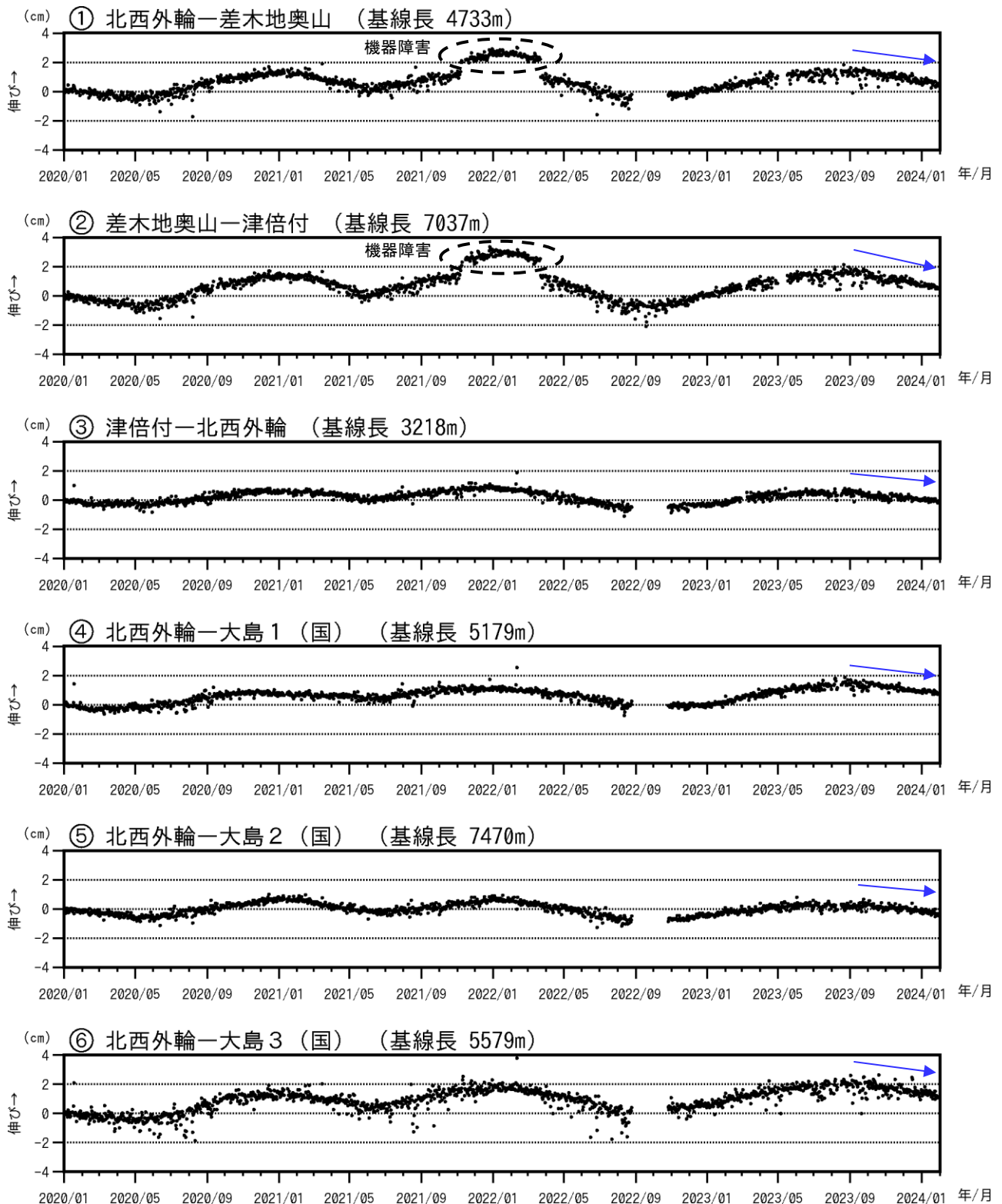
図3-2 伊豆大島 GNSS 連続観測による基線長変化(2020年1月～2024年1月31日)
