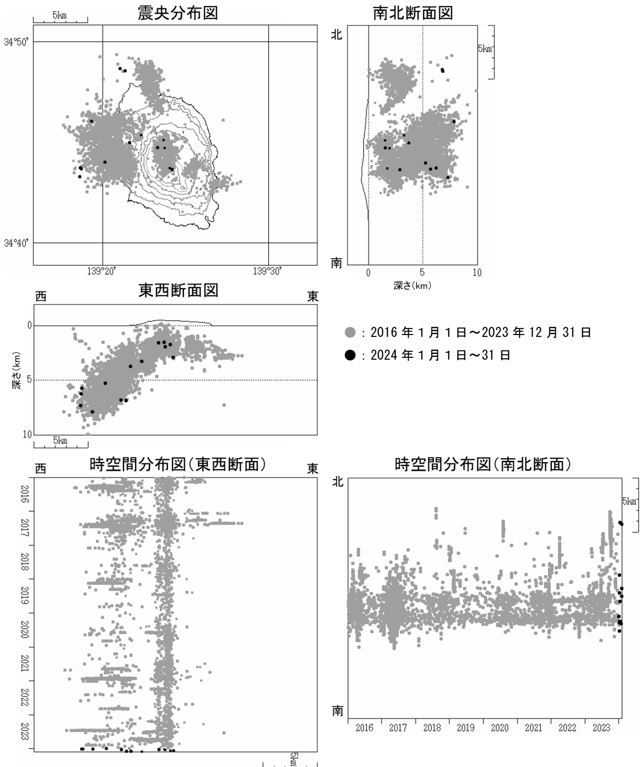
図4 伊豆大島 震源分布図（2016 年 1 月 1 日～2024 年 1 月 31 日）
