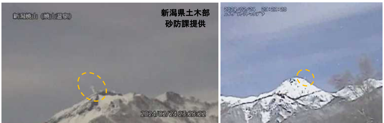
図1 新潟焼山 山頂部の噴煙（橙色粋）の状況 （左：焼山温泉監視カメラ（2月24日）、右：宇棚監視カメラ（2月24日）による）
