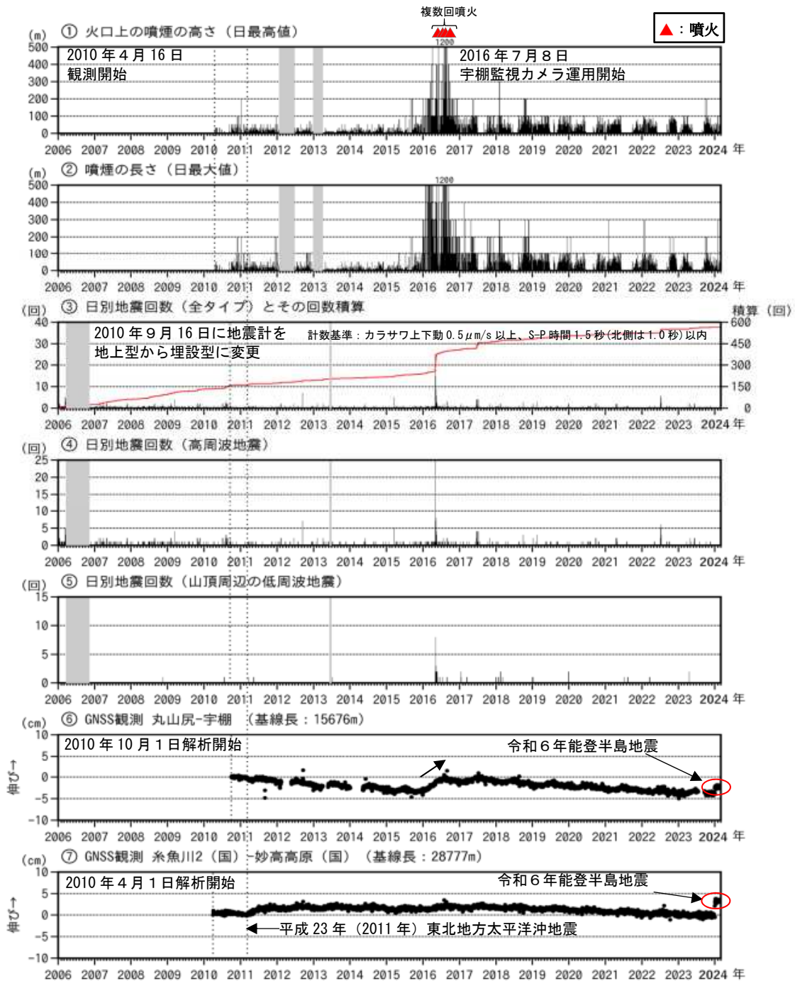
図2 新潟焼山 火山活動経過図（2006年1月1日～2024年2月29日）
