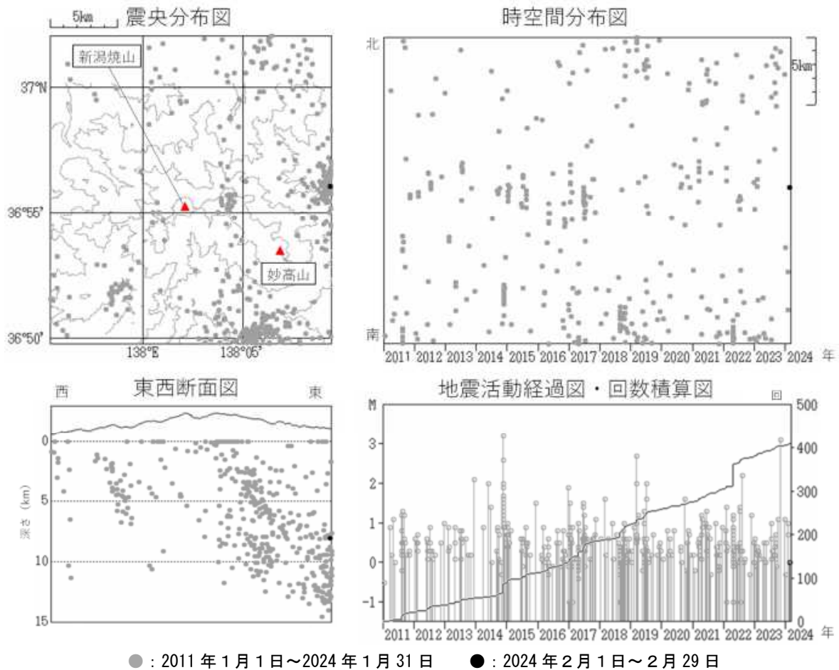
図4 新潟焼山 広域地震観測網による山体・周辺の地震活動（2011 年 1 月 1 日～2024 年 2 月 29 日）
