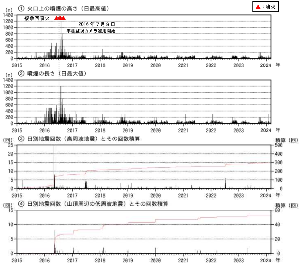
図3 新潟焼山 火山活動経過図（短期）（2015年1月1日～2024年2月29日）
