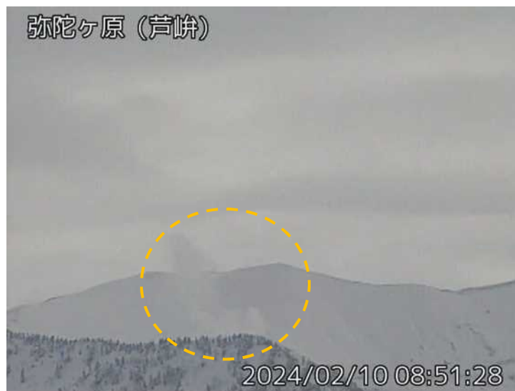
図1 弥陀ヶ原 地獄谷からの噴気の状況（橙丸）（2月10日、芦峠監視カメラによる）
