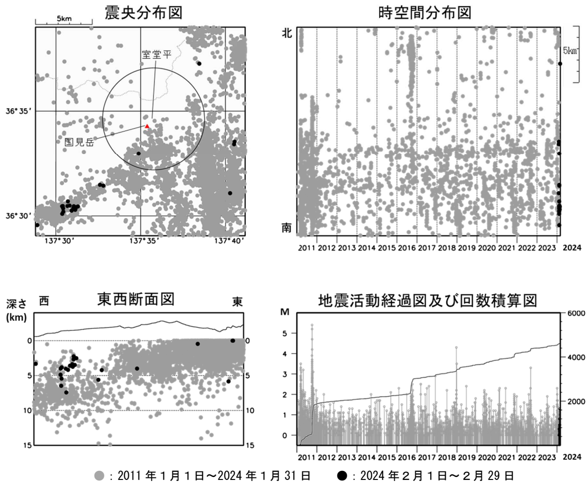
図2 弥陀ヶ原 広域地震観測網による山体・周辺の地震活動（2011 年 1 月 1 日～2024 年 2 月 29 日） 震央分布図中の円は弥陀ヶ原の計数対象地震（室堂平で S-P 時間 1 秒以内）のおよその範囲を示しています。 広域地震観測網により震源決定したもので、深さは全て海面以下として決定しています。 図中の震源要素は一部暫定値が含まれており、後日変更することがあります。 この図では、関係機関の地震波形を一元的に処理し、地震観測点の標高を考慮する等した手法で得られた震源を用いています（ただし、2020 年 8 月以前の地震については火山活動評価のための参考震源です）。
