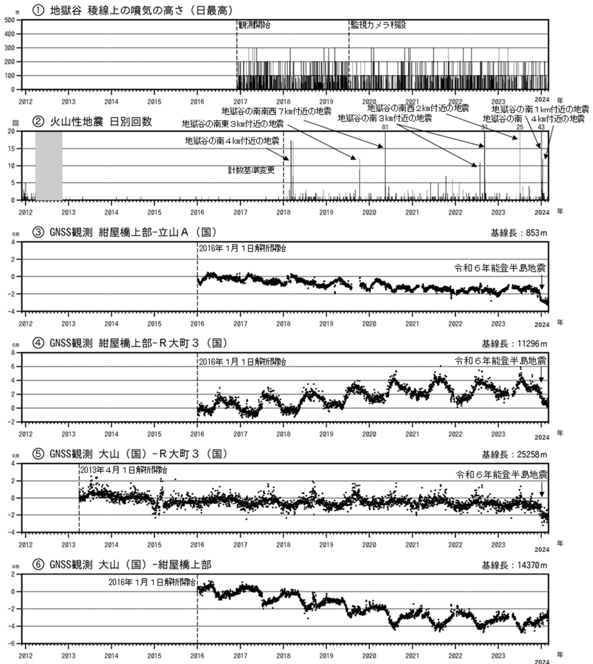
図3 弥陀ヶ原 火山活動経過図（2011年12月1日～2024年2月29日）
