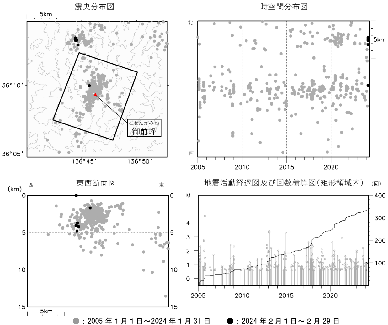
図4 白山 広域地震観測網による山体・周辺の地震活動（2005年1月1日～2024年2月29日）
