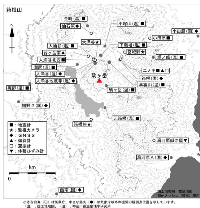
図 6 箱根山 観測点配置図 小さな白丸（○）は気象庁、小さな黒丸（●）は気象庁以外の観測点を示しています。 （国）：国土地理院、 （温）：神奈川県温泉地学研究所
