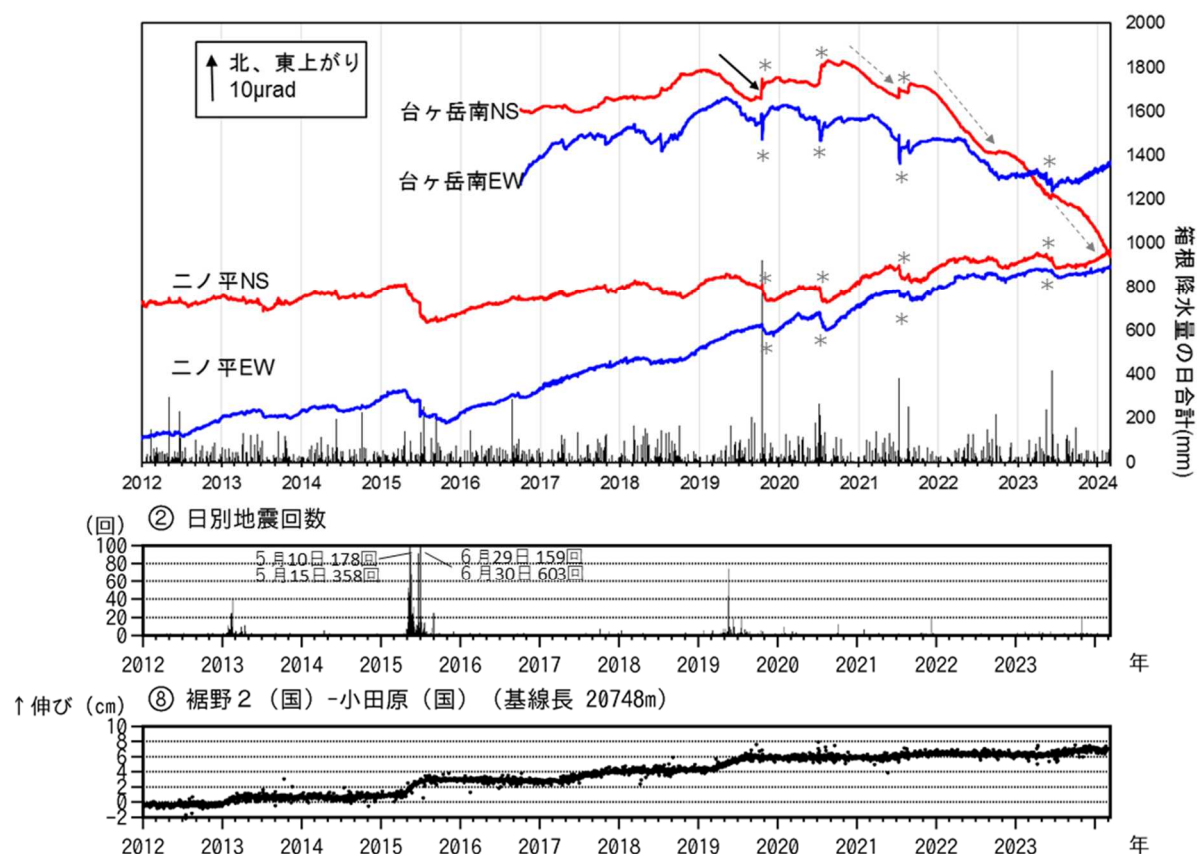
図5 箱根山 傾斜観測及び地震回数・GNSS観測（2012年1月1日～2024年2月29日） *印は降水による影響と考えられる変動を示します。（国）：国土地理院 ⑧は図3-2基線⑧に対応します。
