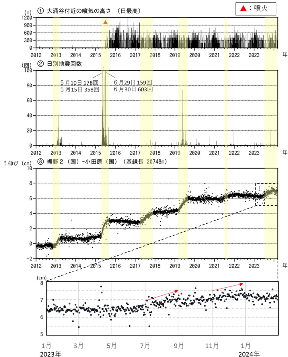
図3-1 箱根山 火山活動経過図（2012年1月1日～2024年2月29日）
