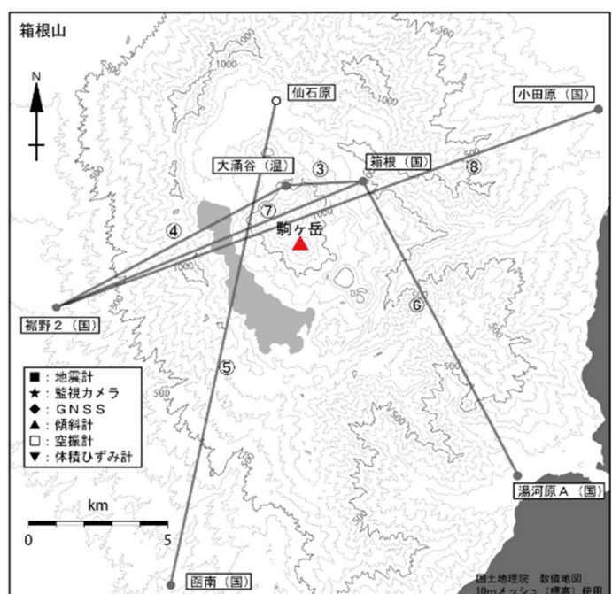
図3-2 箱根山 GNSS 連続観測による基線長変化及び観測点配置図 (2012年1月1日～2024年2月29日) (国)：国土地理院 (温)：神奈川県温泉地学研究所 空白部分は欠測を示します。
