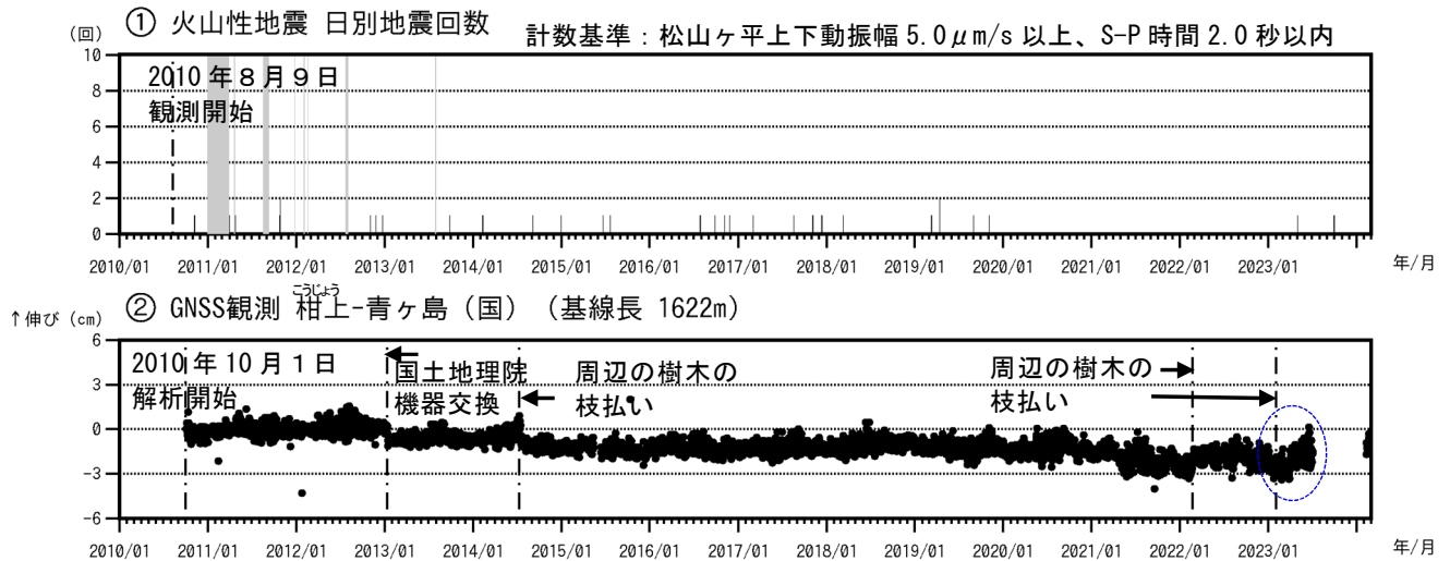
図2 青ヶ島 火山活動経過図（2010年8月9日～2024年2月29日）
