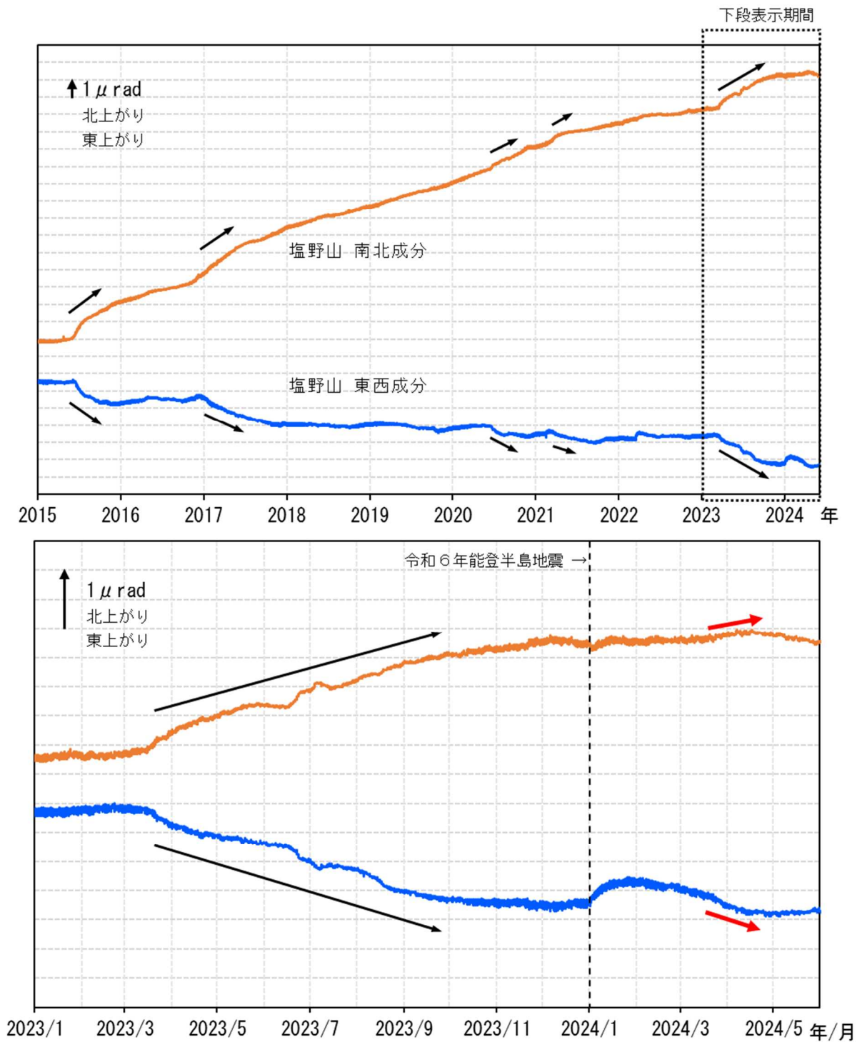
図6 浅間山 塩野山観測点における傾斜データ（2015年1月1日～2024年5月31日）
