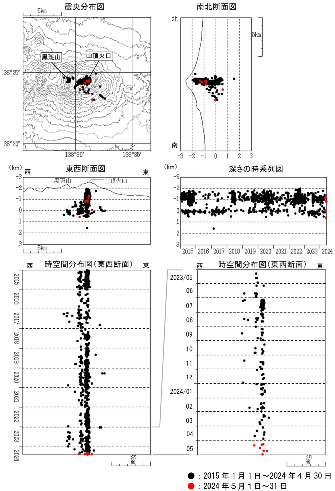
図5 浅間山 震源分布図（2015 年 1 月 1 日～2024 年 5 月 31 日）
