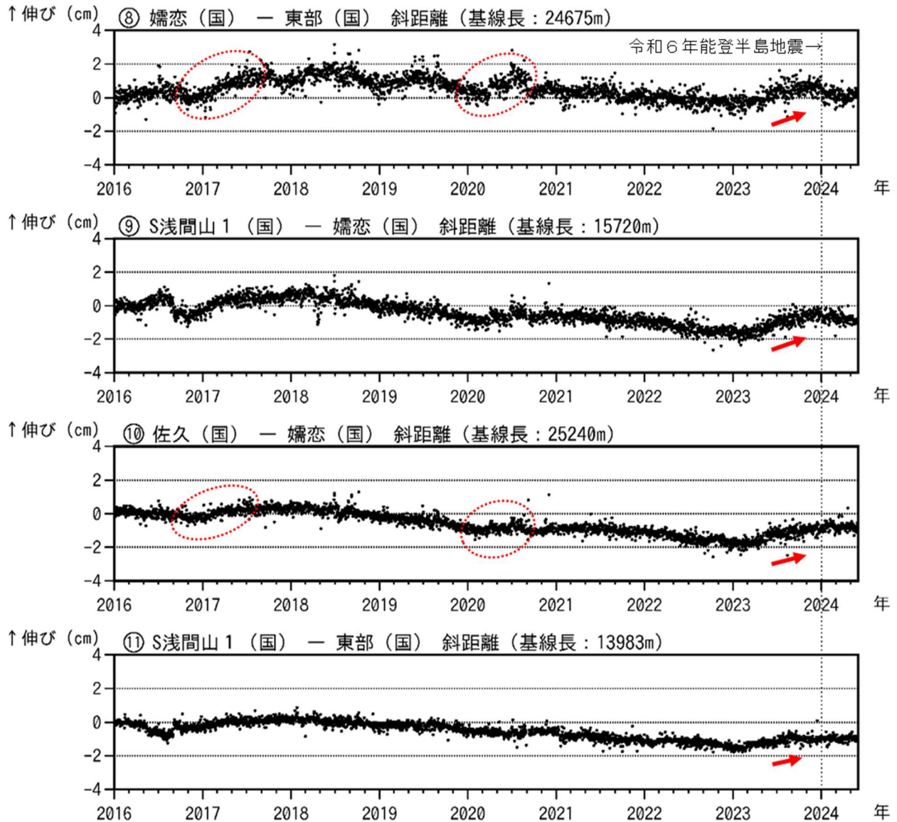
図7-2 浅間山 GNSS 連続観測結果(2016年1月1日～2024年5月31日)
