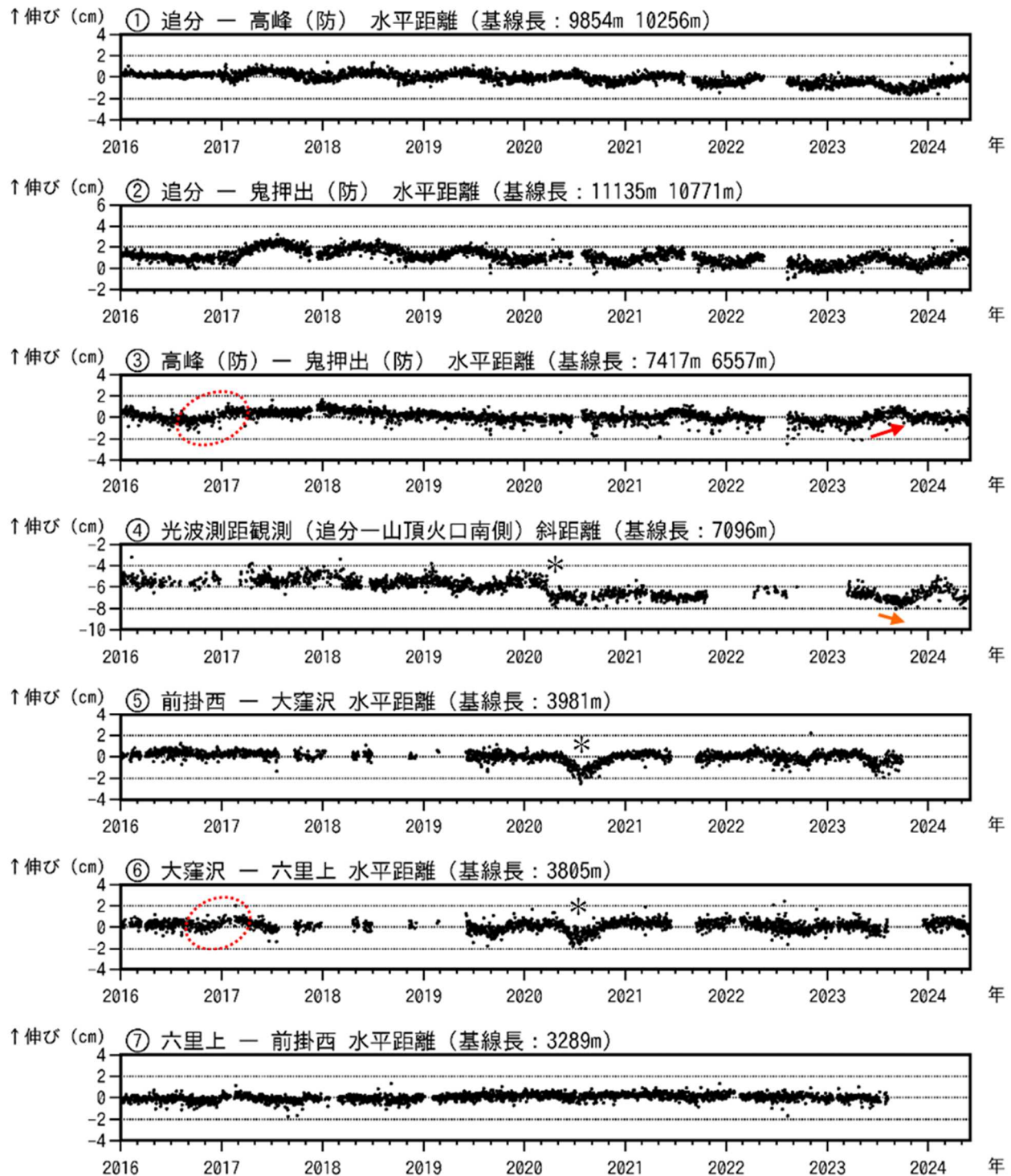
図7-1 浅間山 GNSS 連続観測及び光波測距観測結果(2016年1月1日~2024年5月31日)
