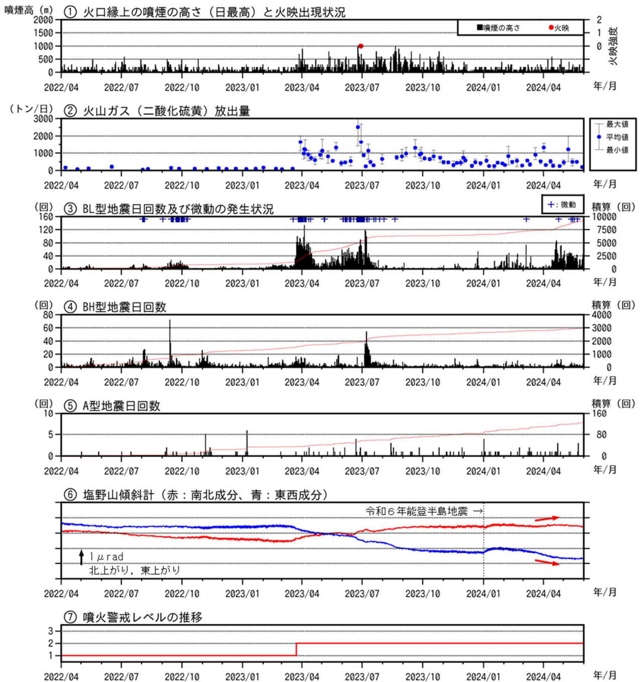
図2 浅間山 短期火山活動経過図（2022年4月1日～2024年5月31日）
