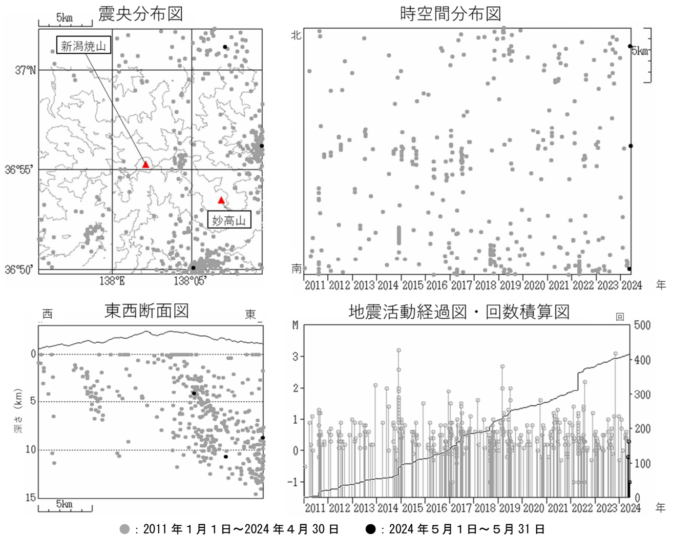
図4 新潟焼山 広域地震観測網による山体・周辺の地震活動（2011 年 1 月 1 日～2024 年 5 月 31 日）
