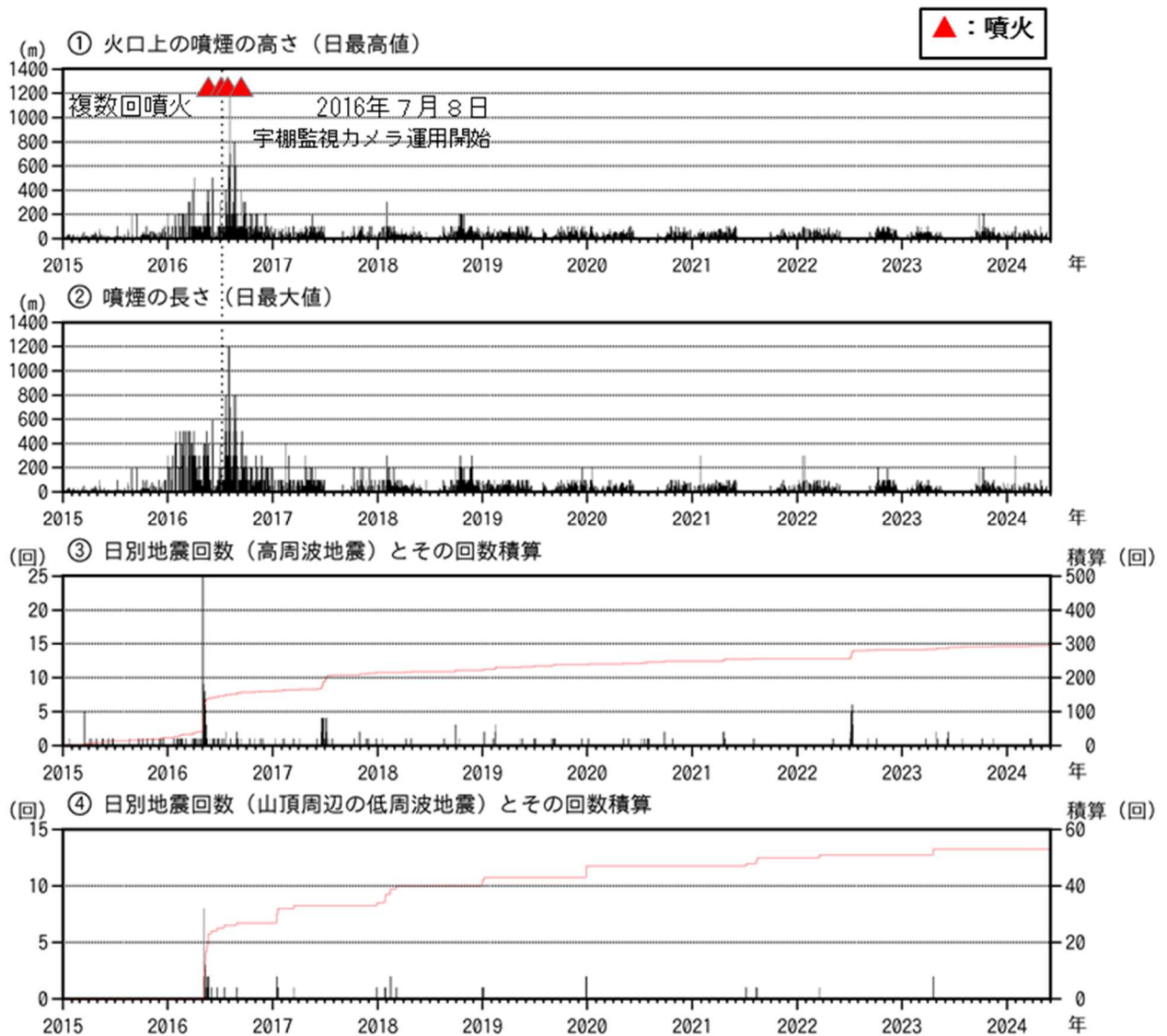
図3 新潟焼山 火山活動経過図（短期）（2015年1月1日～2024年5月31日）
