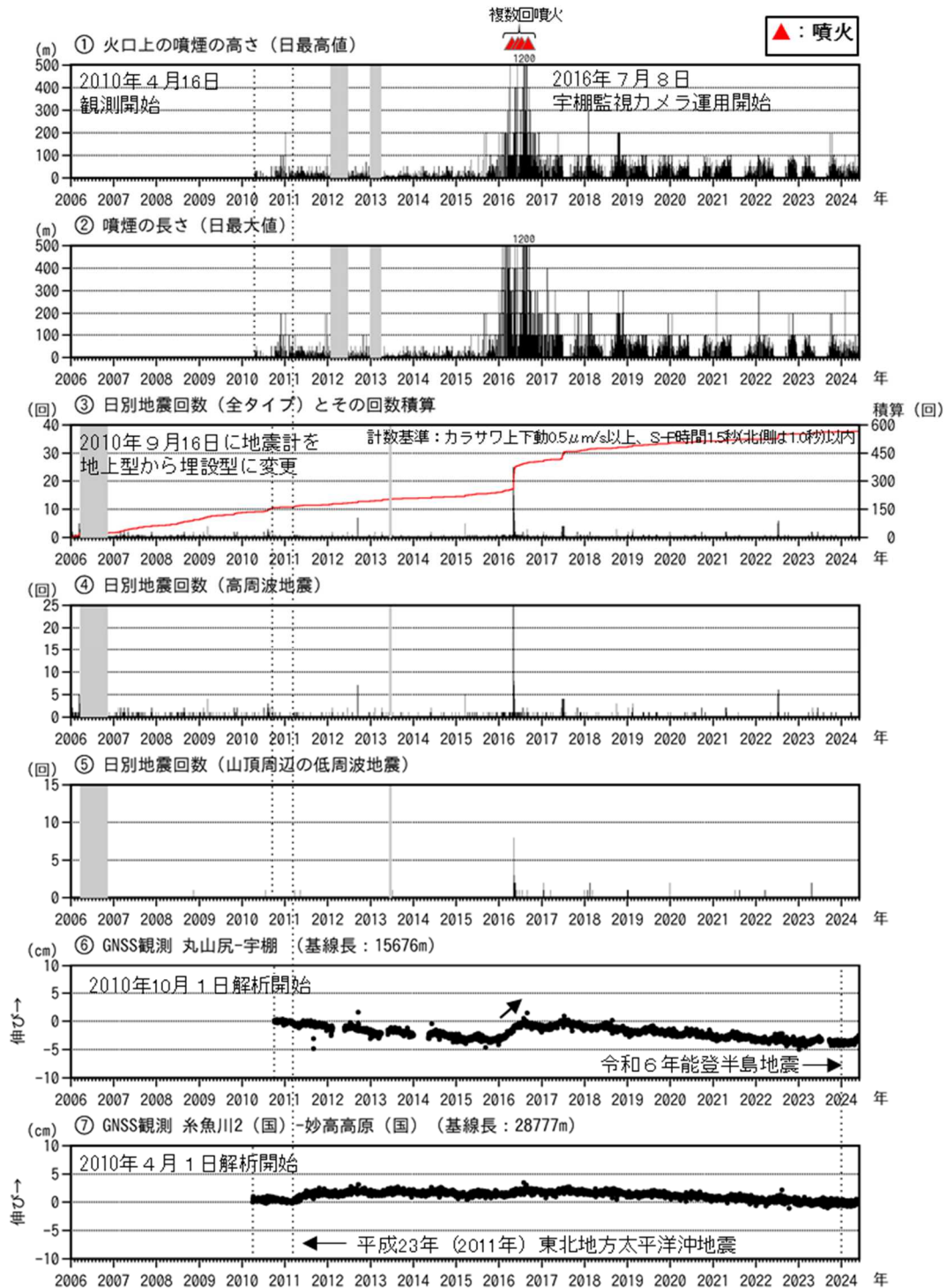
図2 新潟焼山 火山活動経過図（2006年1月1日～2024年5月31日）
