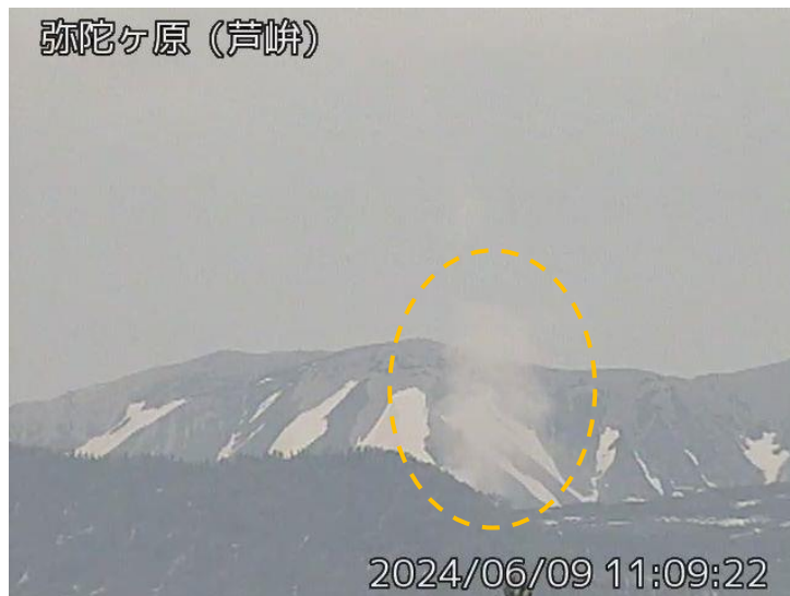
図1 弥陀ヶ原 地獄谷からの噴気の状況（橙丸）（6月9日、芦峠監視カメラによる）
