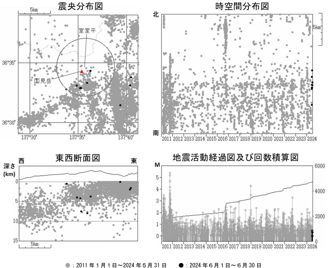
図2 弥陀ヶ原 広域地震観測網による山体・周辺の地震活動（2011 年 1 月 1 日～2024 年 6 月 30 日） 震央分布図中の円は弥陀ヶ原の計数対象地震（室堂平で S-P 時間 1 秒以内）のおよその範囲を示しています。 広域地震観測網により震源決定したもので、深さは全て海面以下として決定しています。 図中の震源要素は一部暫定値が含まれており、後日変更することがあります。 この図では、関係機関の地震波形を一元的に処理し、地震観測点の標高を考慮する等した手法で得られた震源を用いています（ただし、2020 年 8 月以前の地震については火山活動評価のための参考震源です）。
