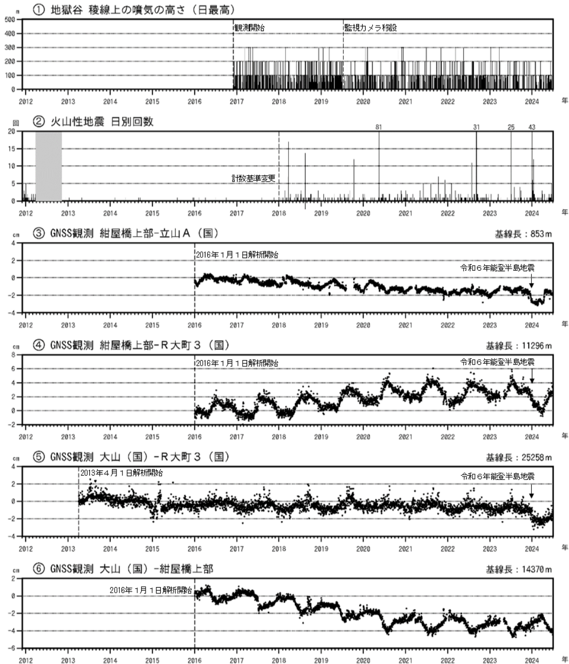
図3 弥陀ヶ原 火山活動経過図（2011年12月1日～2024年6月30日）
