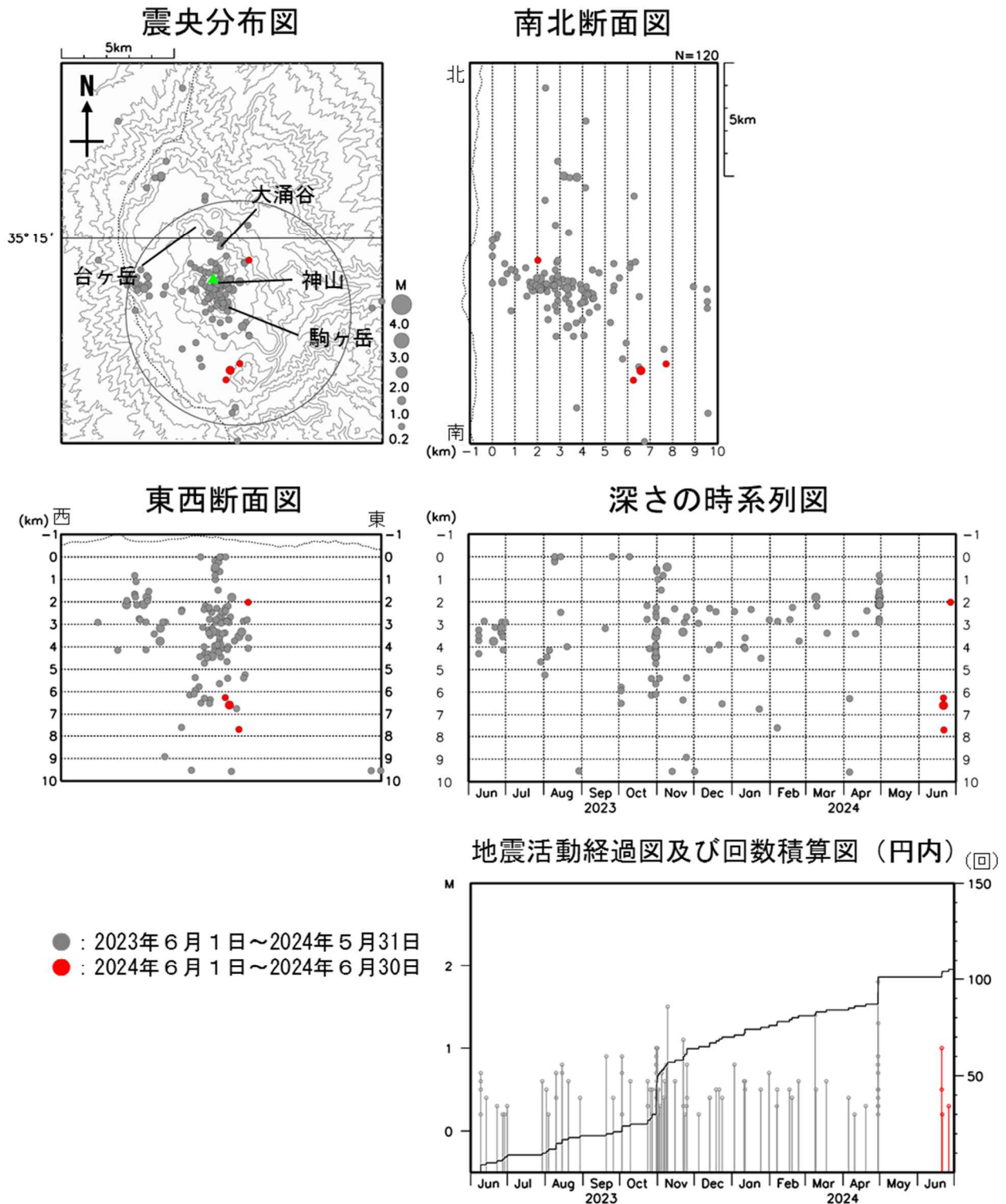
図4 箱根山 広域地震観測網による山体周辺の震源分布図（2023年6月1日～2024年6月30日）
