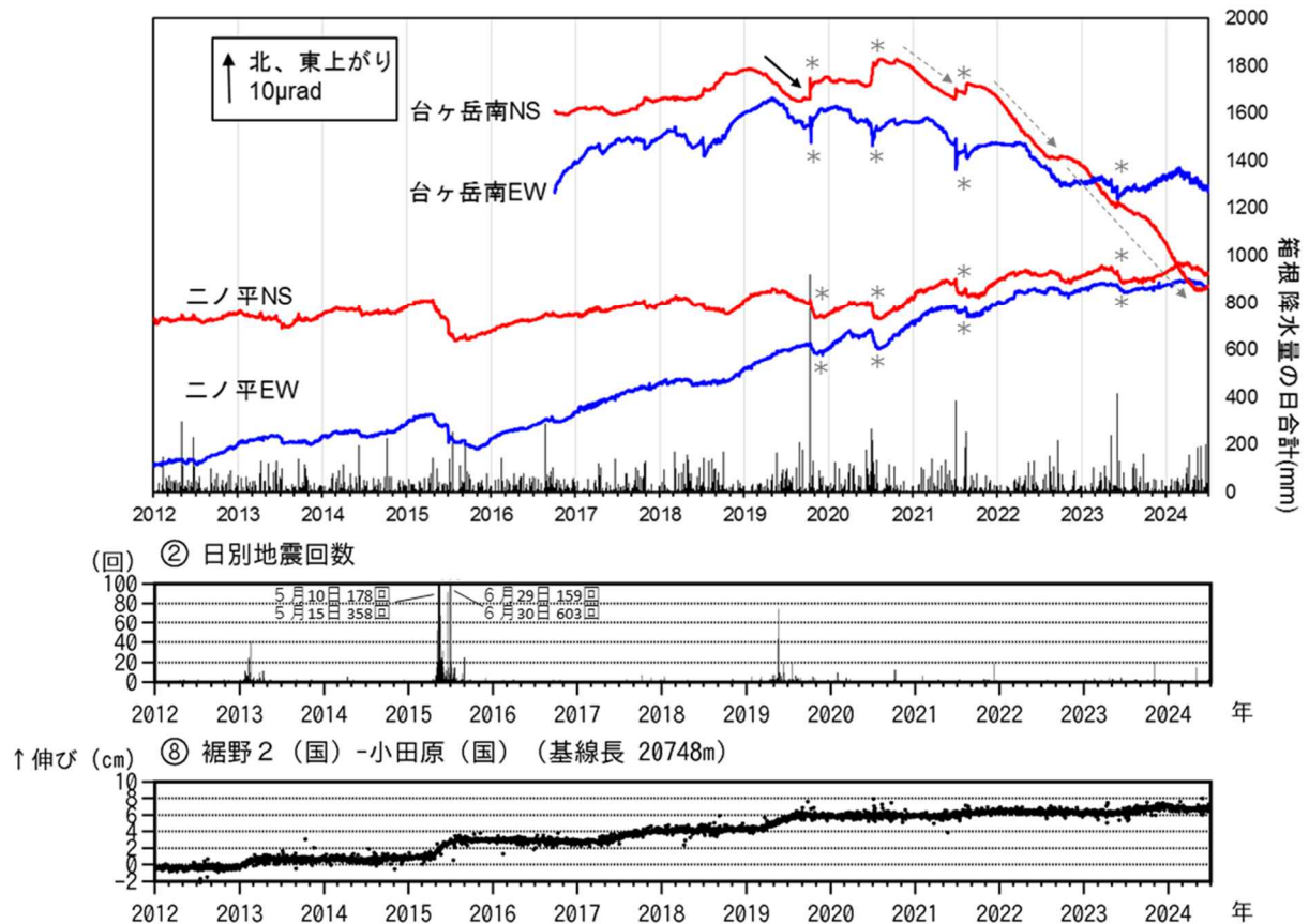
図5 箱根山 傾斜観測及び地震回数・GNSS観測（2012年1月1日～2024年6月30日）
