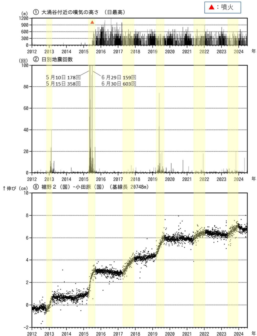
図3-1 箱根山 火山活動経過図（2012年1月1日～2024年6月30日）
