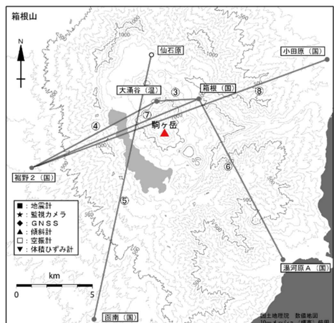
図3-2 箱根山 GNSS 連続観測による 基線長変化及び観測点配置図 (2012年1月1日～2024年6月30日) (国)：国土地理院 (温)：神奈川県温泉地学研究所 空白部分は欠測を示します。
