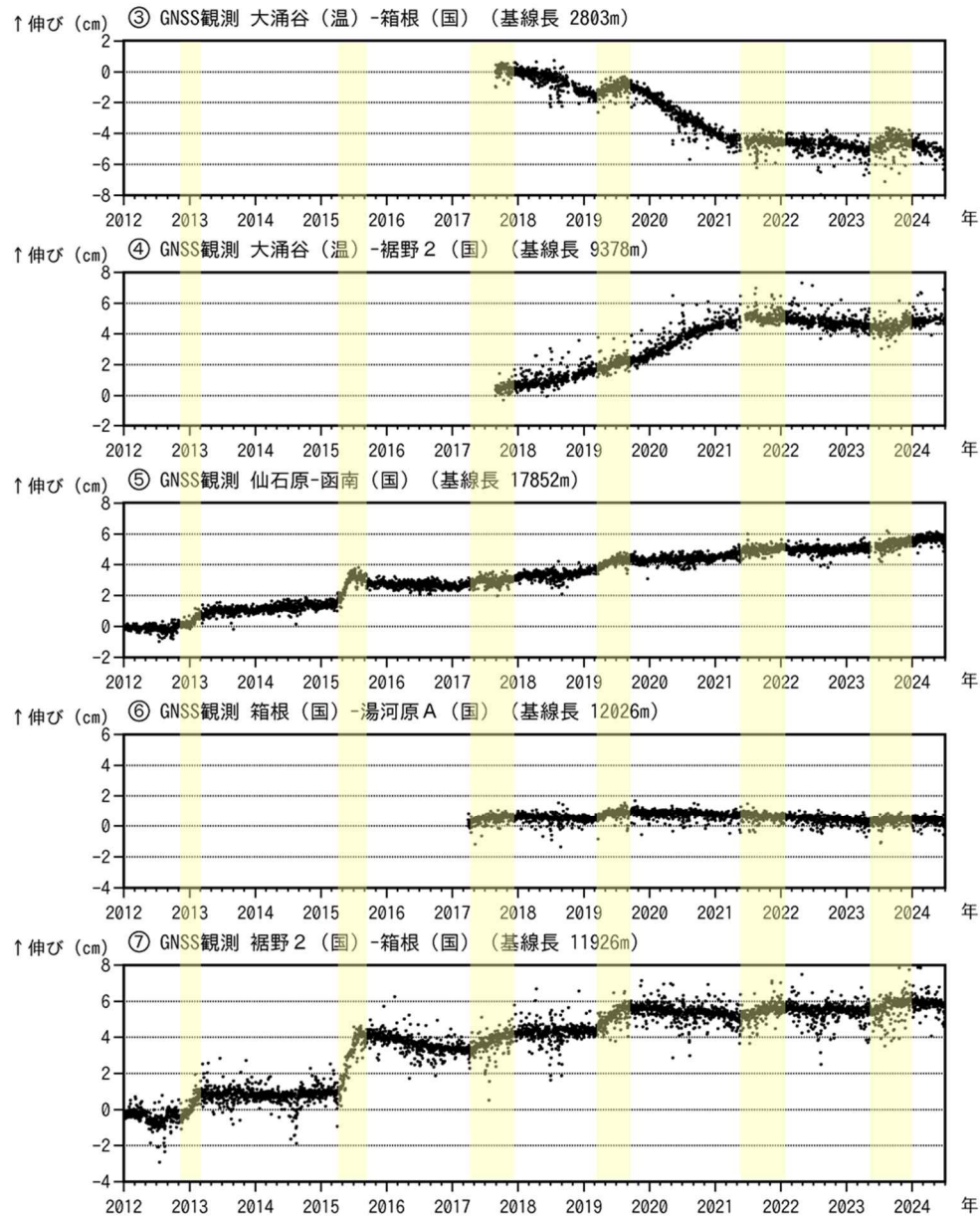
図3-2 箱根山 GNSS 連続観測による 基線長変化及び観測点配置図 (2012年1月1日～2024年6月30日) (国)：国土地理院 (温)：神奈川県温泉地学研究所 空白部分は欠測を示します。
