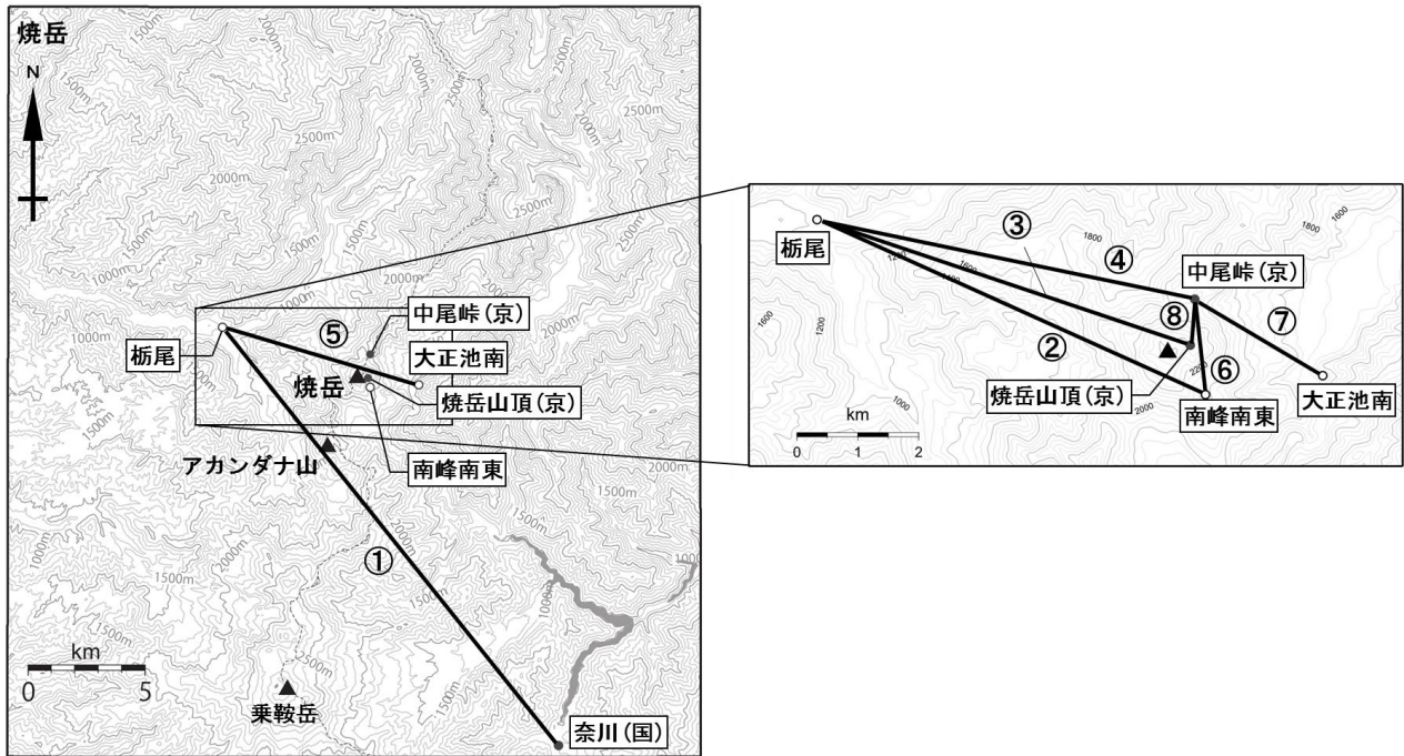
図8 焼岳 GNSS 連続観測点配置
