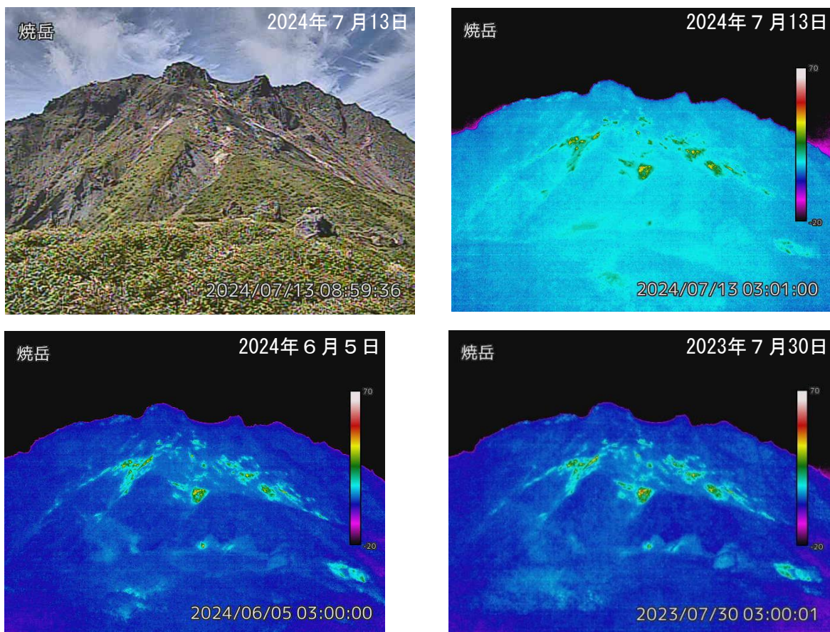
図4 焼岳 中尾峠赤外熱映像カメラによる焼岳の北側斜面の地表面温度分布と可視画像 撮影場所と撮影方向は図12を参照。 ・前月（左下図）及び前年（右下図）と比較して、噴気の状態や地表面温度分布に特段の変化はありません。
