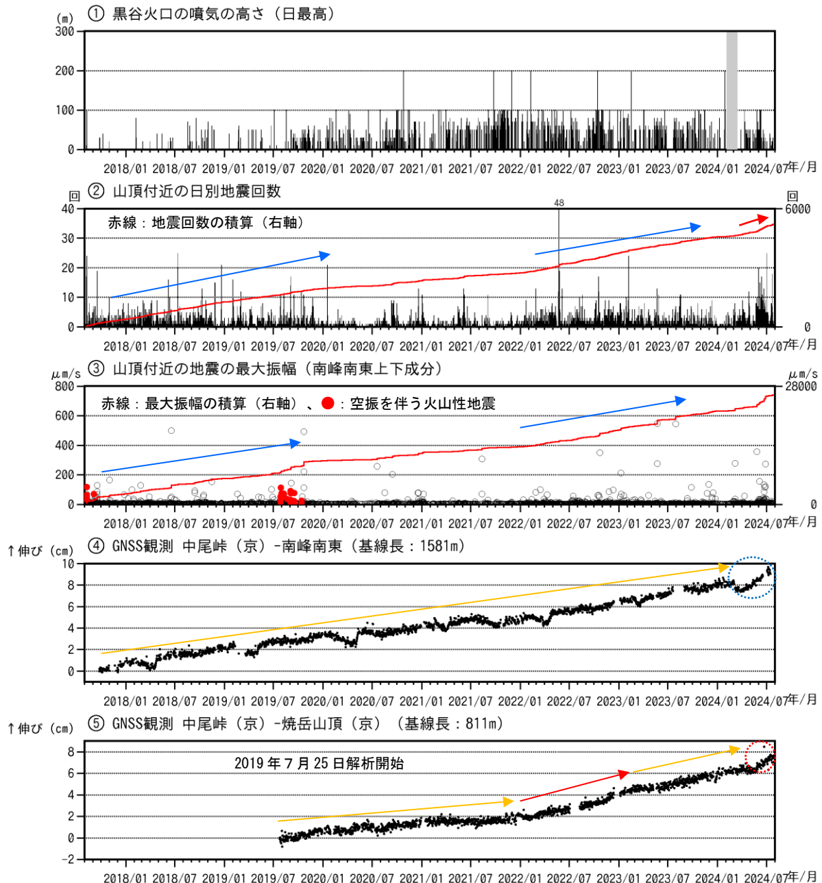
図1-1 焼岳 火山活動経過図（2017年8月1日～2024年7月31日）
