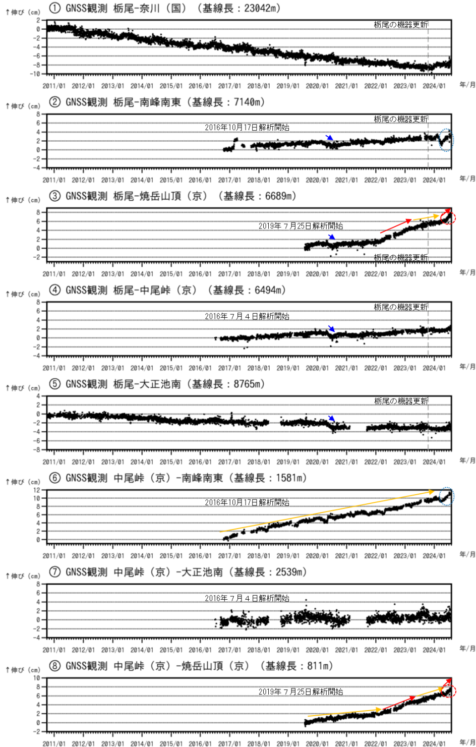
図7 焼岳 GNSS 連続観測による基線長変化（2010年10月1日～2024年7月31日）
