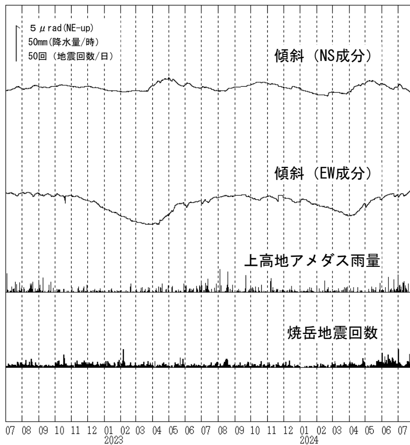
図9 焼岳 南峰南東観測点における傾斜データ（2022年7月1日～2024年7月31日）
