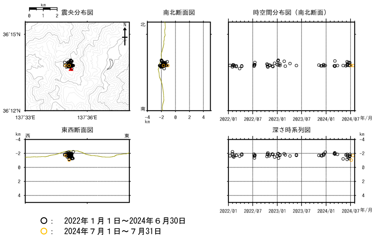
図2 焼岳 山頂付近の地震の震源分布図（2022年1月1日～2024年7月31日）
