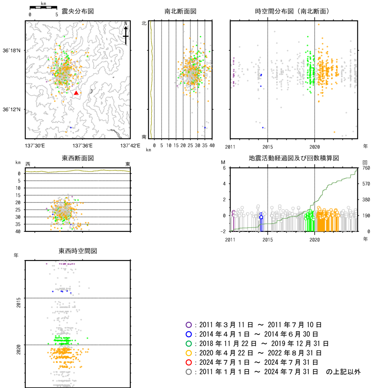
図11 焼岳 広域地震観測網による深部低周波地震の震源分布図（2011年1月1日～2024年7月31日） 広域地震観測網により震源決定したもので、深さは全て海面以下として決定しています。そのため、山頂付近の浅い地震の震源も海面下に決定されています。 M（マグニチュード）は地震の規模を表します。 図中の震源要素は一部暫定値が含まれており、後日変更することがあります。 ・ 焼岳の北西側の深い所を震源とする低周波地震の発生状況に特段の変化は見られません。 ・ 過去には、図6に示したような焼岳周辺の地震活動の活発化がみられた期間付近で、深部低周波地震が増加したことがあります。
