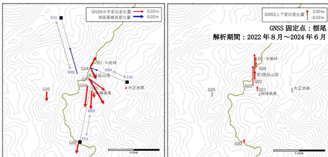
図5－2 焼岳 焼岳周辺の繰り返しGNSS観測及び光波測距観測 ベクトル図（GNSSの固定点：栃尾） ・2022年8月と2024年6月の観測結果の差を示しています。 ・2024年6月11日～13日及び18日～20日に実施した繰り返しGNSS観測では山頂付近を中心に放射状に離れる変化（左図）及び上向きの変化（右図）が観測され、光波測距観測でも同様の変化（左図）が観測されました。 各観測点は図5－3を参照。
