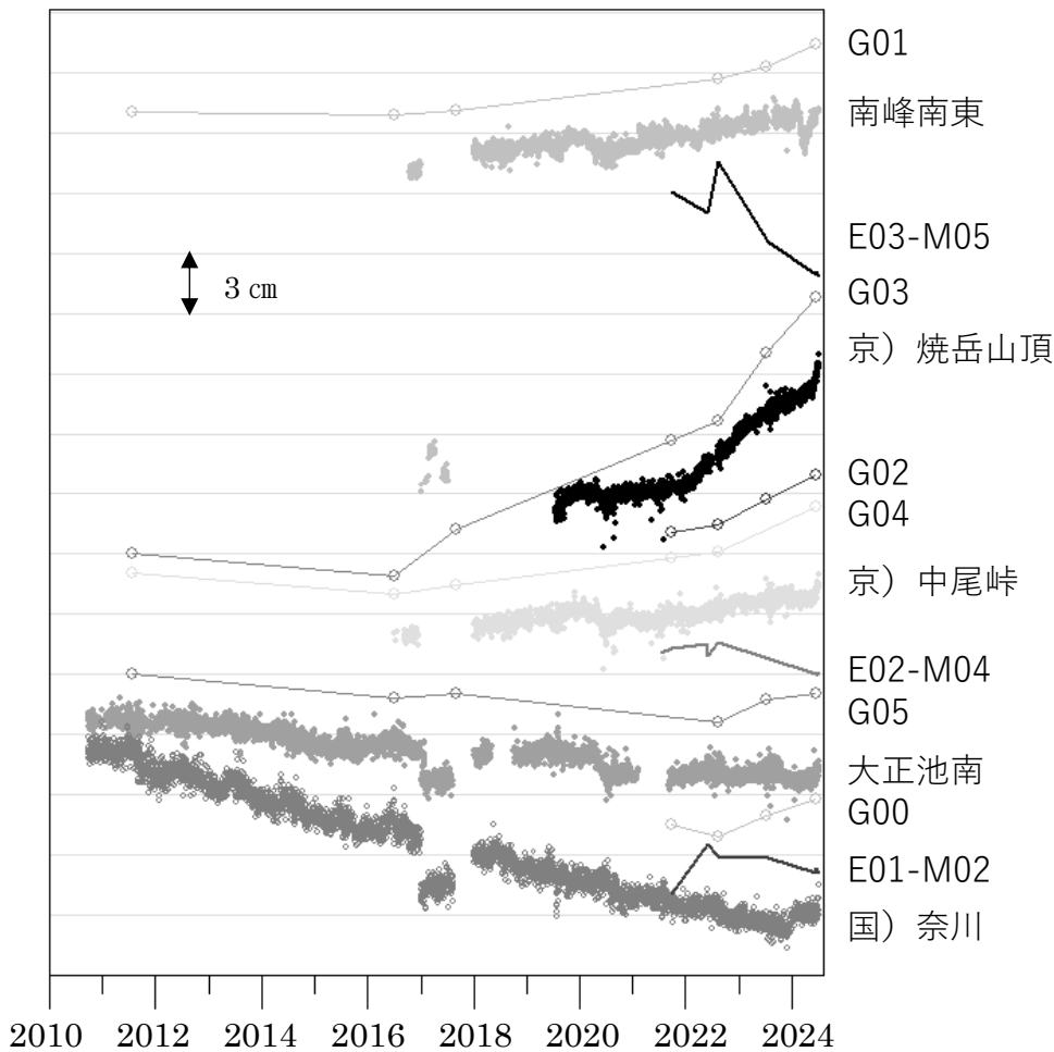
図5－1 焼岳 焼岳周辺の繰り返しGNSS観測（栃尾観測点との基線長）及び光波測距観測時系列図 各観測点は図5－3を参照。
