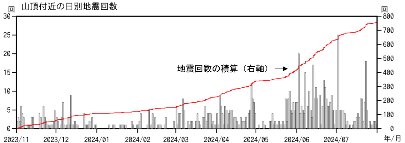
図1-2 焼岳 山頂付近の日別地震回数の推移（2023年11月1日～2024年7月31日）
