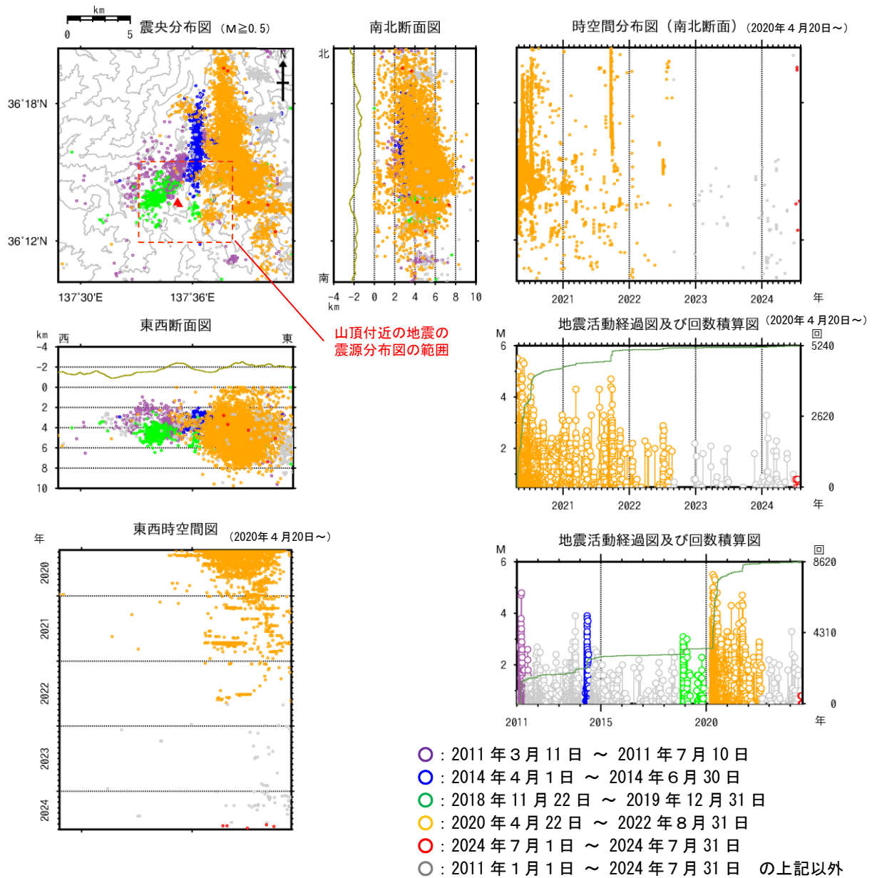
図10 焼岳 広域地震観測網による山体及び周辺の地震活動(2011年1月1日～2024年7月31日)
