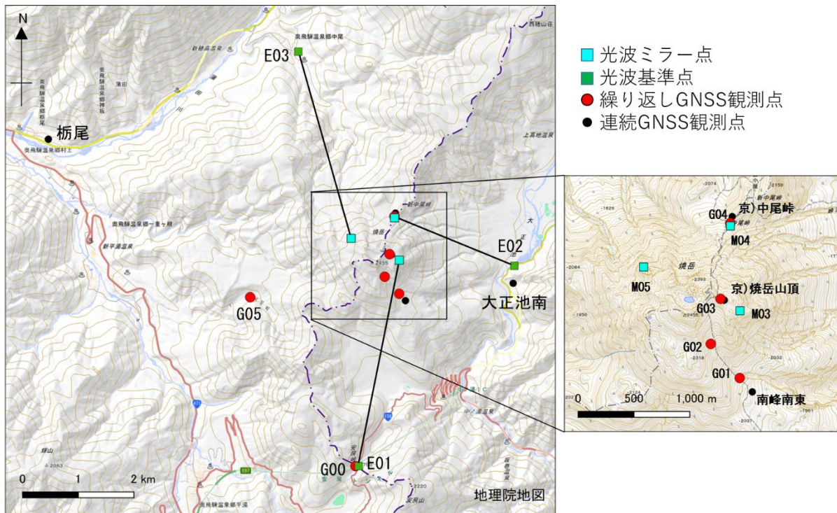
図5-3 焼岳 焼岳周辺の繰り返しGNSS観測及び光波測距観測 観測点位置図
