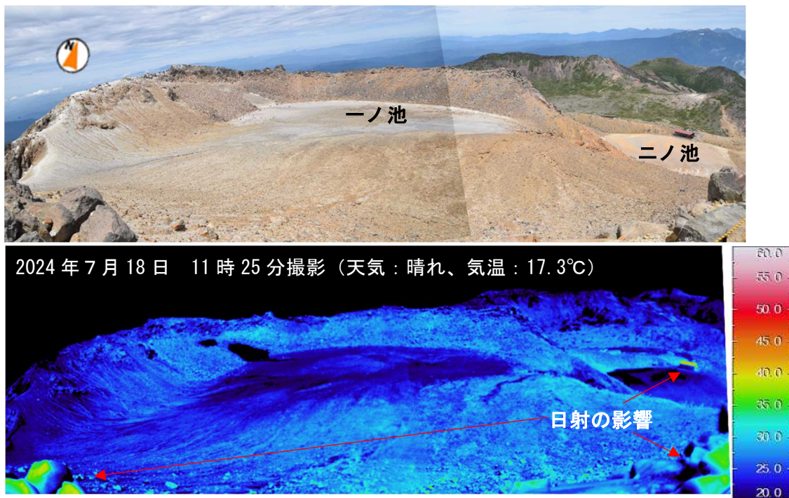
図7-2 御嶽山 一の池及び二の池の可視画像及び赤外熱映像装置による地表面温度分布 観測位置及び撮影方向は図7-1に示しています。
