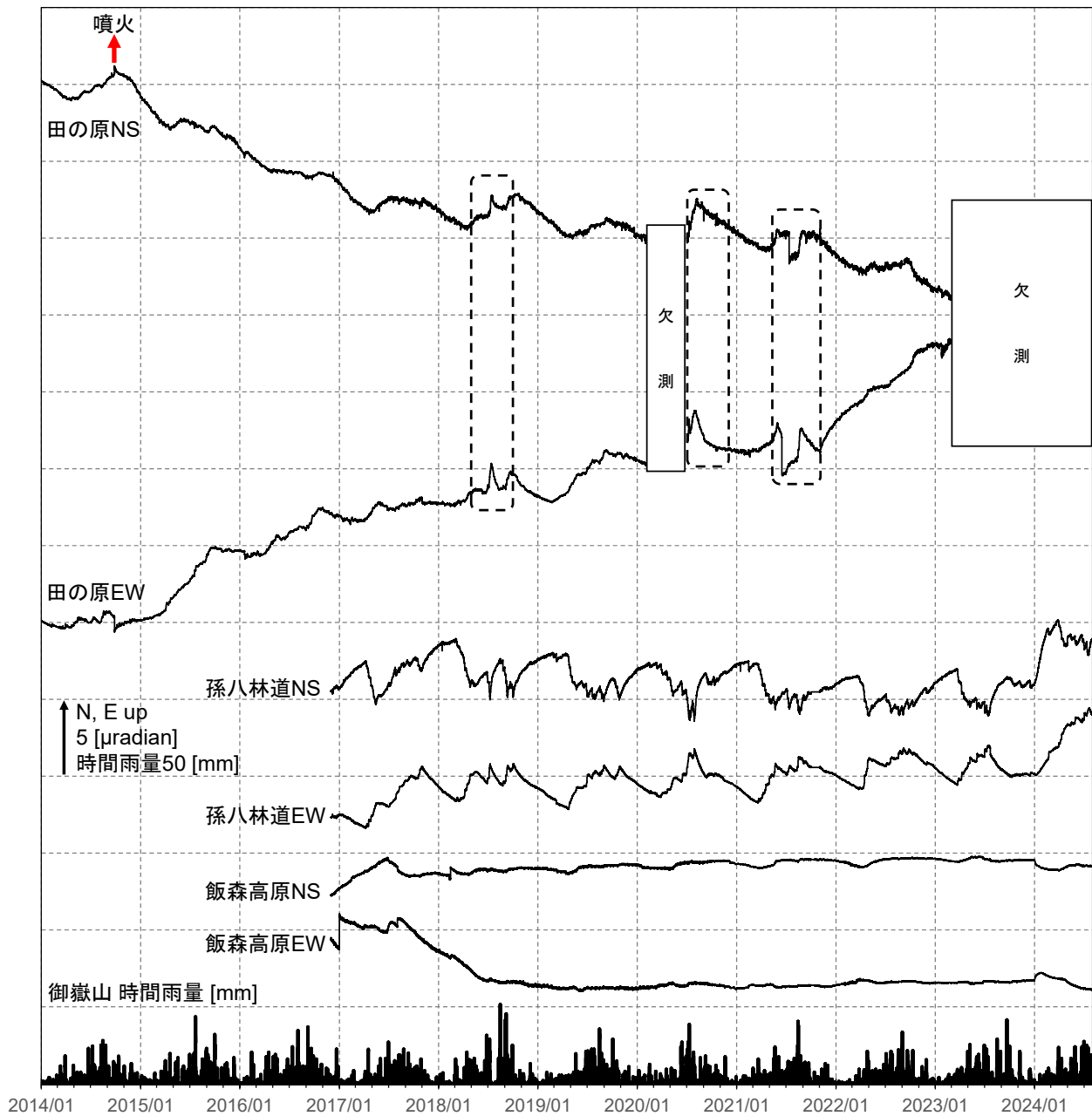
図6 御嶽山 傾斜変動（2014年1月1日～2024年7月31日）
