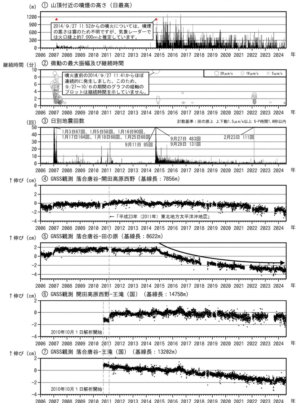
図1 御嶽山 長期間の火山活動経過図（2006年1月1日～2024年7月31日）
