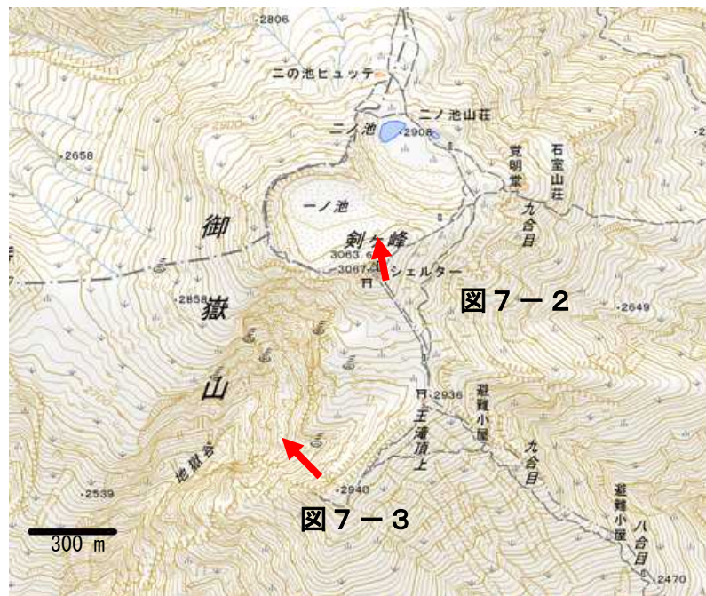
図7-1 御嶽山 現地調査での観測位置と撮影方向（赤色矢印）
