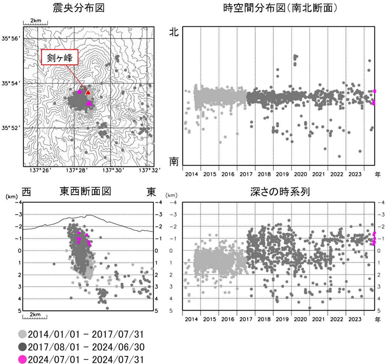
図4 御嶽山 震源分布図（2014年1月1日～2024年7月31日）
