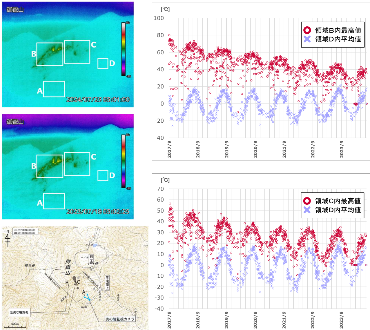
図3 御嶽山 奥の院赤外熱映像カメラによる剣ヶ峰南西側における最高温度の推移 (2017年9月13日～2024年7月31日)
