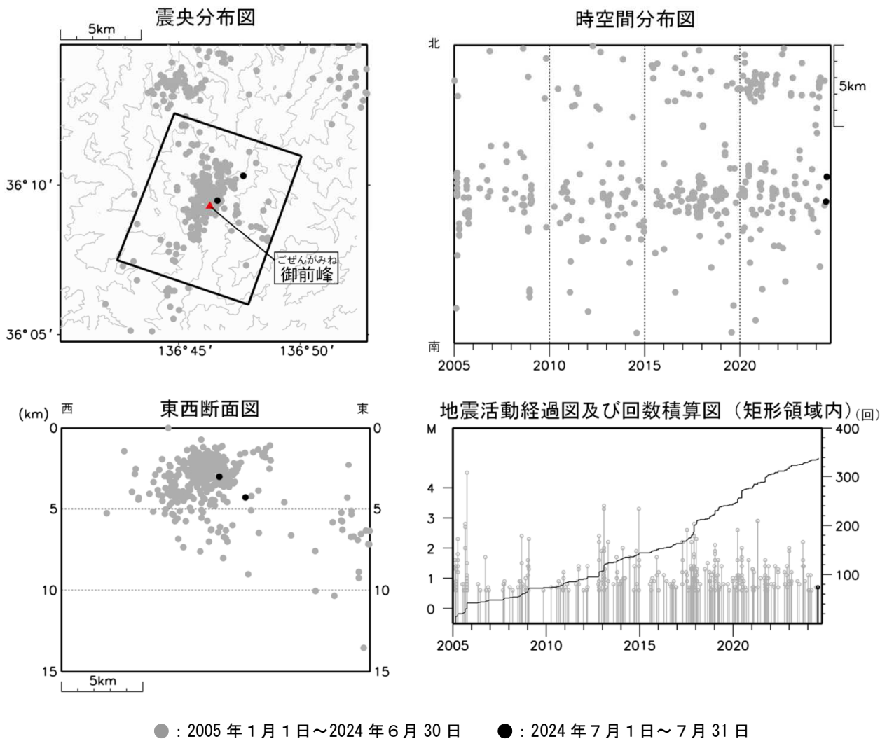
図4 白山 広域地震観測網による山体・周辺の地震活動（2005年1月1日～2024年7月31日）
