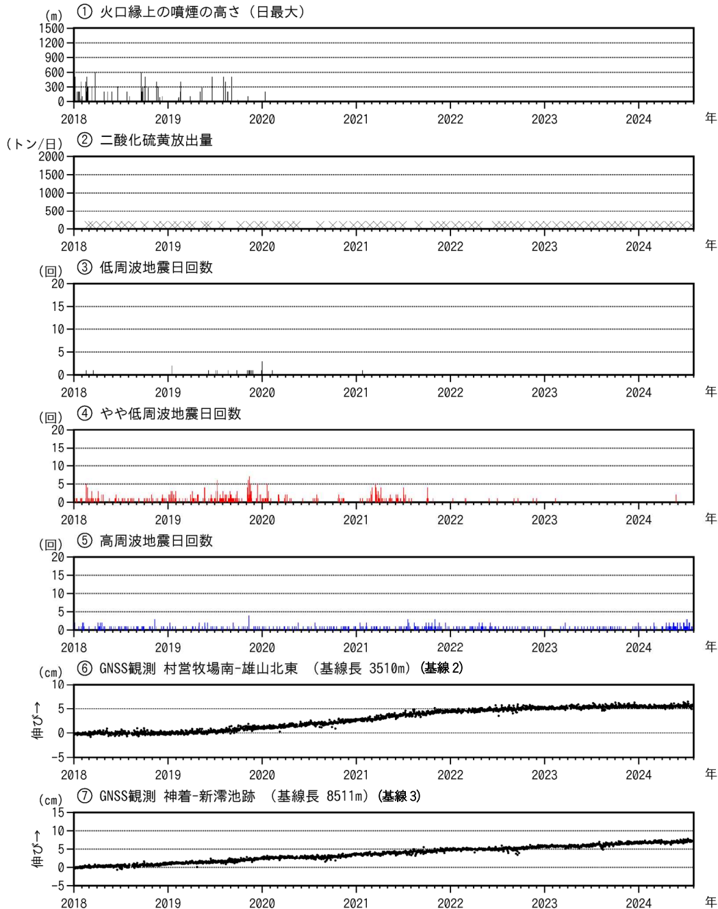
図5 三宅島 火山活動経過図（2018年1月1日～2024年7月31日）
