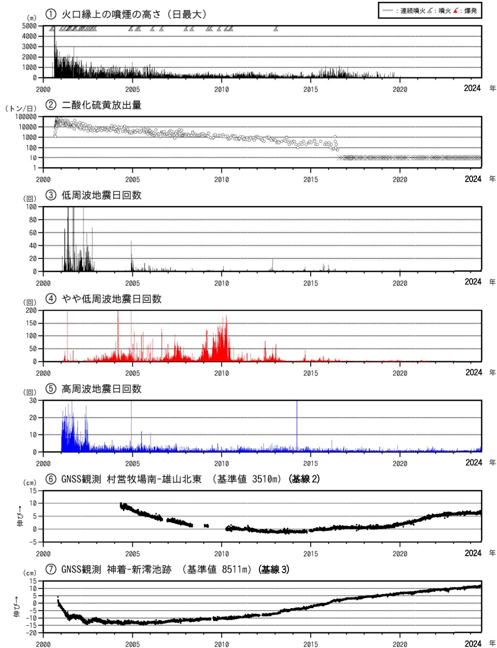
図6 三宅島 長期の火山活動経過図（2000年1月1日～2024年7月31日）
