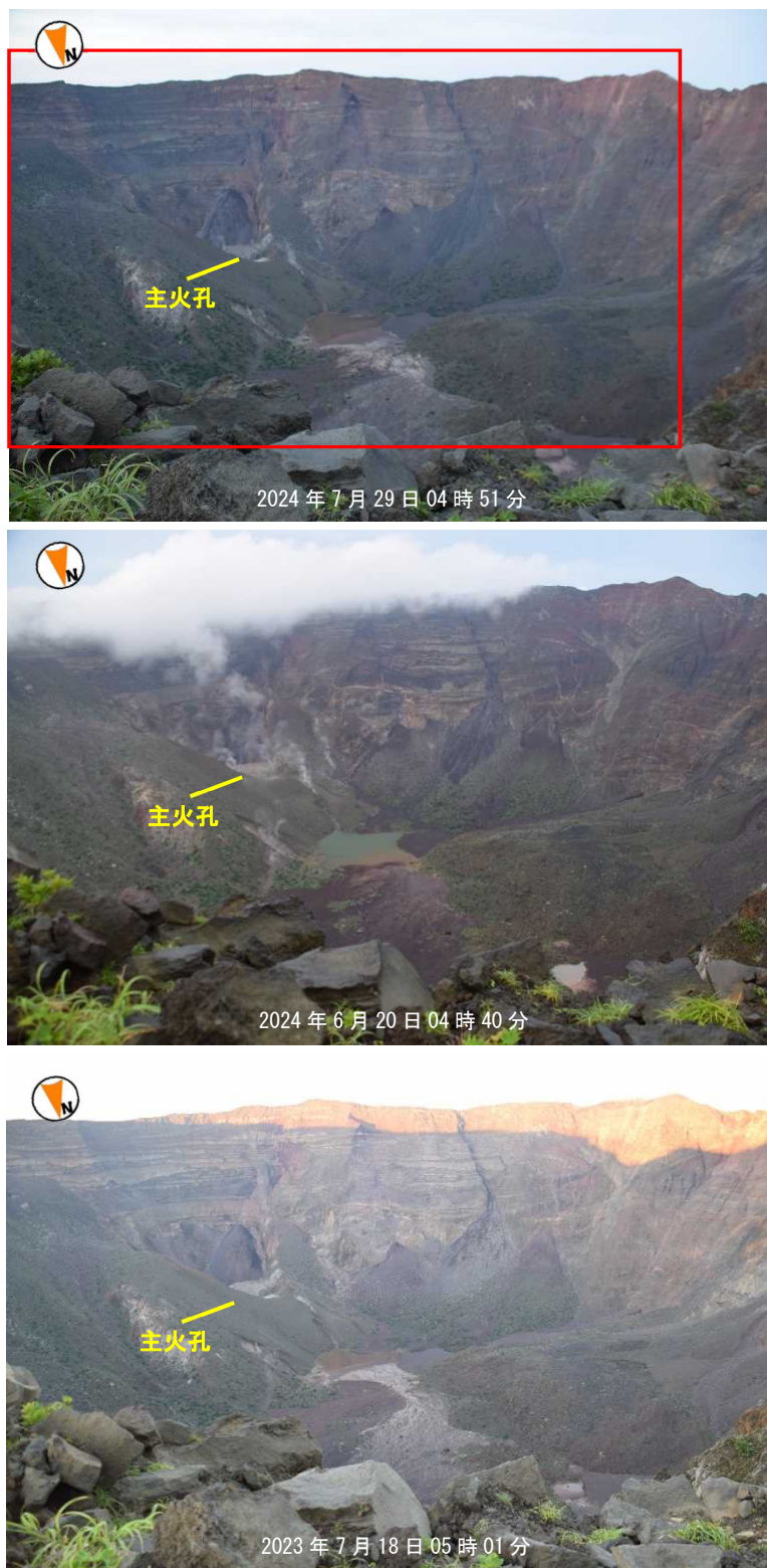
図3 三宅島 山頂火口内の状況（スオウ穴から撮影） ※図中の赤四角は図4の赤外熱映像の範囲を示しています。
