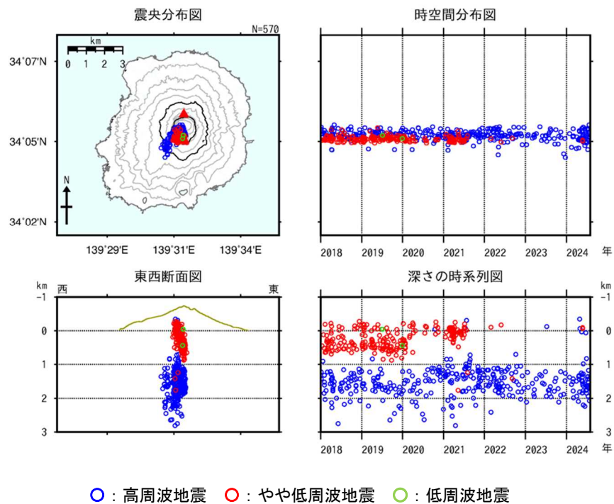
図8 三宅島 震源分布図
