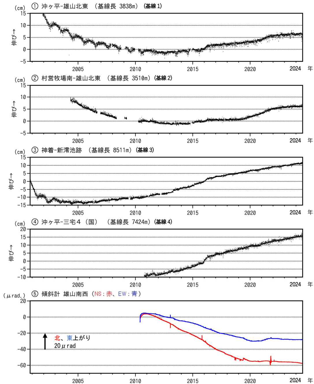
図7 三宅島 GNSS 連続観測及び傾斜計観測結果（2000年10月26日～2024年7月31日）
