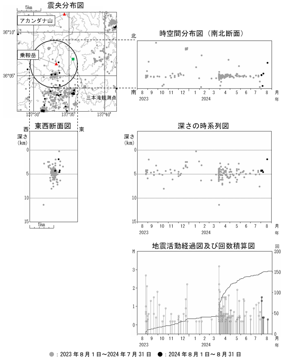
図3 乗鞍岳 広域地震観測網による山体・周辺の地震活動(2023 年 8 月 1 日～2024 年 8 月 31 日)
