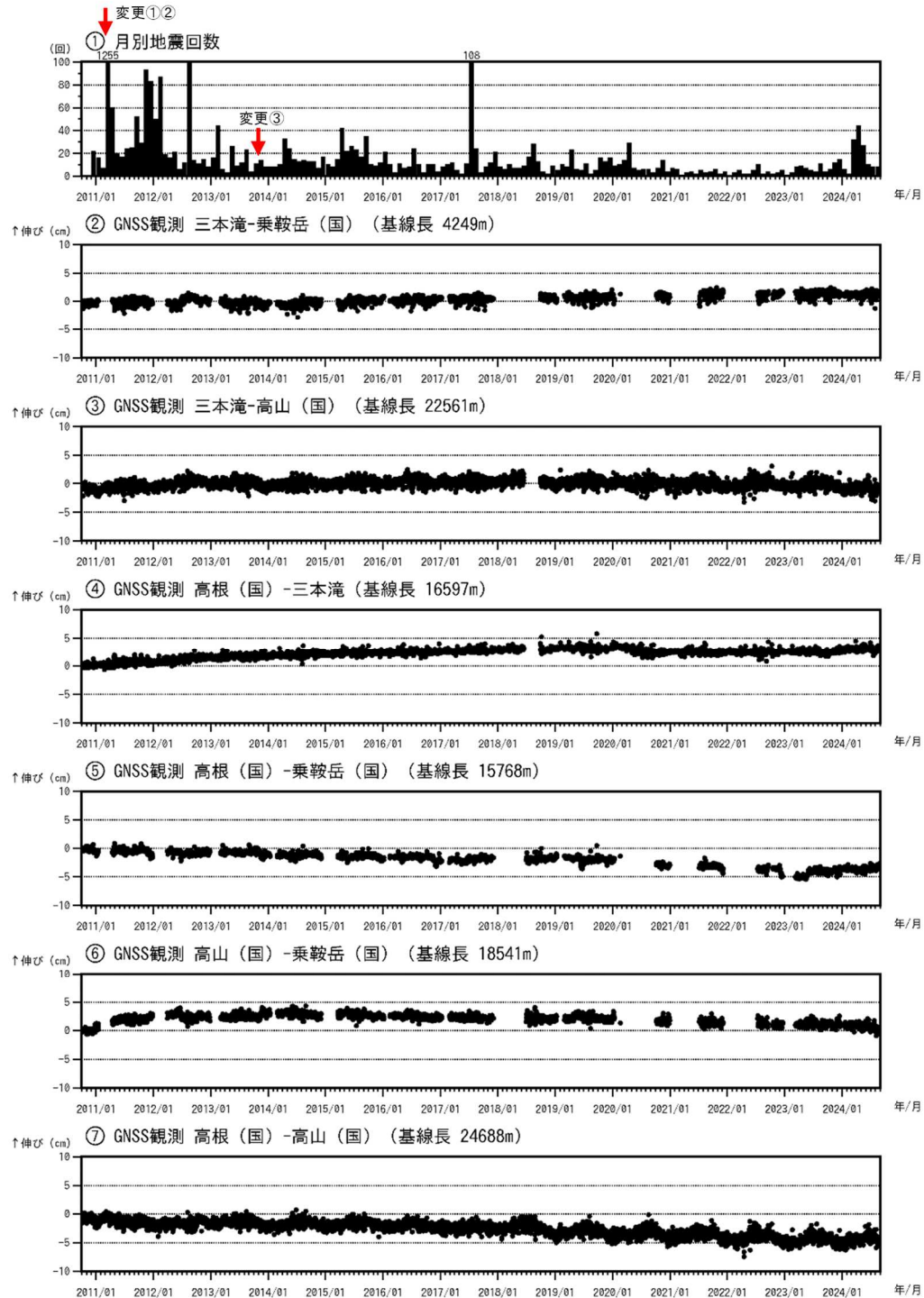
図2 乗鞍岳 火山活動経過図（2010年10月1日～2024年8月31日）
