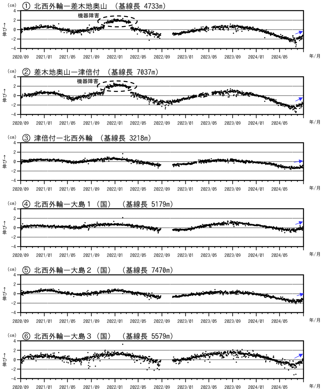
図3-2 伊豆大島 GNSS 連続観測による基線長変化(2020年9月～2024年8月31日)
