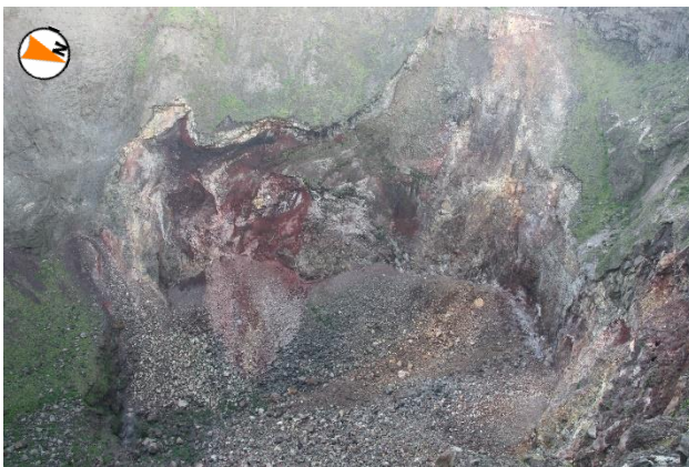
中央火孔東カメラ位置からの可視画像 （7月23日 現地調査時に撮影）
