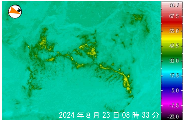
中央火孔東カメラ位置からの熱画像 （8月23日 現地調査時に撮影）
