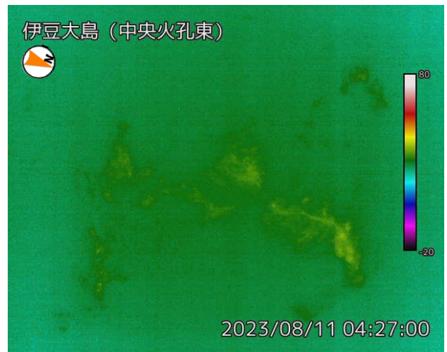
2023年8月11日 中央火孔東監視カメラによる
