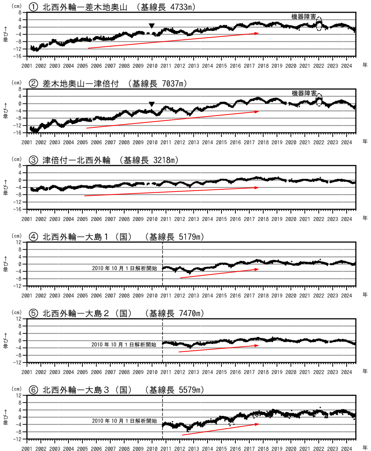
図3-1 伊豆大島 GNSS 連続観測による基線長変化(2001年1月～2024年8月31日)
