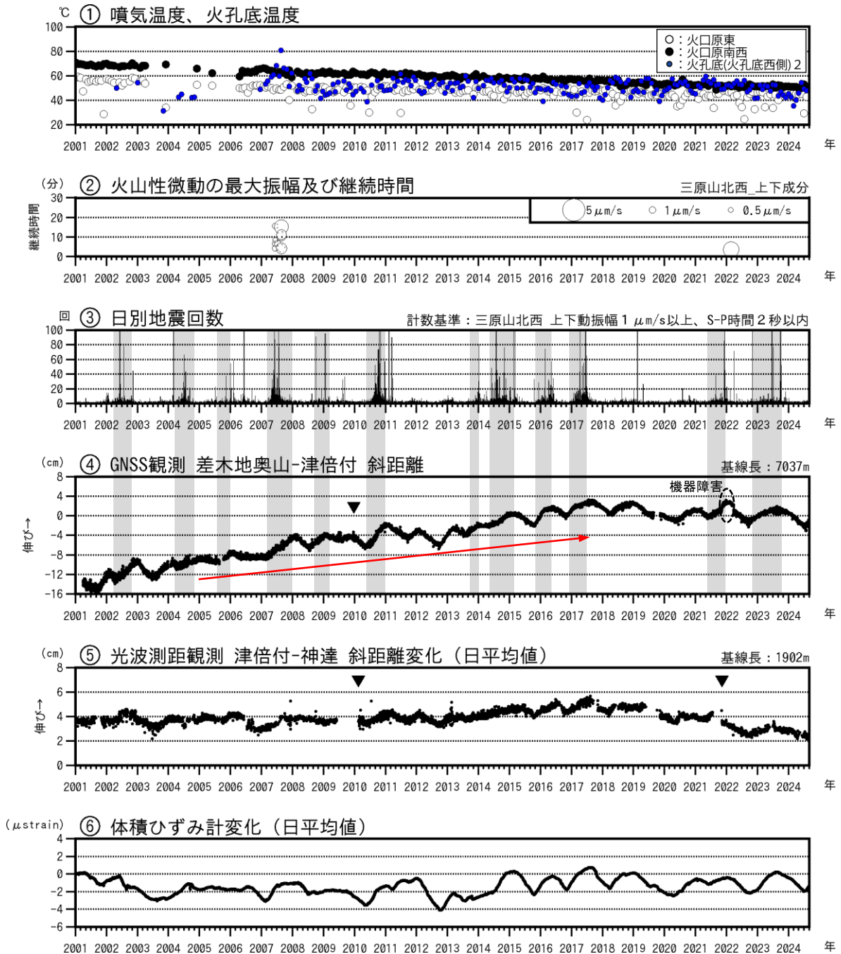
図2 伊豆大島 最近の火山活動経過図（2001年1月～2024年8月31日）
