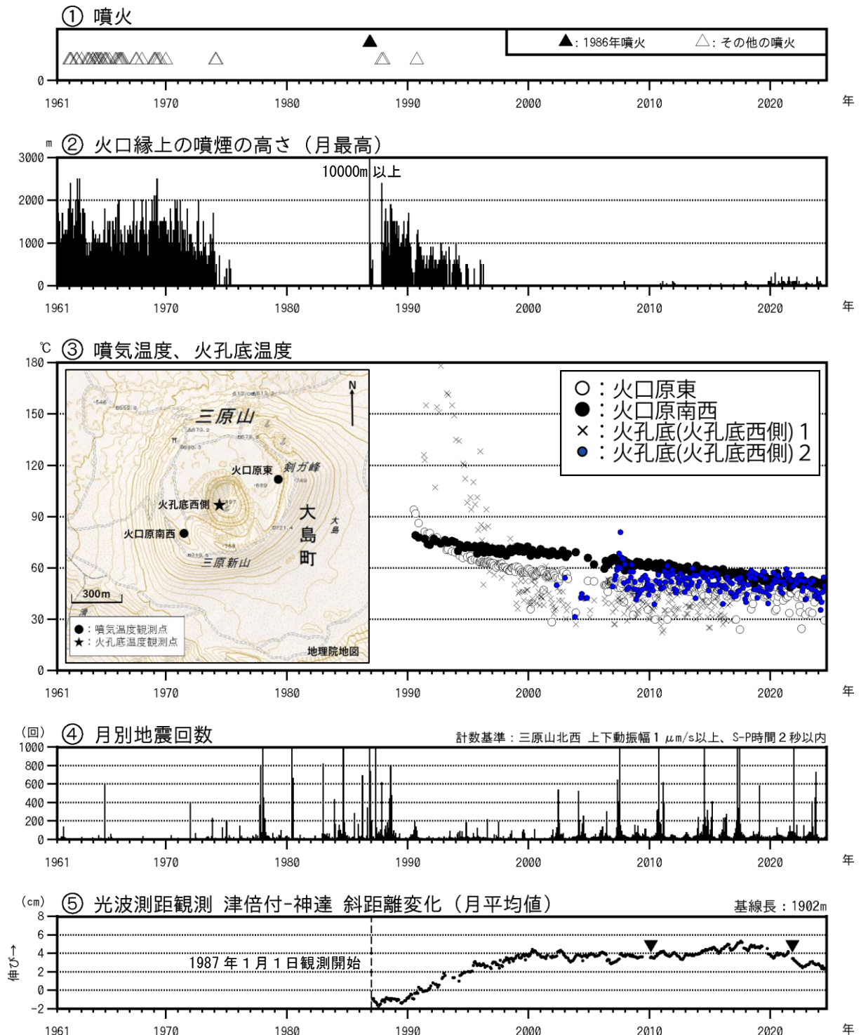
図1 伊豆大島 長期間の火山活動経過図（1961年1月～2024年8月31日）
