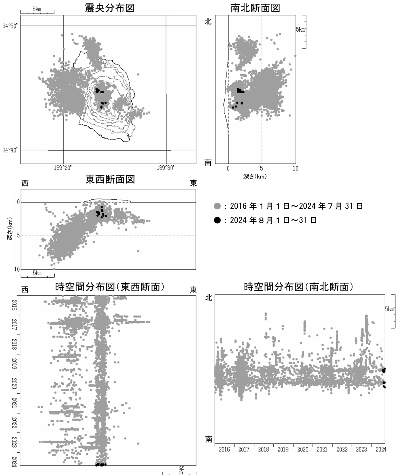
図4 伊豆大島 震源分布図（2016 年 1 月 1 日～2024 年 8 月 31 日）
