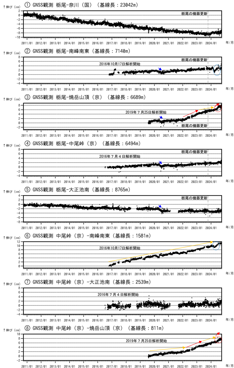
図6 焼岳 GNSS 連続観測による基線長変化（2010年10月1日～2024年9月30日）
