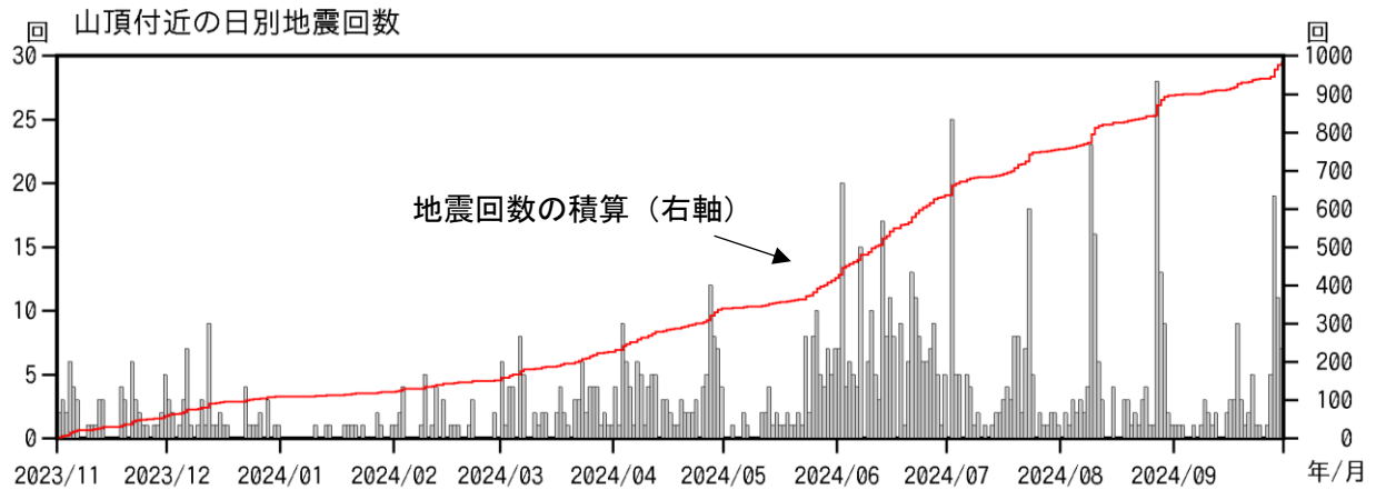
図1-2 焼岳 山頂付近の日別地震回数の推移（2023年11月1日～2024年9月30日）
