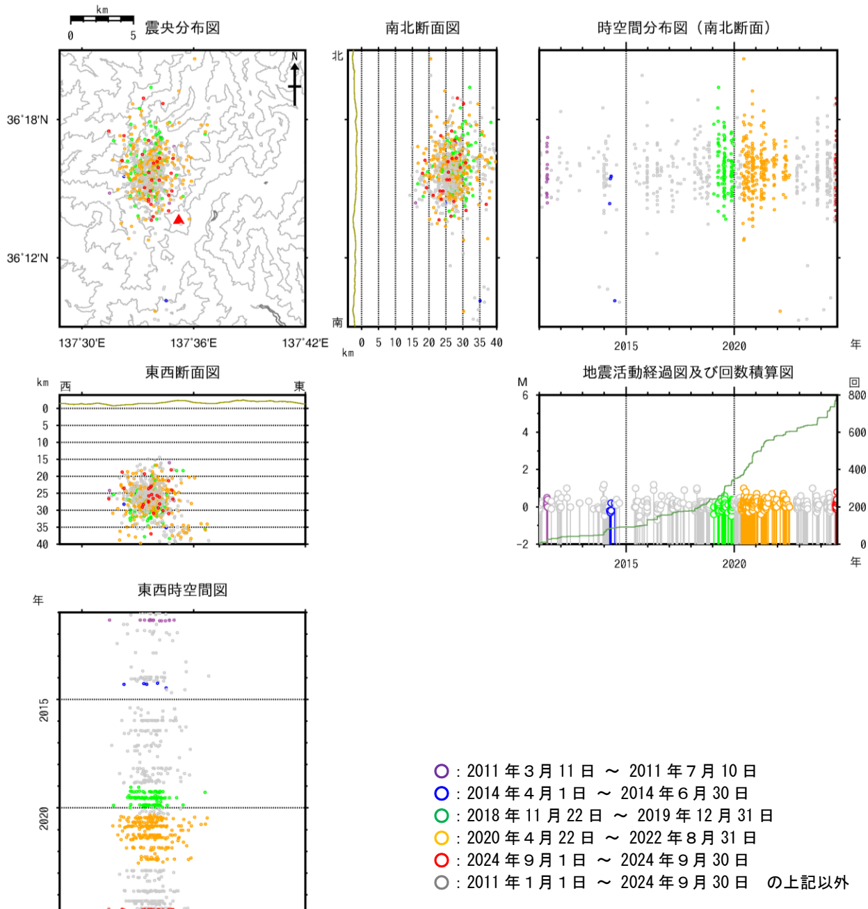
図10 焼岳 広域地震観測網による深部低周波地震の震源分布図（2011年1月1日～2024年9月30日） 広域地震観測網により震源決定したもので、深さは全て海面以下として決定しています。そのため、山頂付近の浅い地震の震源も海面下に決定されています。 M（マグニチュード）は地震の規模を表します。 図中の震源要素は一部暫定値が含まれており、後日変更することがあります。 ・焼岳の北西側の深い所を震源とする低周波地震の発生状況に特段の変化は見られません。 ・過去には、図9に示したような焼岳周辺の地震活動の活発化がみられた期間付近で、深部低周波地震が増加したことがあります。
