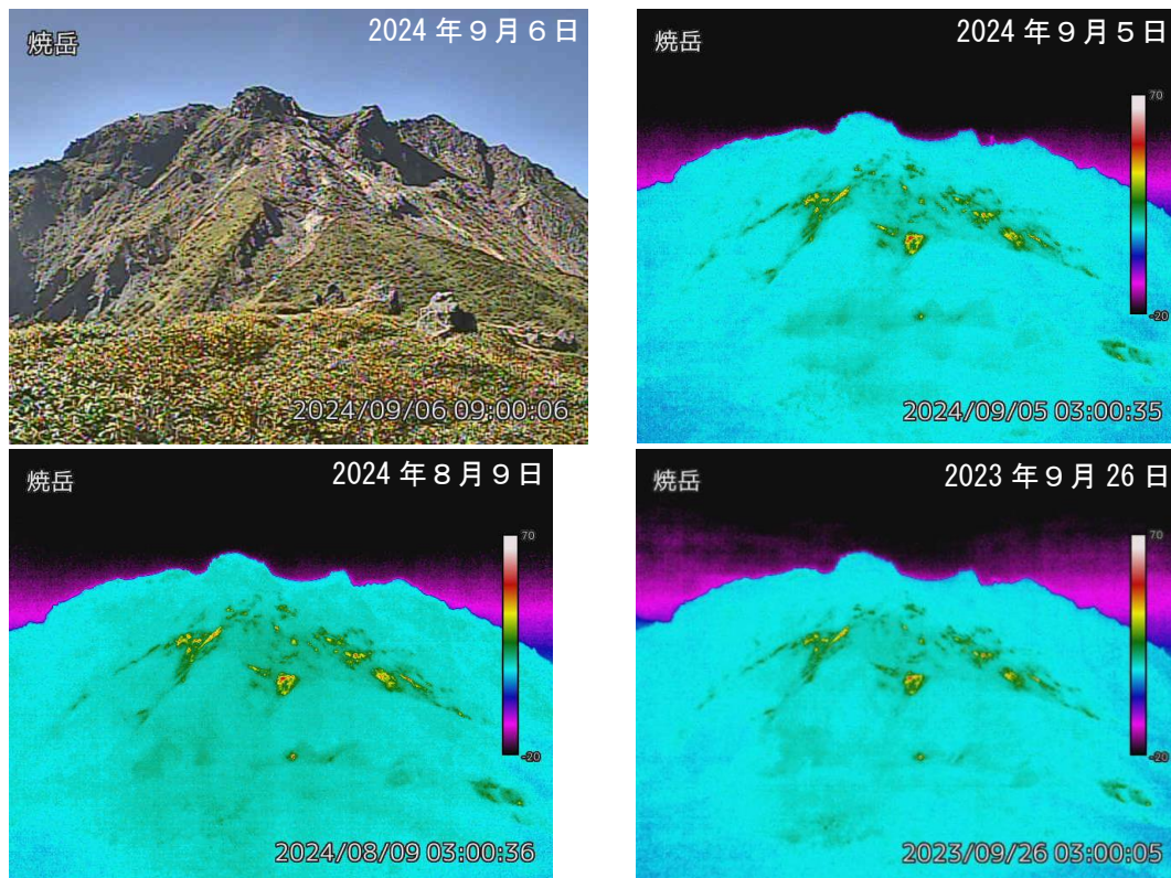
図4 焼岳 中尾峠赤外熱映像カメラによる焼岳の北側斜面の地表面温度分布と可視画像
