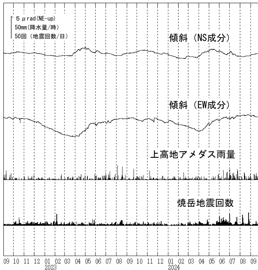
図8 焼岳 南峰南東観測点における傾斜データ（2022年9月1日～2024年9月30日）
