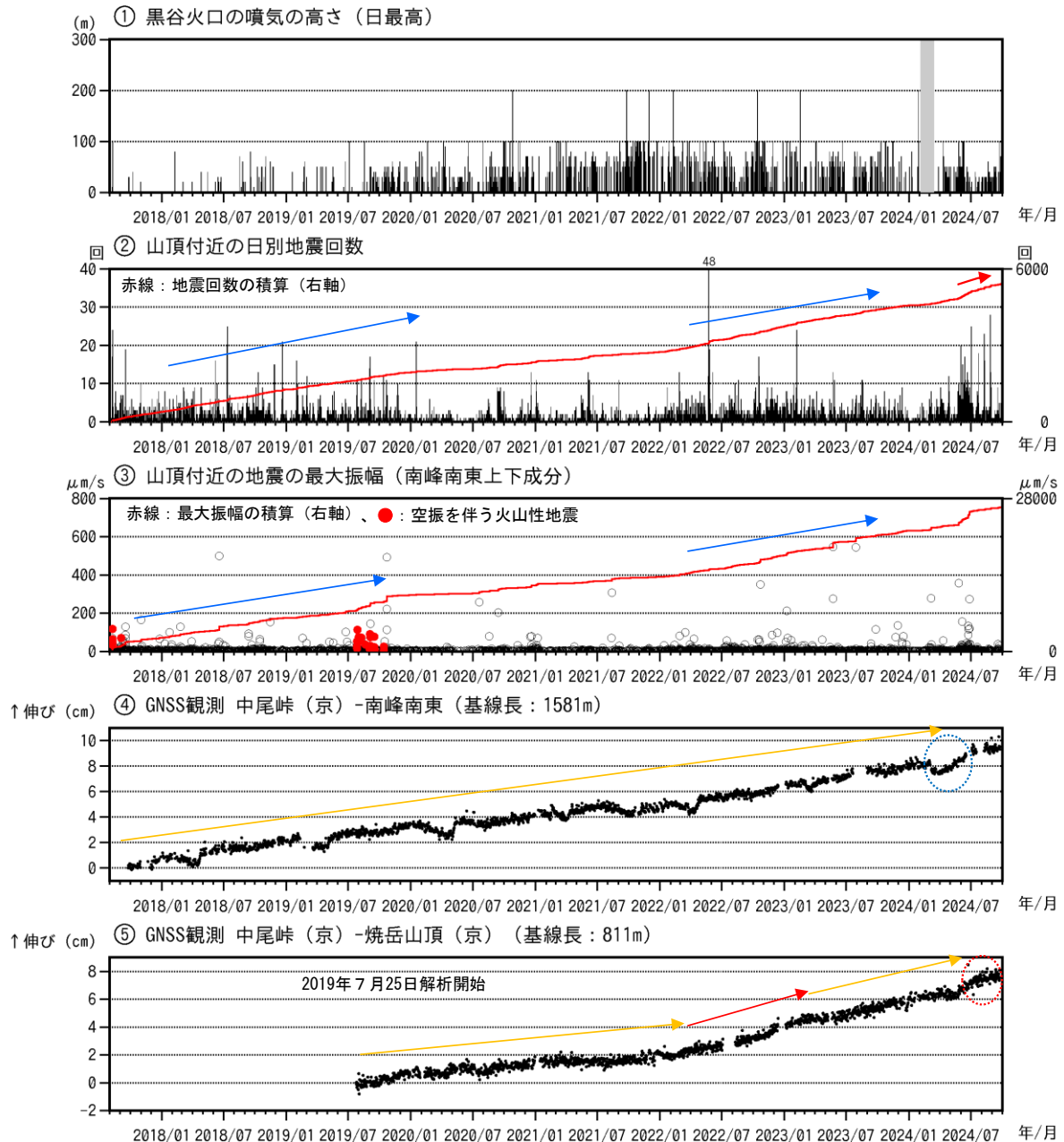
図1-1 焼岳 火山活動経過図（2017年8月1日～2024年9月30日）
