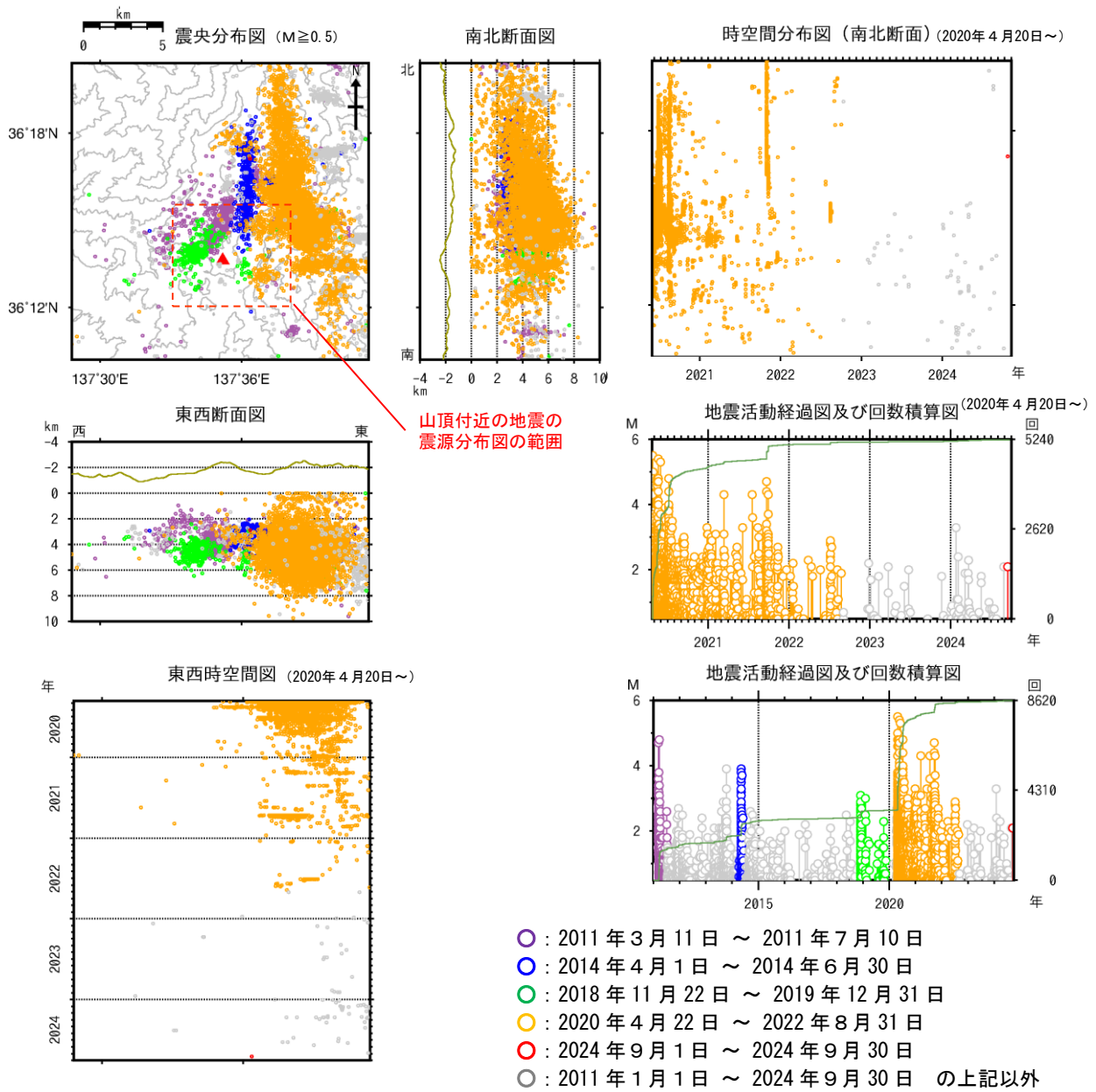
図9 焼岳 広域地震観測網による山体及び周辺の地震活動(2011年1月1日～2024年9月30日)
