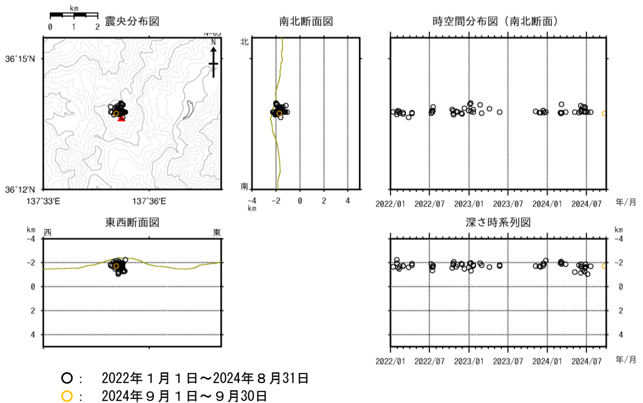
図2 焼岳 山頂付近の地震の震源分布図（2022年1月1日～2024年9月30日）
