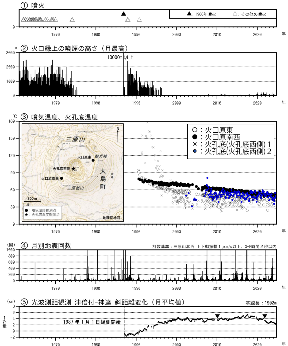
図1 伊豆大島 長期間の火山活動経過図（1961年1月～2024年9月30日）
