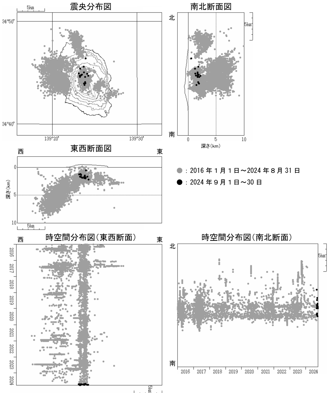
図4 伊豆大島 震源分布図（2016 年 1 月 1 日～2024 年 9 月 30 日）
