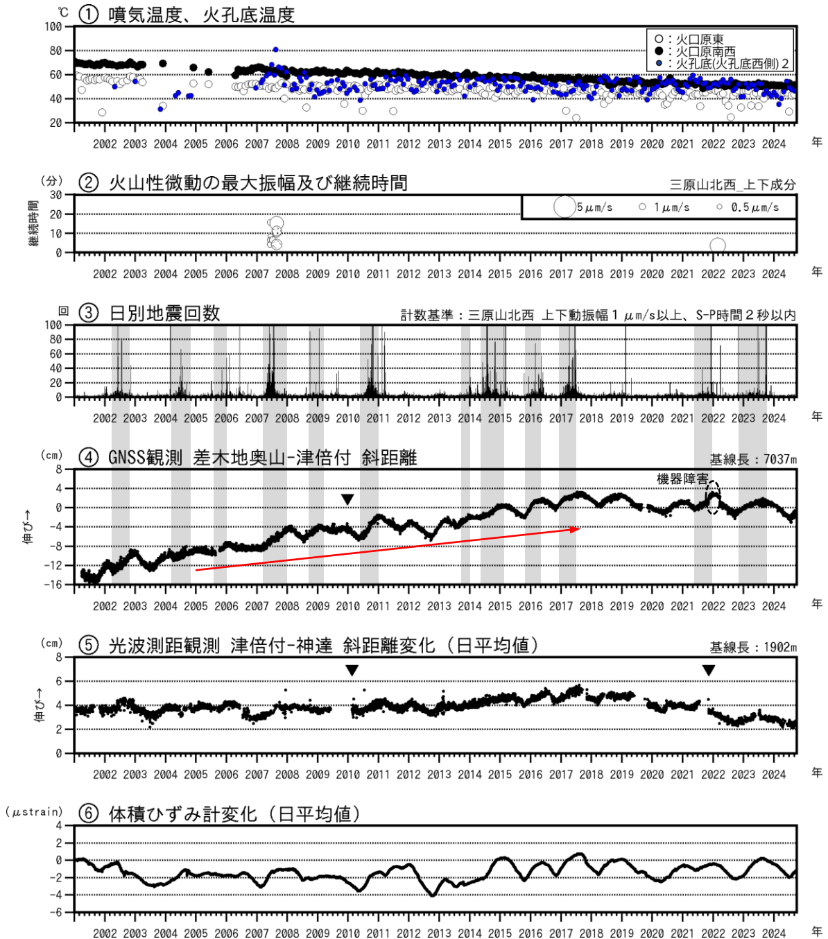
図2 伊豆大島 最近の火山活動経過図（2001年1月～2024年9月30日）
