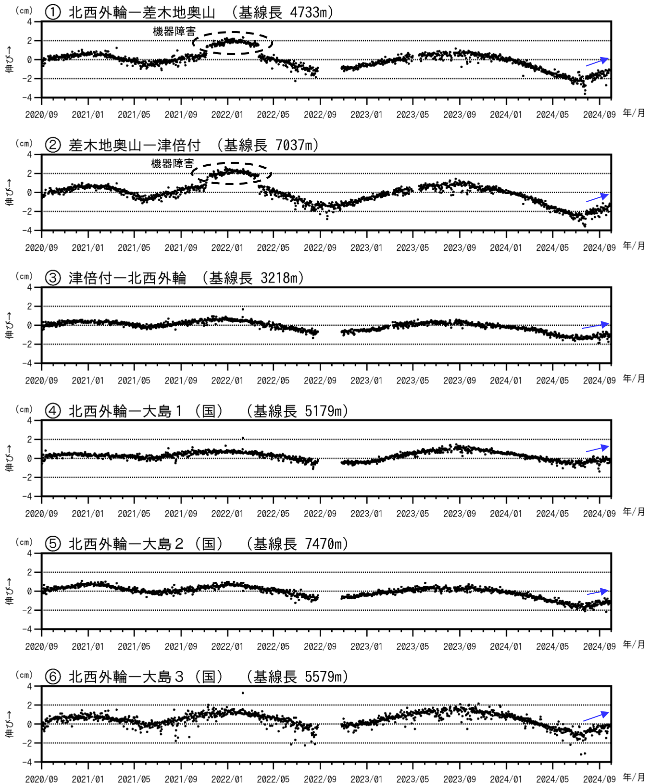
図3-2 伊豆大島 GNSS 連続観測による基線長変化(2020年9月～2024年9月30日)
