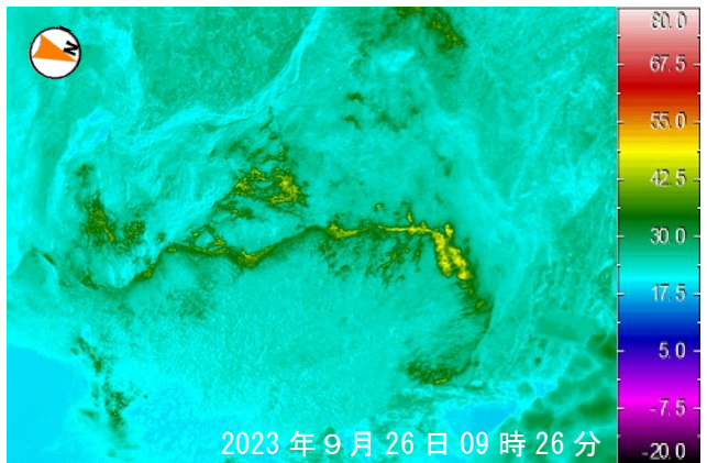
中央火孔東カメラ位置からの熱画像 （2023年9月26日 現地調査時に撮影）
