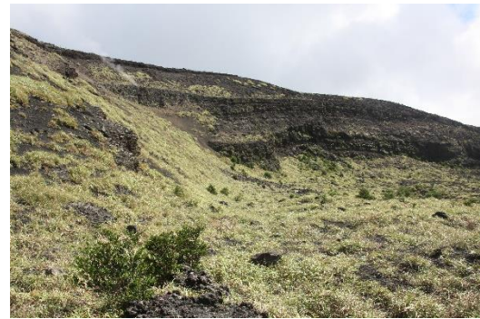
剣ガ峰付近（9月12日撮影）
