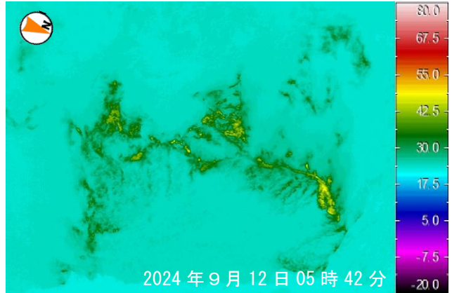
中央火孔東カメラ位置からの熱画像 （9月12日 現地調査時に撮影）
