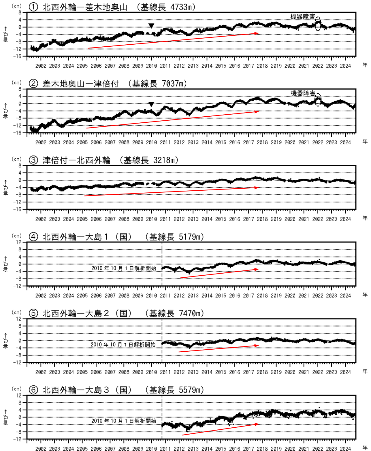
図3-1 伊豆大島 GNSS 連続観測による基線長変化(2001年1月～2024年9月30日)
