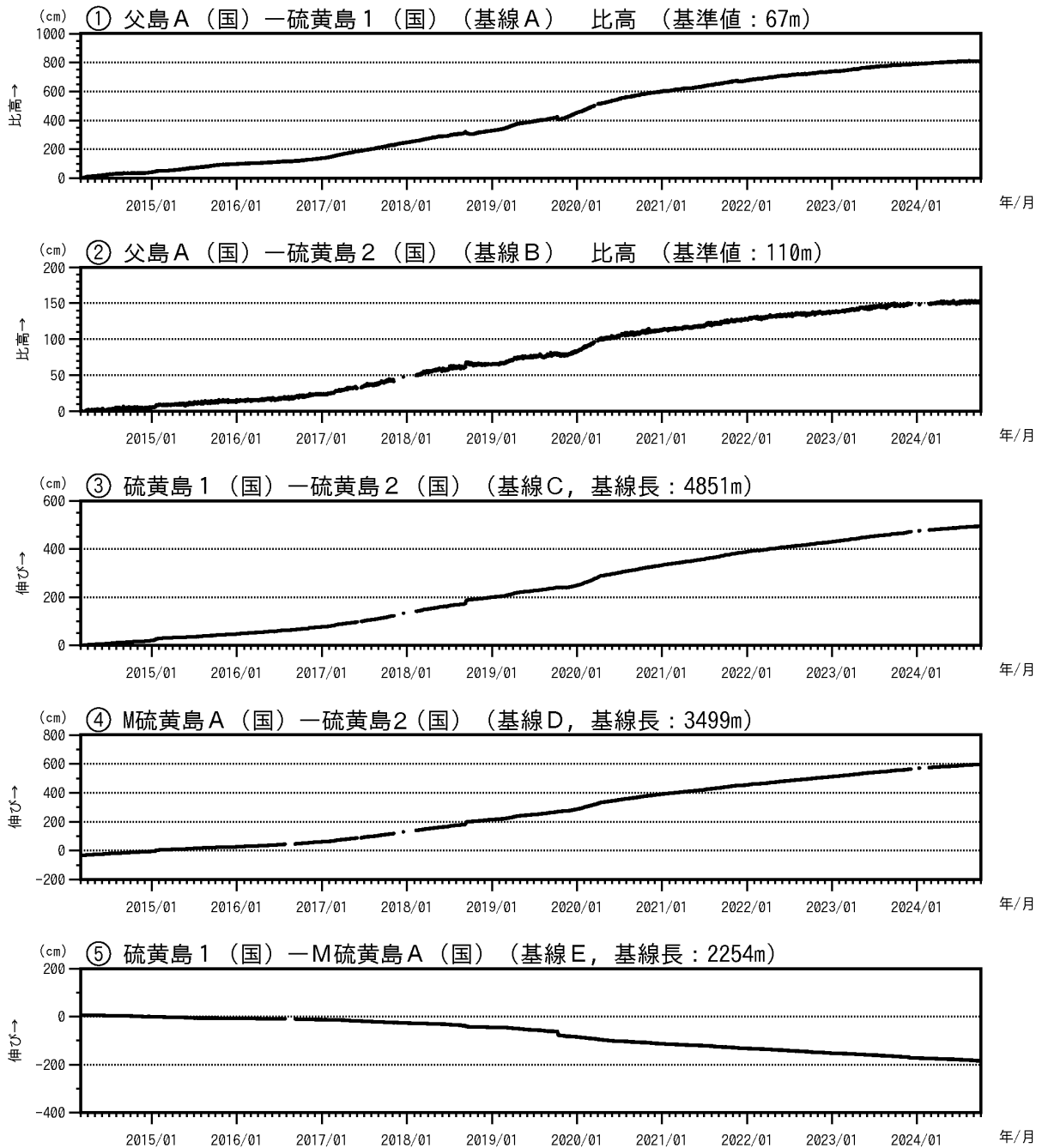
図6 硫黄島 GNSS 連続観測結果（2014年3月1日～2024年9月30日）
