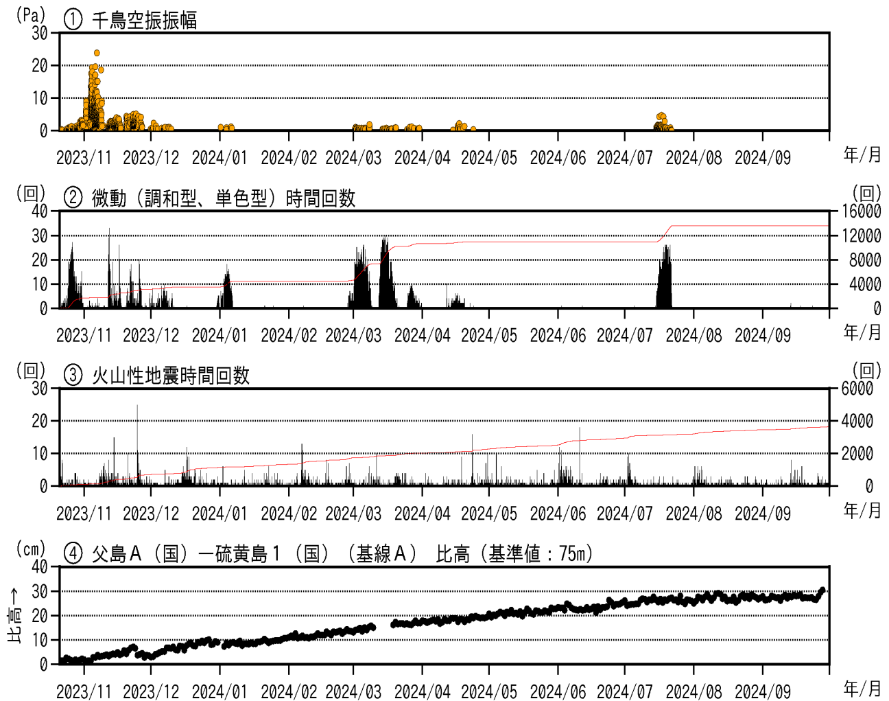
図4 硫黄島 火山活動経過図（2023年10月21日～2024年9月30日）
