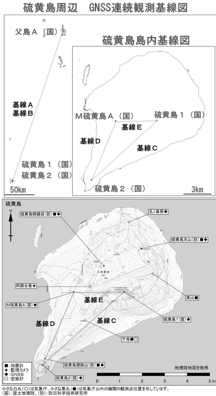
GNSS 基線（A～E）は図4、図5及び6の基線に対応しています。
