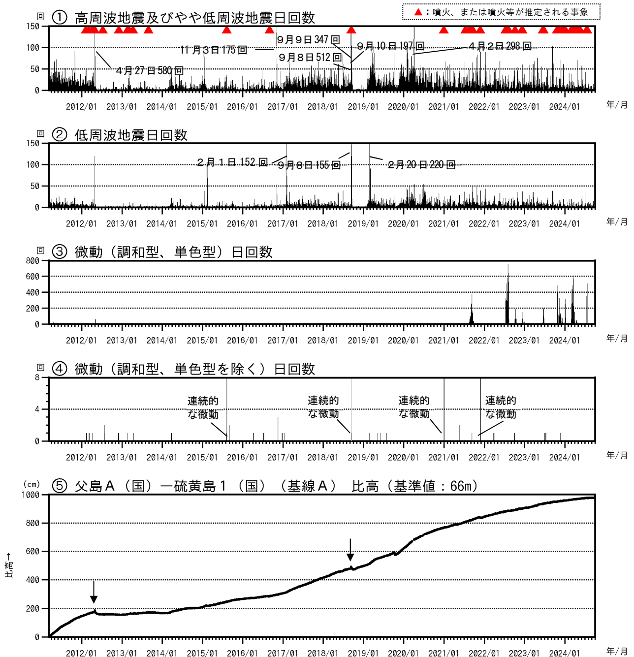
図5 硫黄島 火山活動経過図（2011年3月8日～2024年9月30日）
