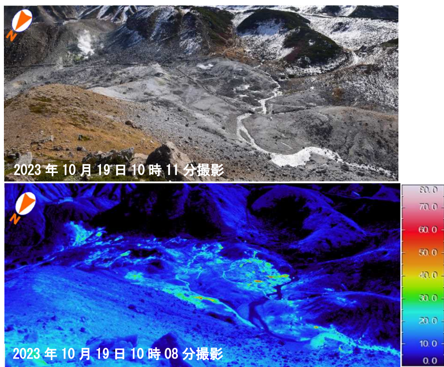
図2-3 弥陀ヶ原 地獄谷（鍛冶屋地獄及び百姓地獄）の状況（撮影位置及び撮影方向は図2-1参照）
