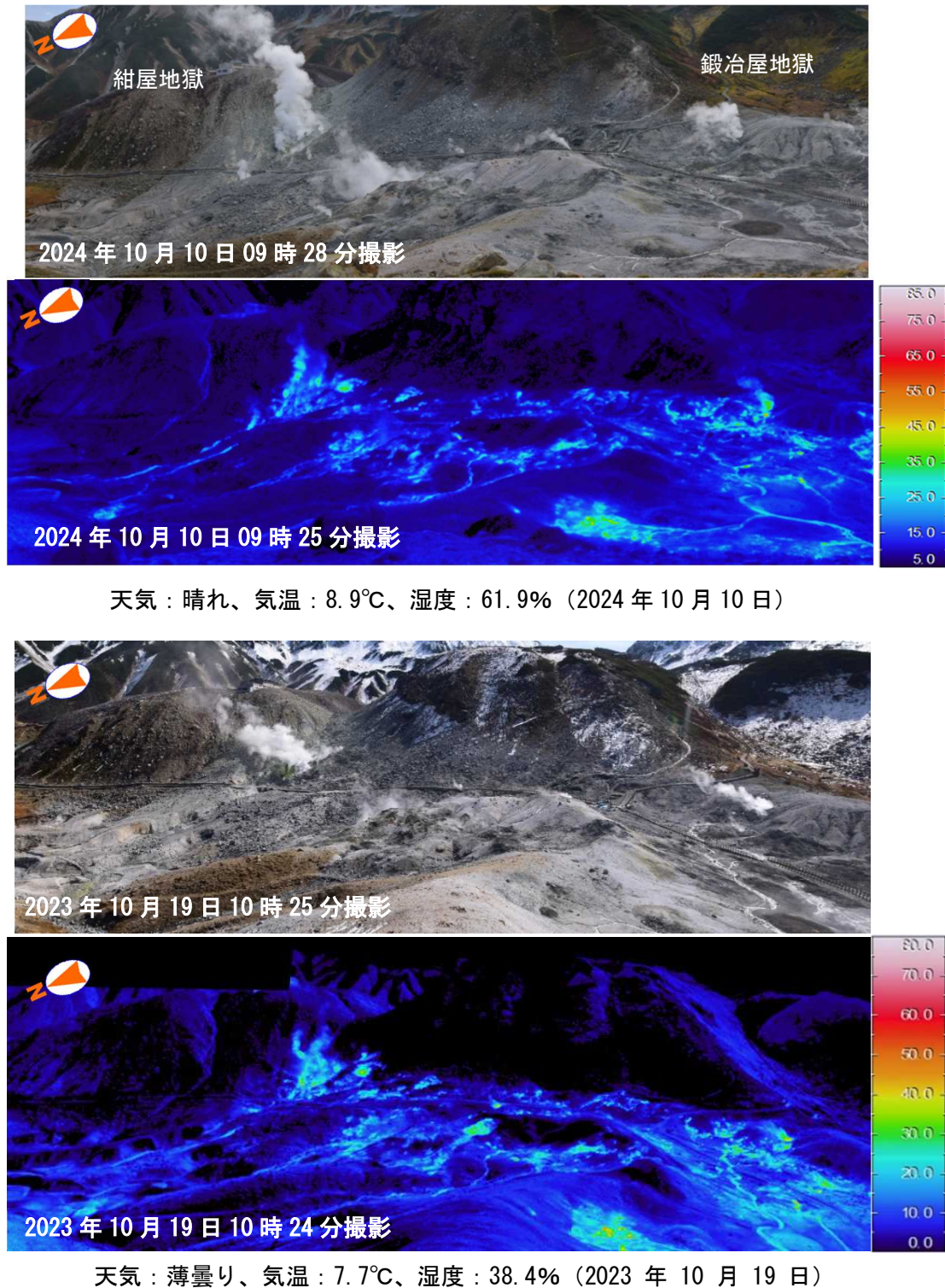
図 2-2 弥陀ヶ原 地獄谷（紺屋地獄及び鍛冶屋地獄）の状況（撮影位置及び撮影方向は図 2-1 参照）
