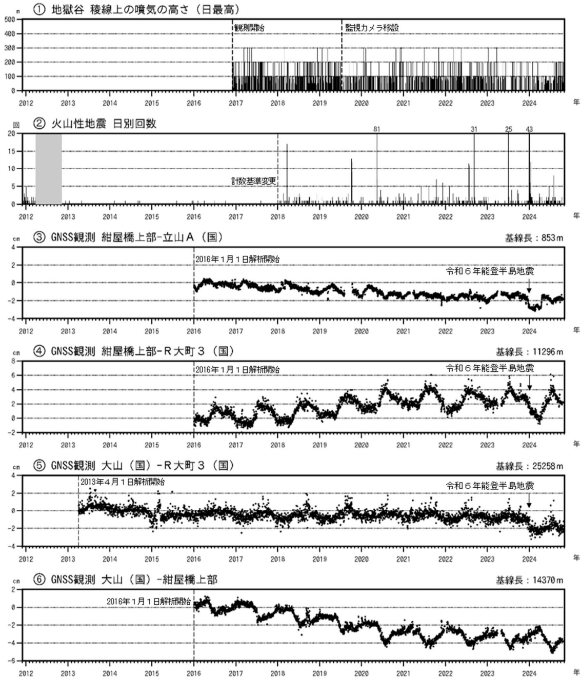
図4 弥陀ヶ原 火山活動経過図（2011年12月1日～2024年10月31日）
