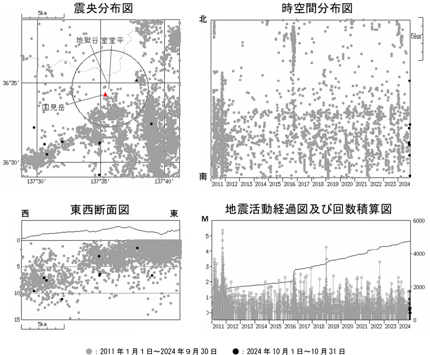
図3 弥陀ヶ原 広域地震観測網による山体・周辺の地震活動（2011 年 1 月 1 日～2024 年 10 月 31 日） 震央分布図中の円は弥陀ヶ原の計数対象地震（室堂平で S-P 時間 1 秒以内）のおよその範囲を示しています。 広域地震観測網により震源決定したもので、深さは全て海面以下として決定しています。 図中の震源要素は一部暫定値が含まれており、後日変更することがあります。 この図では、関係機関の地震波形を一元的に処理し、地震観測点の標高を考慮する等した手法で得られた震源を用いています（ただし、2020 年 8 月以前の地震については火山活動評価のための参考震源です）。
