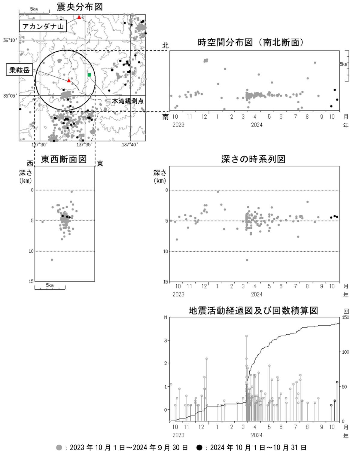
図3 乗鞍岳 広域地震観測網による山体・周辺の地震活動(2023 年 10 月 1 日～2024 年 10 月 31 日) M (マグニチュード) は地震の規模を表し、M0.2 以上の地震を表示しています。 広域地震観測網により震源決定したもので、深さは全て海面以下として決定しています。図中の震源要素は一部暫定値が含まれており、後日変更することがあります。 この図では、関係機関の地震波形を一元的に処理し、地震観測点の標高を考慮する等した手法で得られた震源を用いています。 東西断面図、時空間分布図、深さの時系列図、地震活動経過図及び回数積算図には、乗鞍岳付近（震央分布図中の黒線円の範囲）の地震を示しています。 ・ 3 月 29 日の乗鞍岳の南 2 km 付近を震源とする地震の発生以降、地震回数が増加していましたが、6 月以降はこの地震発生以前の地震回数と同程度となっています。
