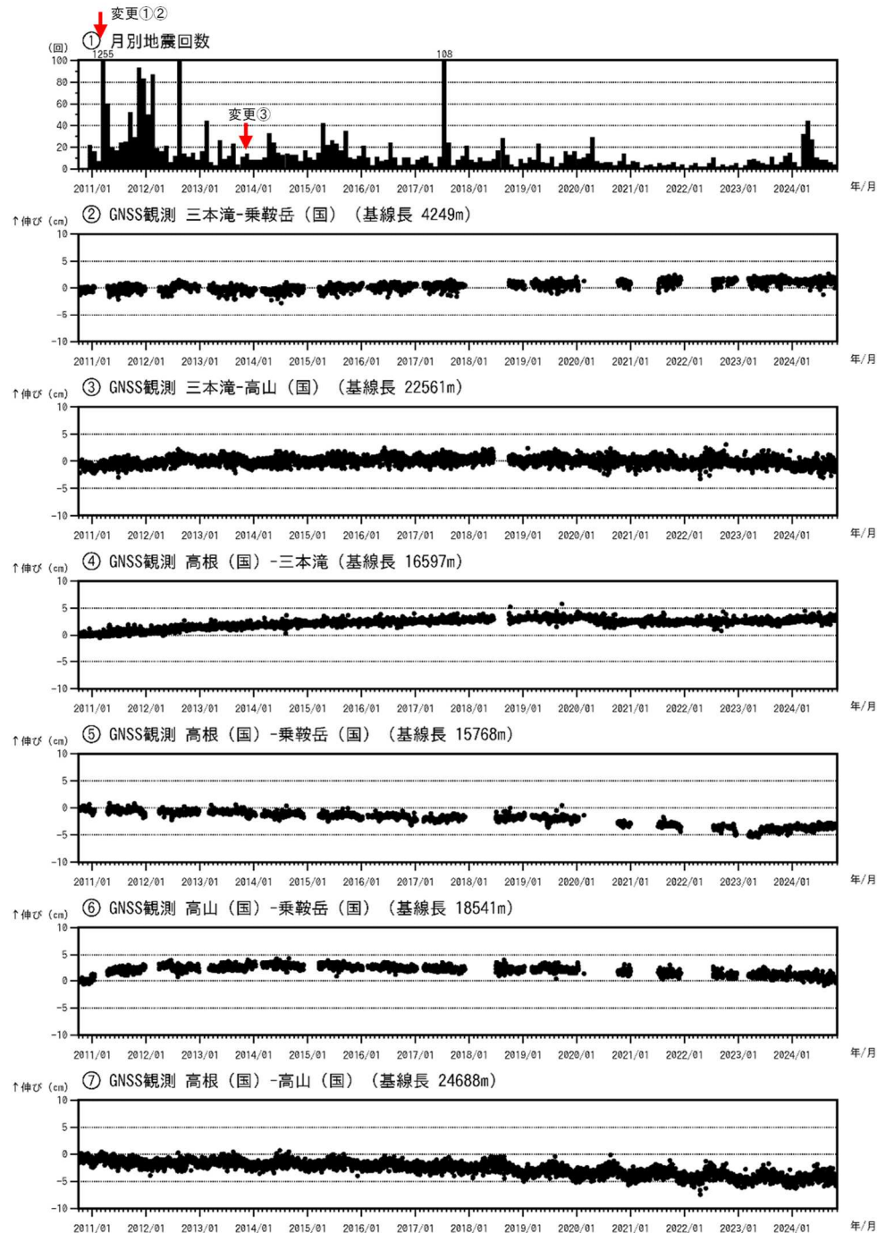
図2 乗鞍岳 火山活動経過図（2010年10月1日～2024年10月31日）
