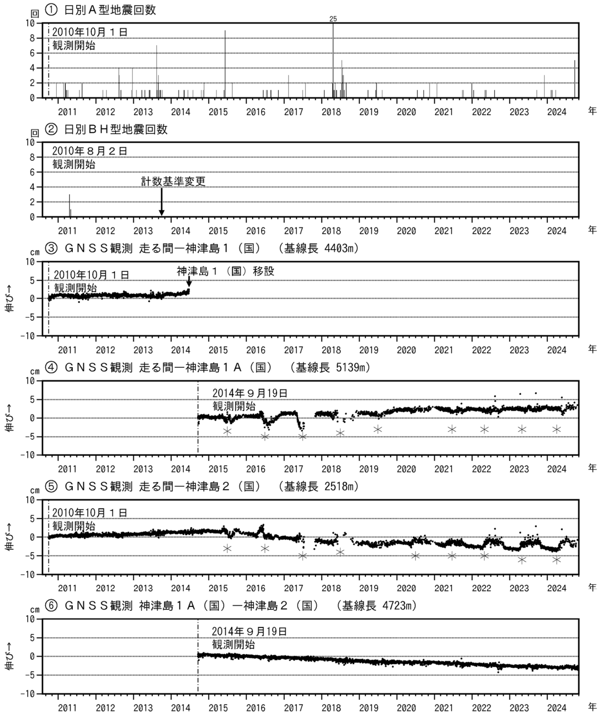
図2 神津島 火山活動経過図(2010年8月2日～2024年10月31日)
