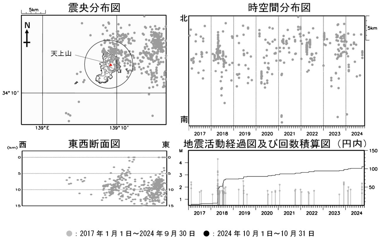
図3 神津島 広域地震観測網による山体・周辺の地震活動（2017年1月1日～2024年10月31日）
