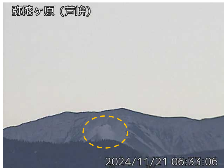
図1 弥陀ヶ原 地獄谷からの噴気の状況（橙丸）（11月21日、芦峠監視カメラによる）
