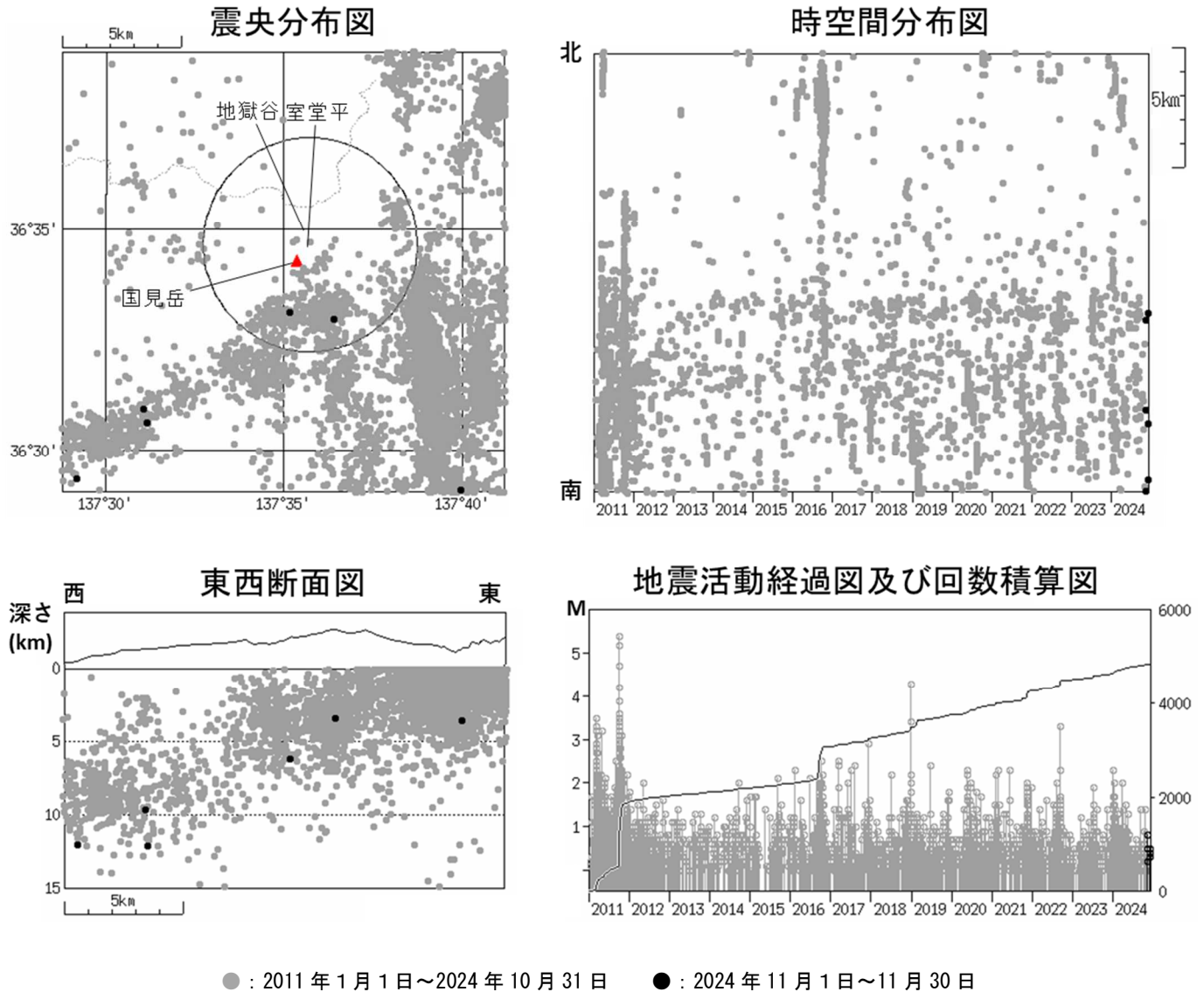
図2 弥陀ヶ原 広域地震観測網による山体・周辺の地震活動（2011 年 1 月 1 日～2024 年 11 月 30 日） 震央分布図中の円は弥陀ヶ原の計数対象地震（室堂平で S-P 時間 1 秒以内）のおよその範囲を示しています。 広域地震観測網により震源決定したもので、深さは全て海面以下として決定しています。なお、2020 年 9 月以降については、地震観測点の標高を考慮する等、震源決定の手法を変更しております。 図中の震源要素は一部暫定値が含まれており、後日変更することがあります。
