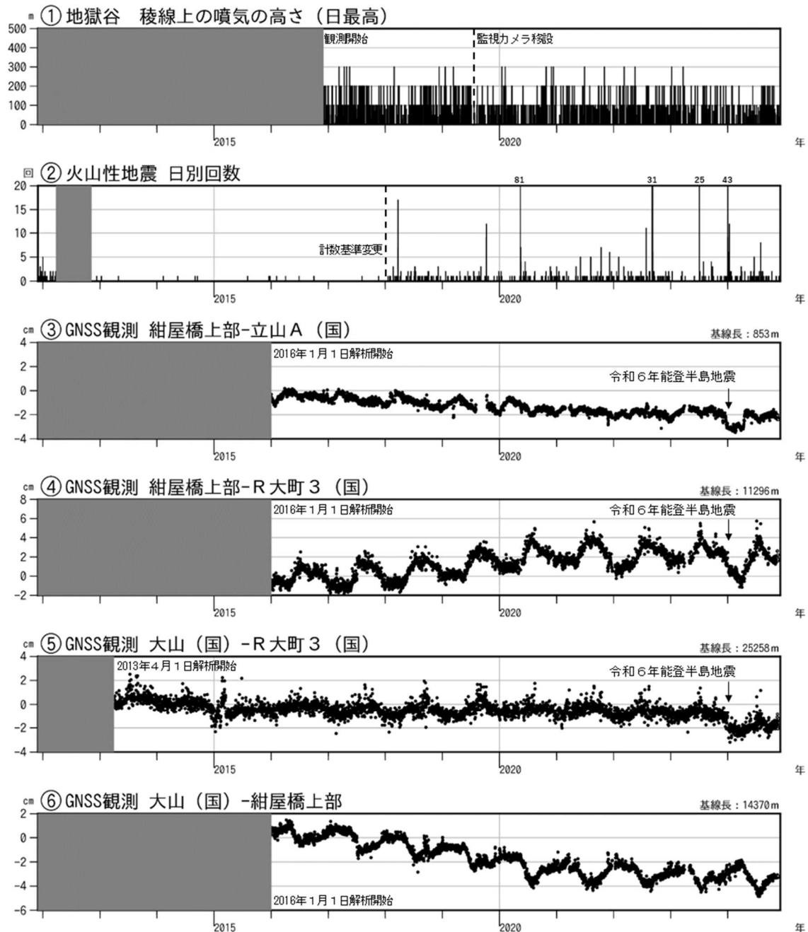
図3 弥陀ヶ原 火山活動経過図（2011年12月1日～2024年11月30日）
