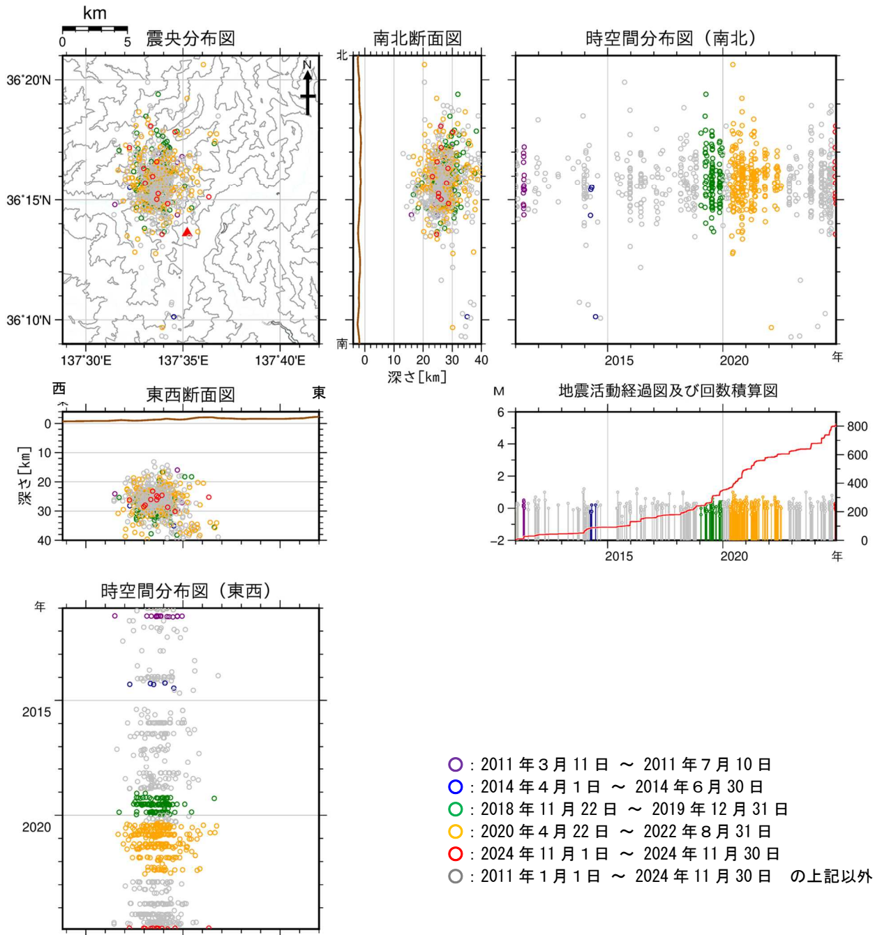
図10 焼岳 広域地震観測網による深部低周波地震の震源分布図（2011年1月1日～2024年11月30日） 広域地震観測網により震源決定したもので、深さは全て海面以下として決定しています。なお、2020年9月以降については、地震観測点の標高を考慮する等、震源決定の手法を変更しております。
