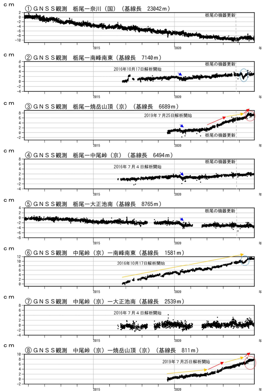
図6 焼岳 GNSS 連続観測による基線長変化（2010年10月1日～2024年11月30日）
