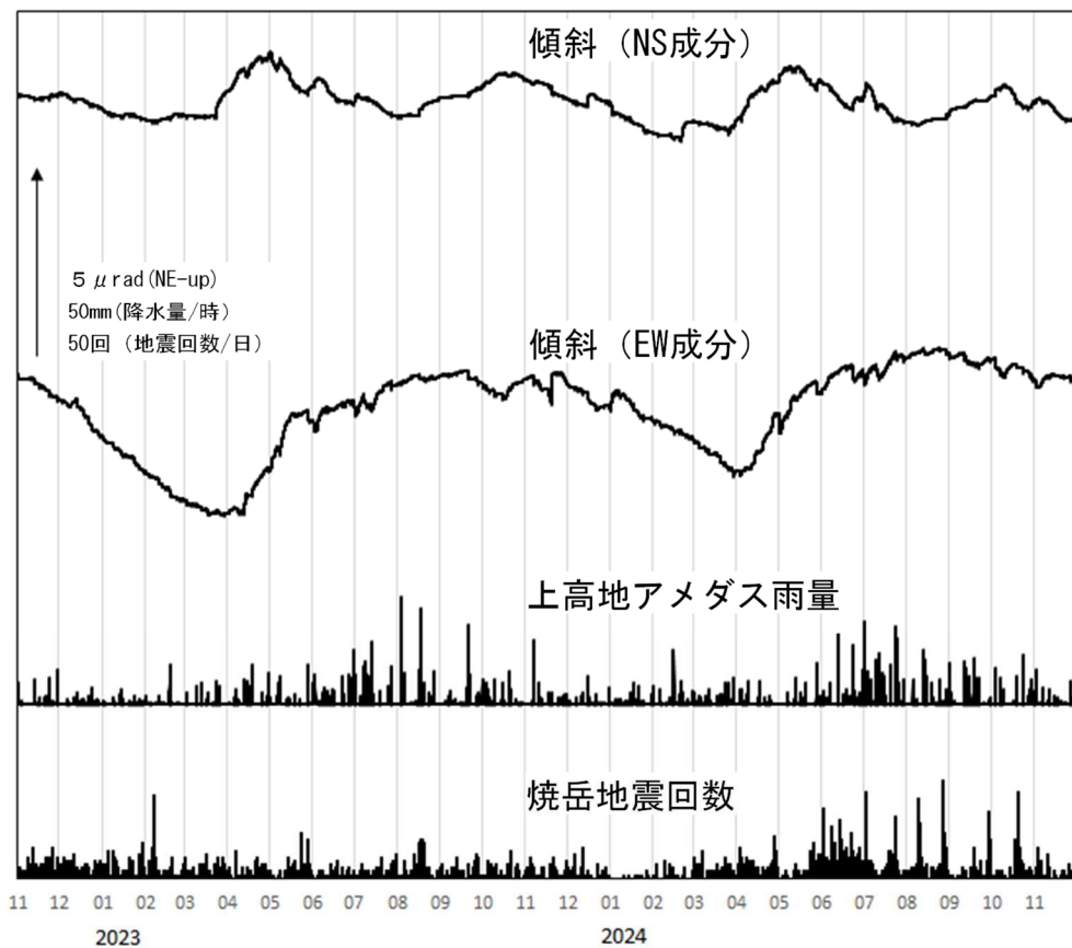
図8 焼岳 南峰南東観測点における傾斜データ（2022年10月1日～2024年11月30日）
