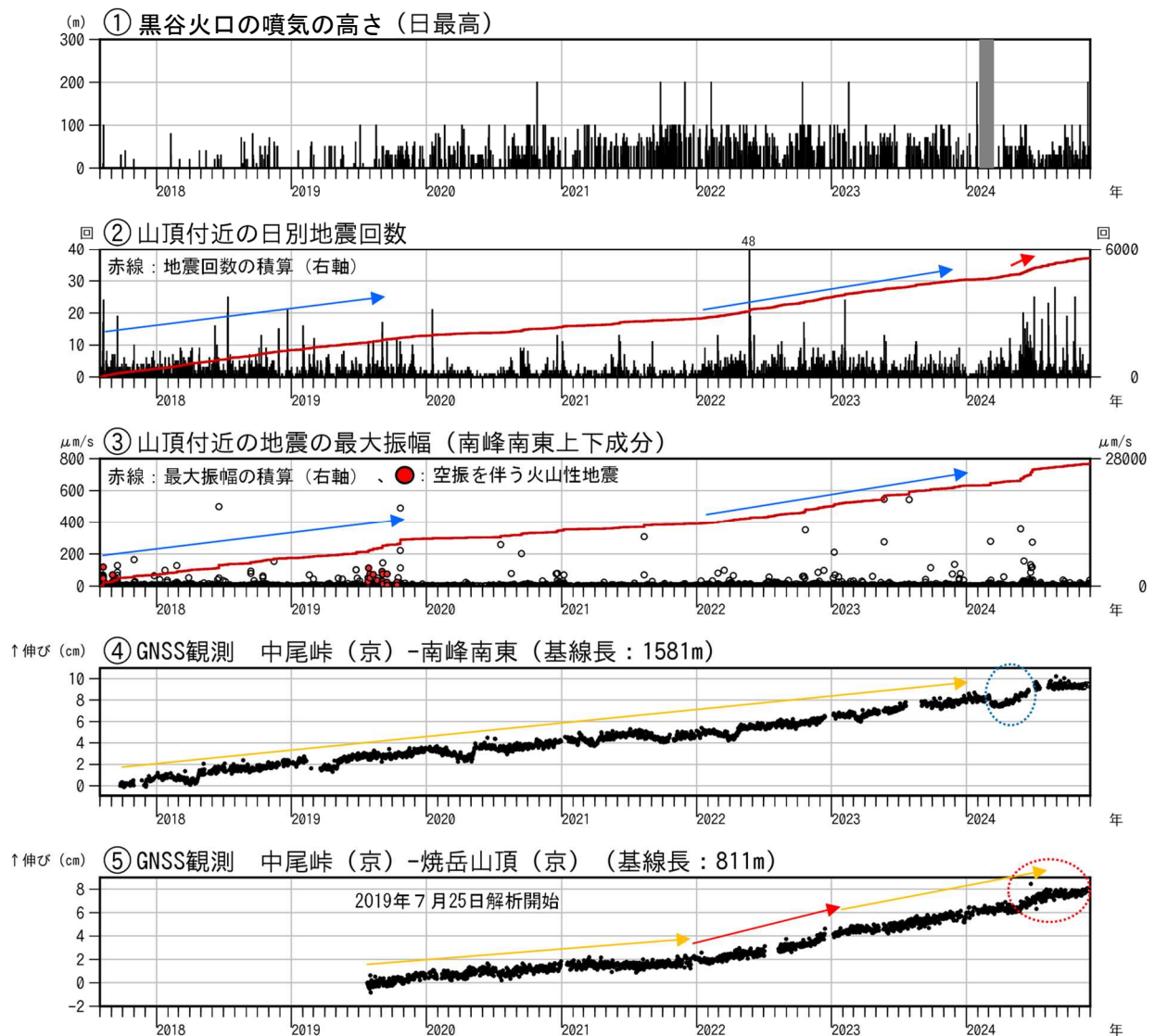
図1-1 焼岳 火山活動経過図（2017年8月1日～2024年11月30日）
