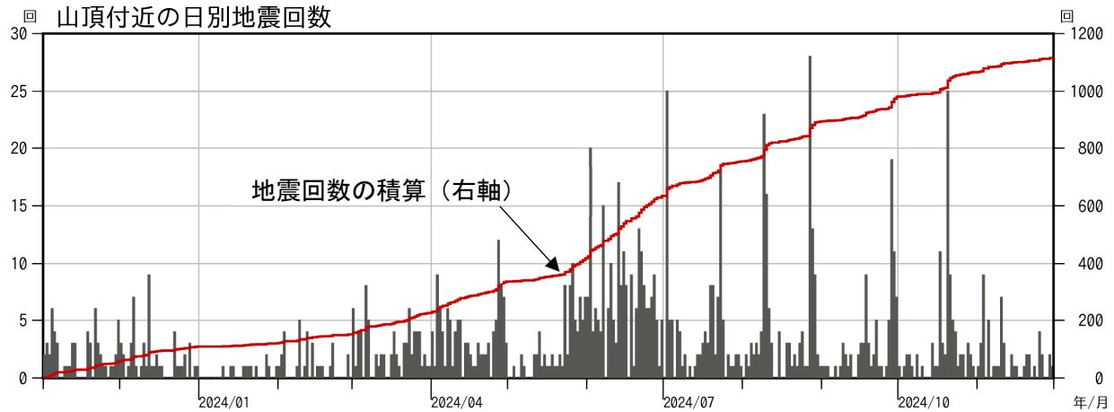
図1-2 焼岳 山頂付近の日別地震回数の推移（2023年11月1日～2024年11月30日）
