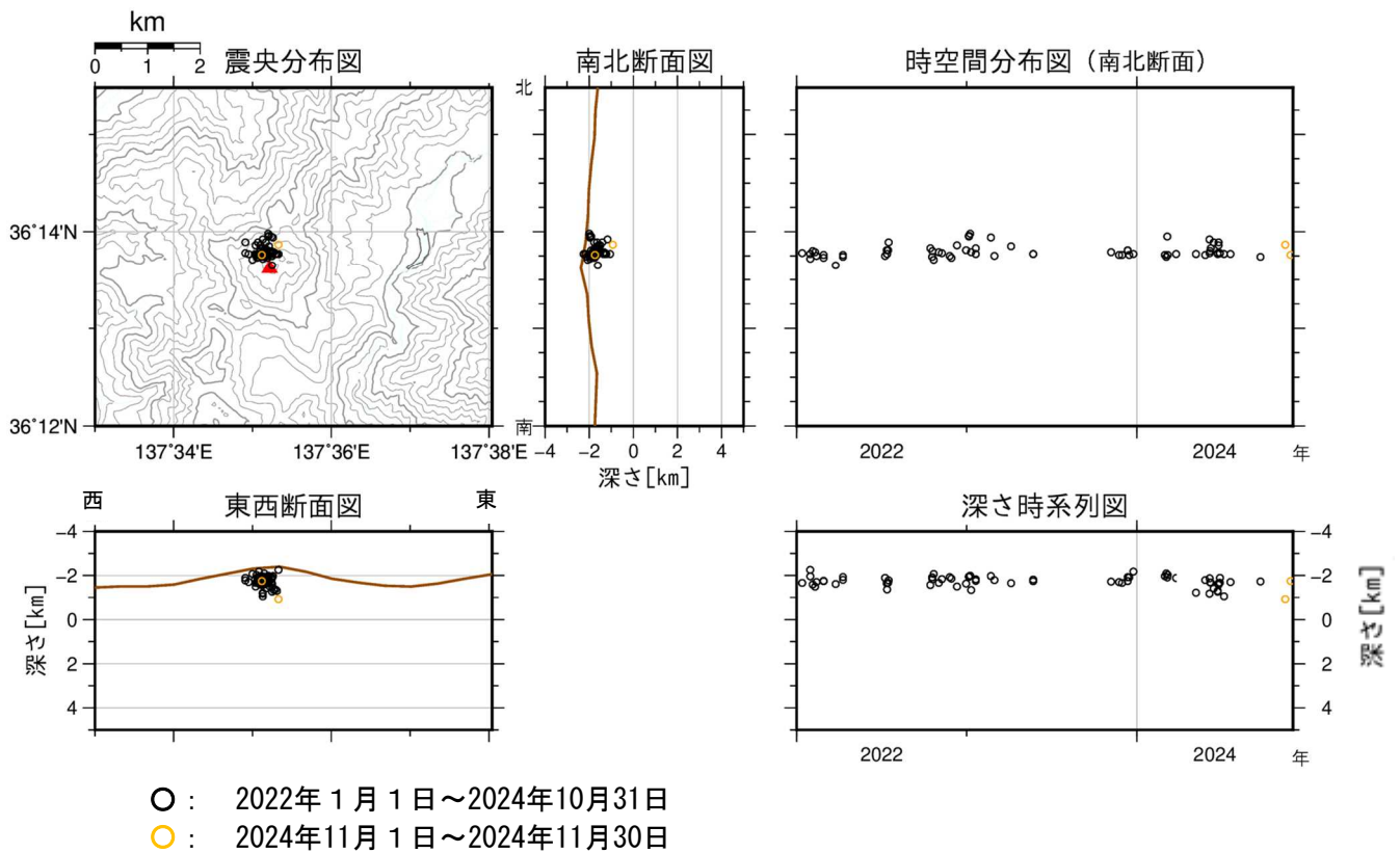
図2 焼岳 山頂付近の地震の震源分布図（2022年1月1日～2024年11月30日）
