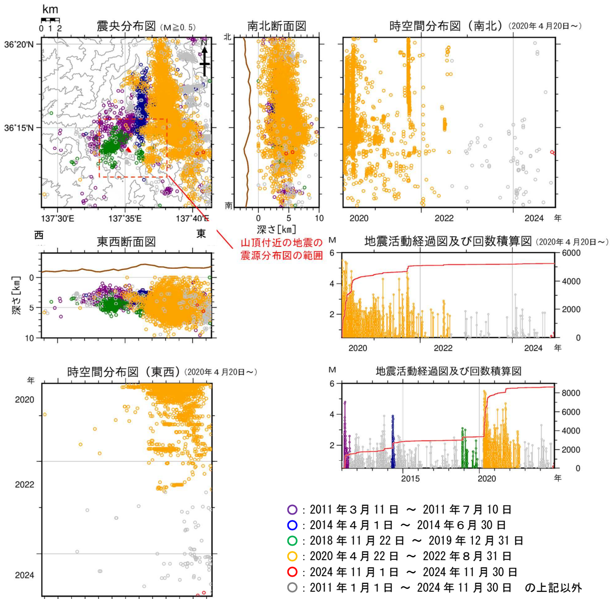
図9 焼岳 広域地震観測網による山体及び周辺の地震活動(2011年1月1日～2024年11月30日)
