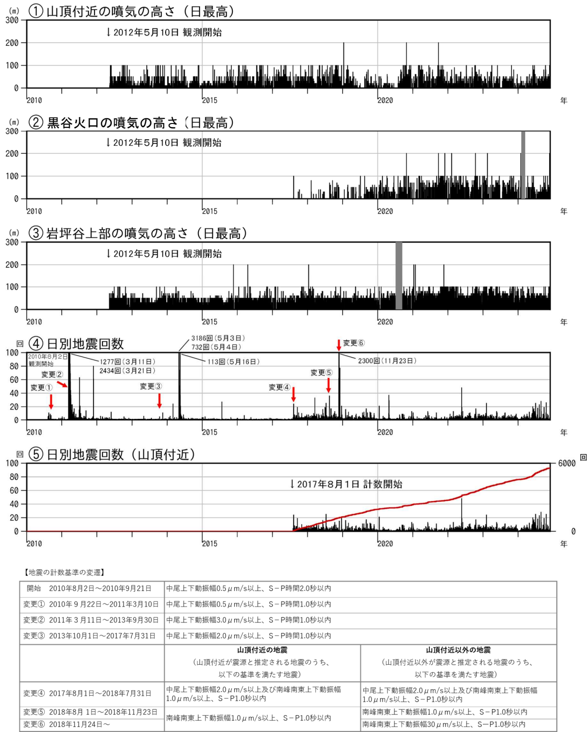
図5 焼岳 噴気の高さと地震回数の推移(2010年8月2日～2024年11月30日) ②黒谷火口の噴気の高さは、2024年2月5日から3月14日にかけて、障害のため欠測（灰色の期間）。 ③岩坪谷上部の噴気の高さは、2020年7月7日から9月10日にかけて、障害のため欠測（灰色の期間）。 ④2017年8月1日以降、山頂付近の地震と山頂付近以外の地震を分けて計数していますが、④ではこれらを合計した回数を示しています。図中の赤矢印は計数基準の変更を示しています。 ⑤山頂付近の日別地震回数（左軸）と日別地震回数の積算（右軸）を示しています。 ・黒谷火口では、2017年夏頃から噴気が時々観測されるようになり、2019年夏頃から噴気を観測する日が増えました。
