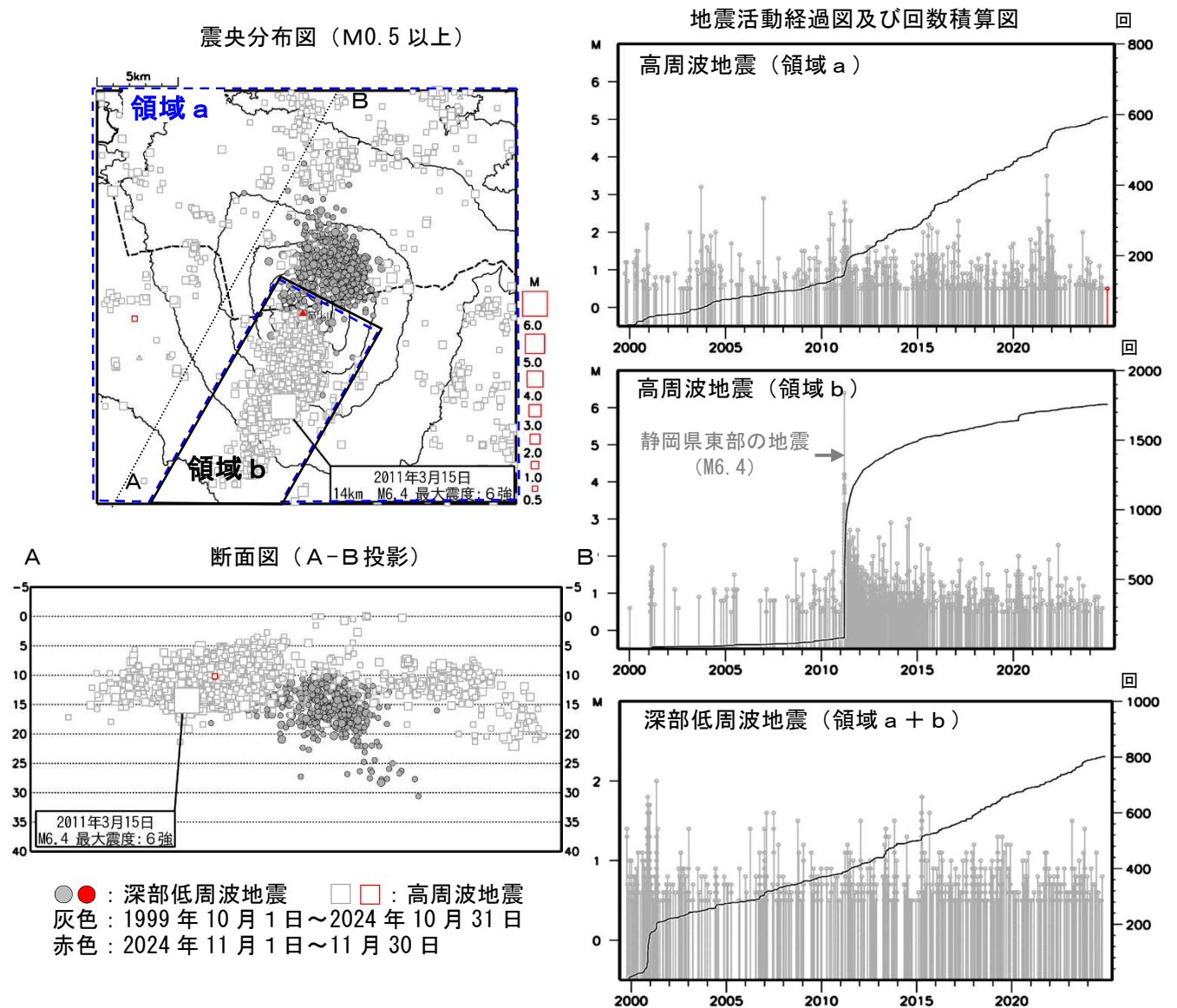
図3 富士山 広域地震観測網による山体及び周辺の地震活動（1999年10月1日～2024年11月30日） 広域地震観測網により震源決定したもの（M0.5 以上）で、深さは全て海面以下として決定しています。 M（マグニチュード）は地震の規模を表します。 図中の震源要素は一部暫定値が含まれており、後日変更することがあります。
