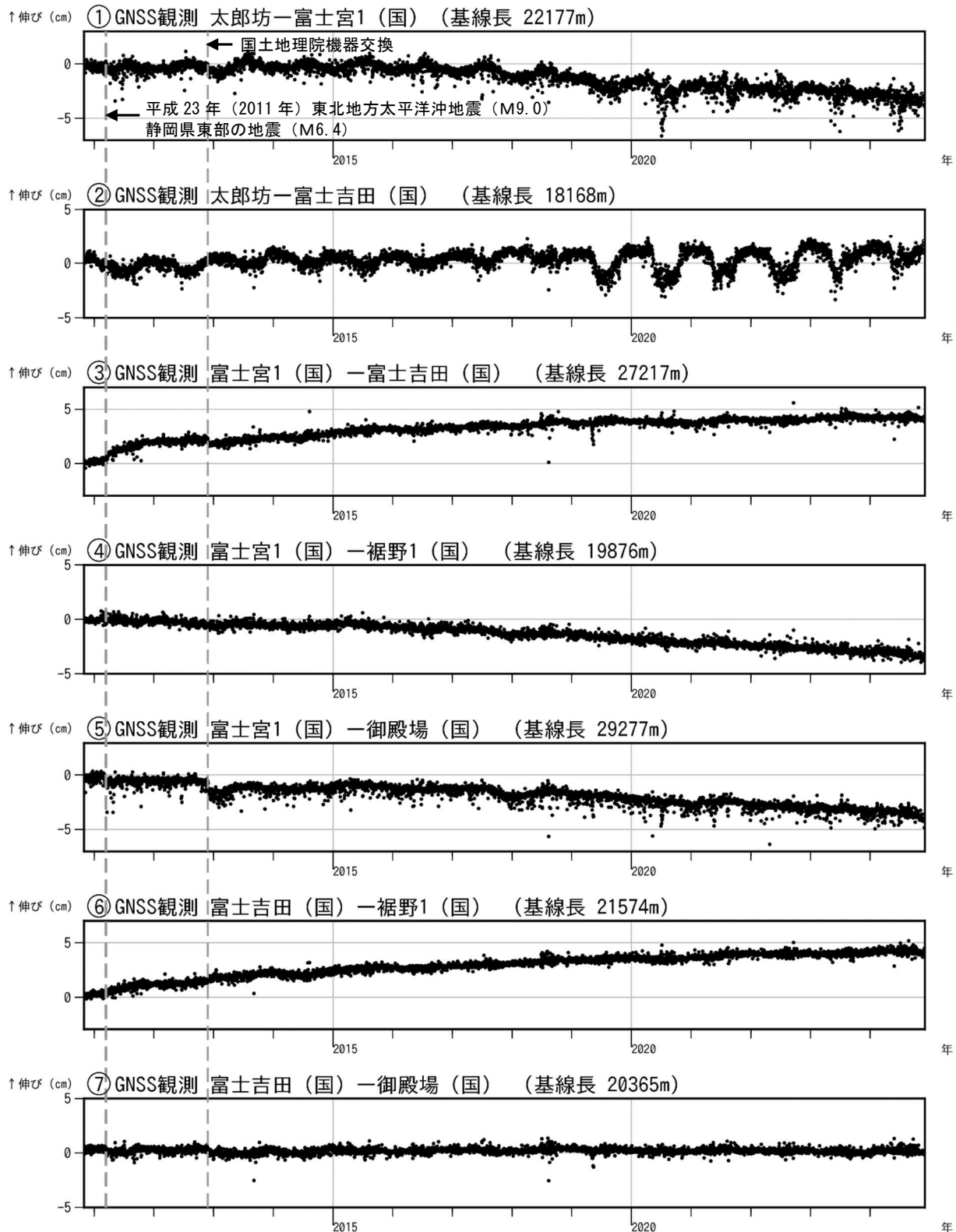
図4 富士山 GNSS 連続観測による基線長変化 (2010 年 10 月 1 日～2024 年 11 月 30 日)
