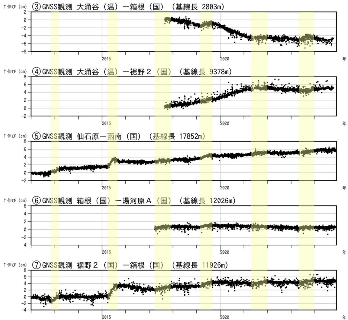
図3-2 箱根山 GNSS 連続観測による 基線長変化及び観測点配置図 (2012年1月1日～2024年11月30日)
