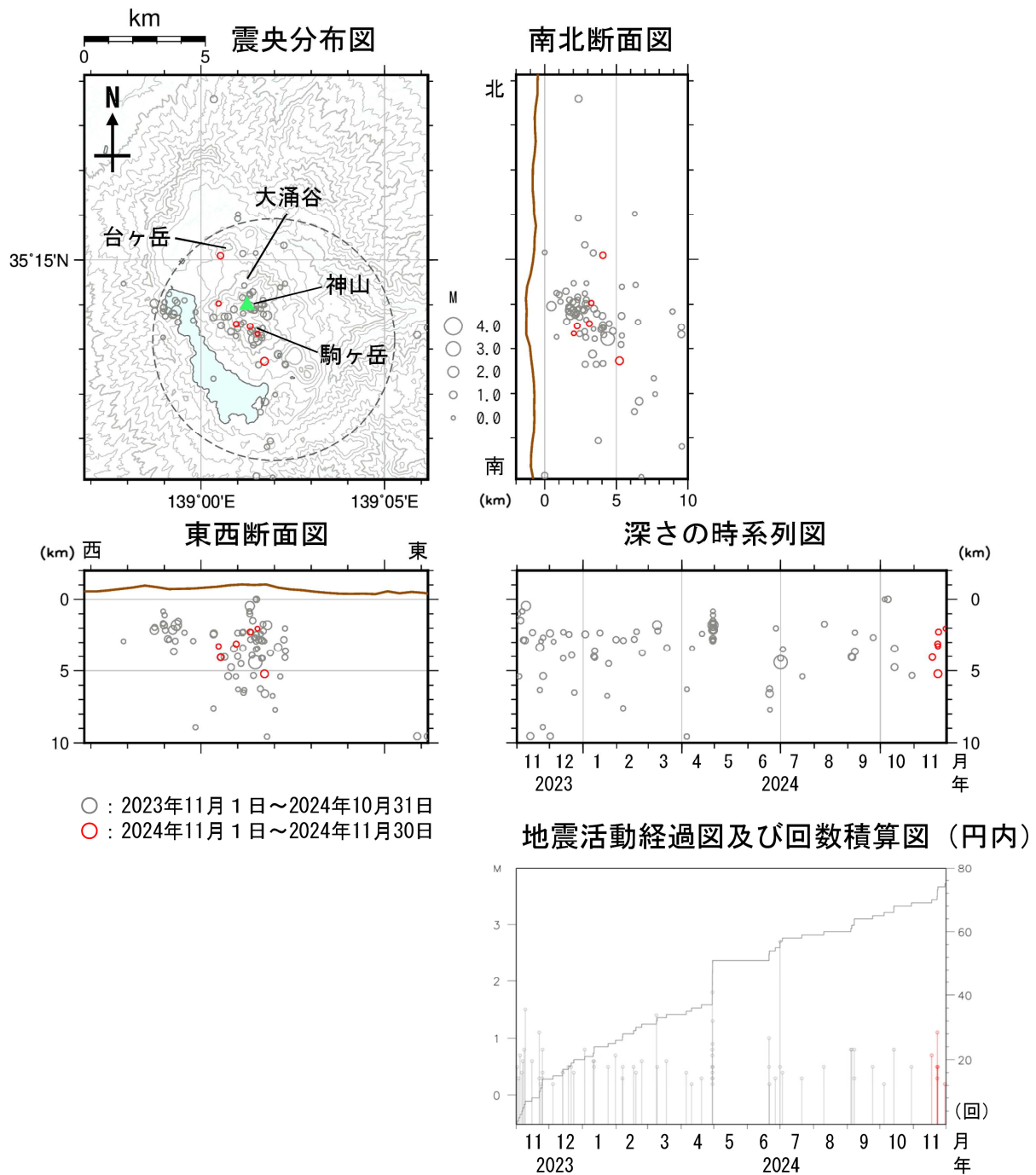
図4 箱根山 広域地震観測網による山体周辺の震源分布図（2023年11月1日～2024年11月30日）
