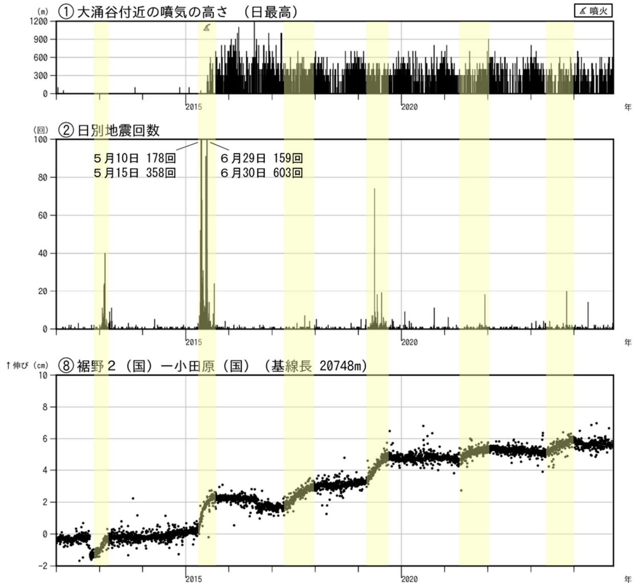
図3-1 箱根山 火山活動経過図（2012年1月1日～2024年11月30日）
