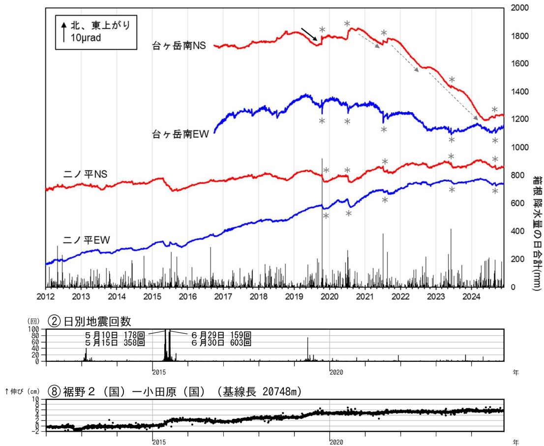
図5 箱根山 傾斜観測及び地震回数・GNSS観測（2012年1月1日～2024年11月30日）
