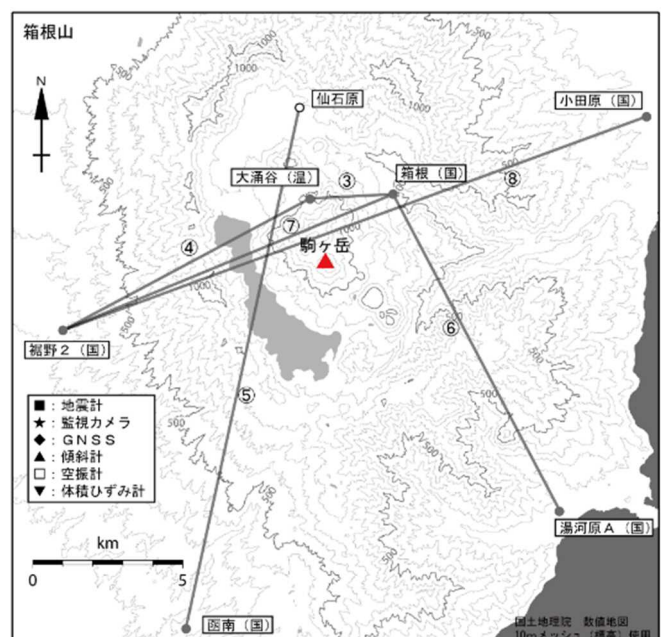
図3-2 箱根山 GNSS 連続観測による 基線長変化及び観測点配置図 (2012年1月1日～2024年11月30日)
