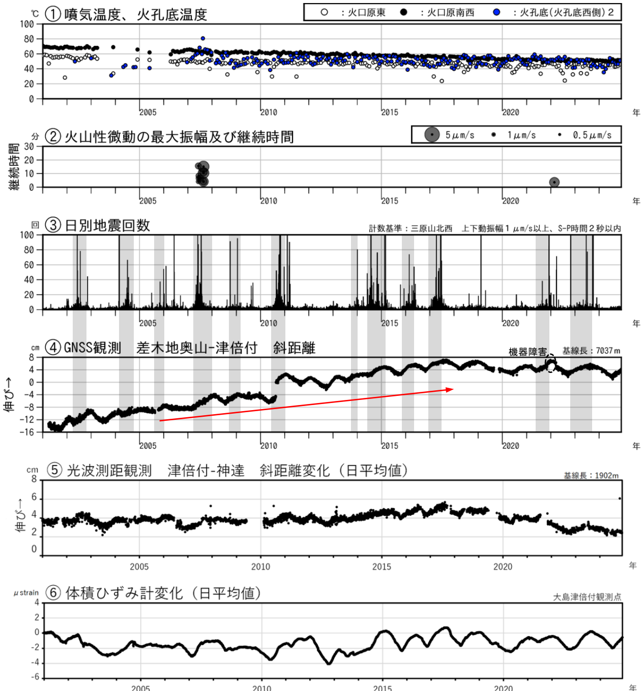
図2 伊豆大島 最近の火山活動経過図（2001年1月～2024年11月30日）
