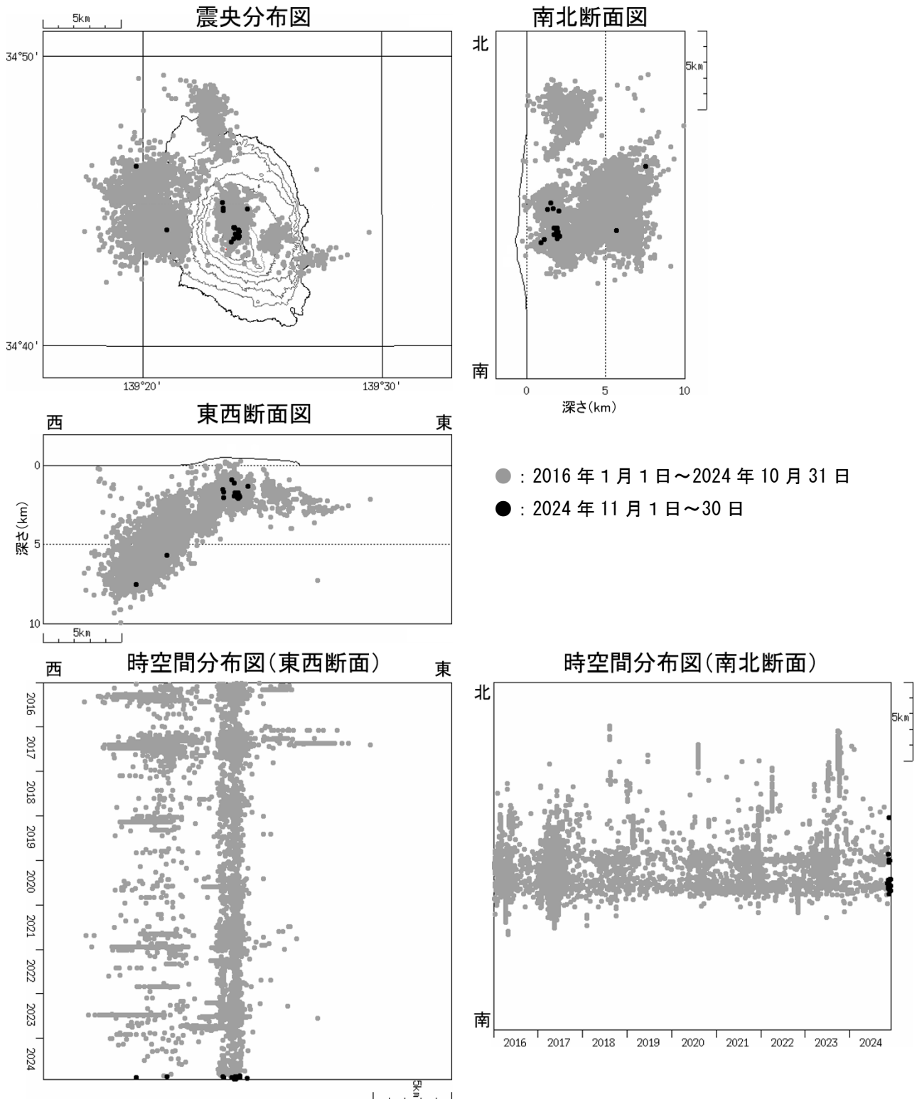
図4 伊豆大島 震源分布図（2016 年 1 月 1 日～2024 年 11 月 30 日）
