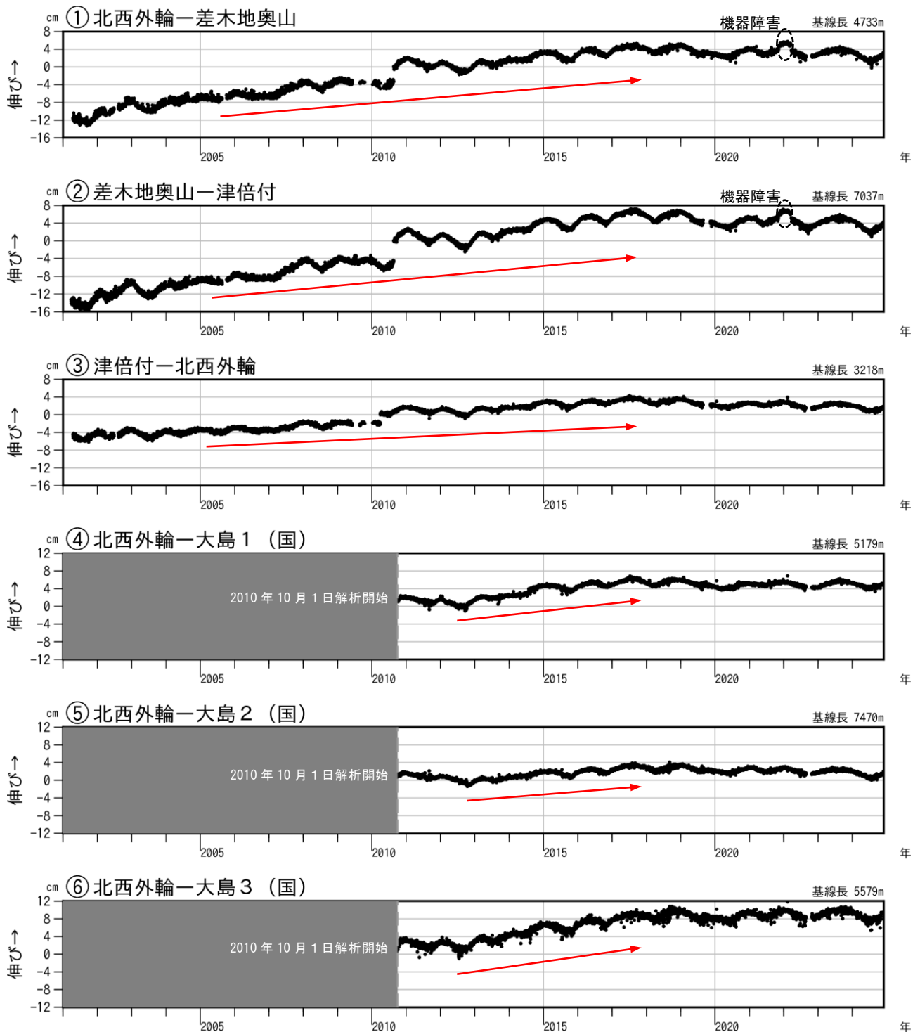
図 3-1 伊豆大島 GNSS 連続観測による基線長変化 (2001 年 1 月～2024 年 11 月 30 日)
