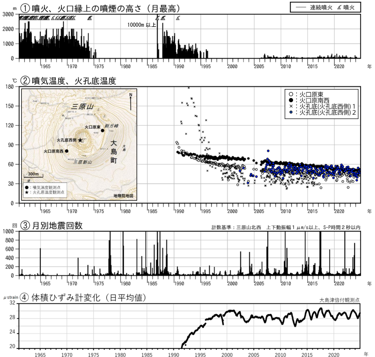
図1 伊豆大島 長期間の火山活動経過図（1961年1月～2024年11月30日）
