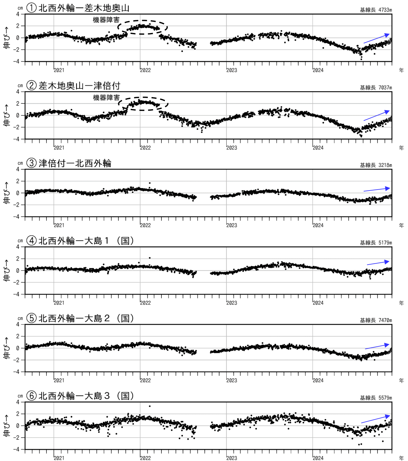
図3-2 伊豆大島 GNSS 連続観測による基線長変化(2020年9月～2024年11月30日)
