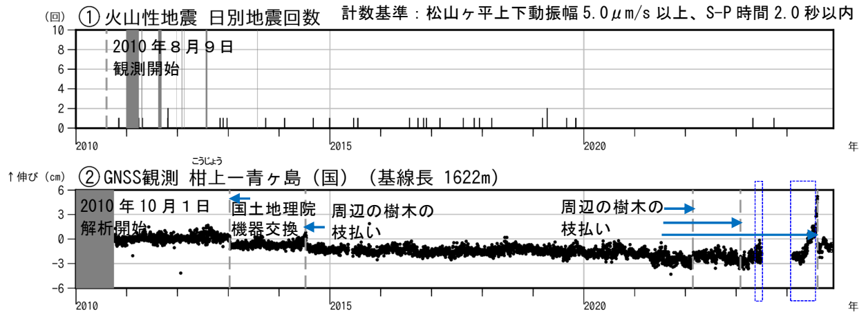
図2 青ヶ島 火山活動経過図 (2010年8月9日～2024年11月30日)
