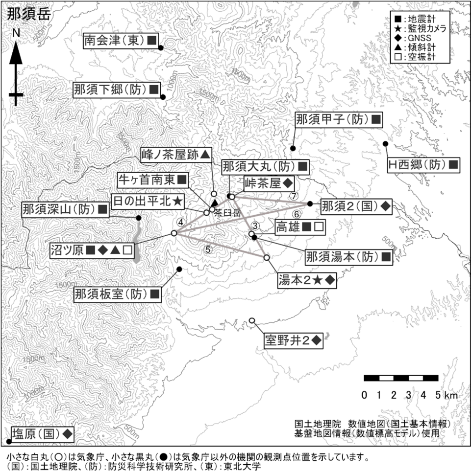
図6 那須岳 観測点配置図 GNSS 基線③～⑦は図4の③～⑦に対応しています。
