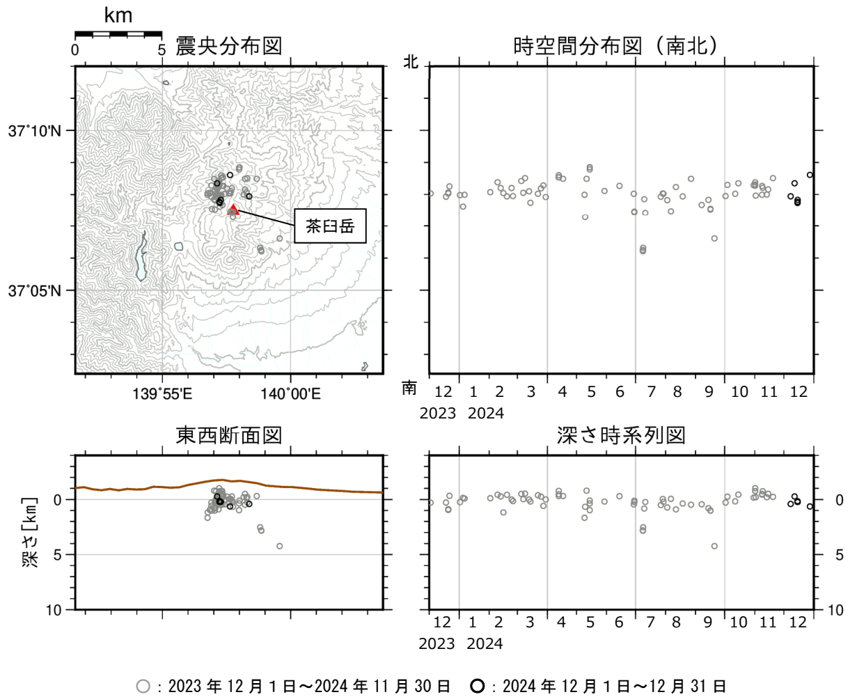
図5 那須岳 震源分布図（2023 年 12 月 1 日～2024 年 12 月 31 日）
