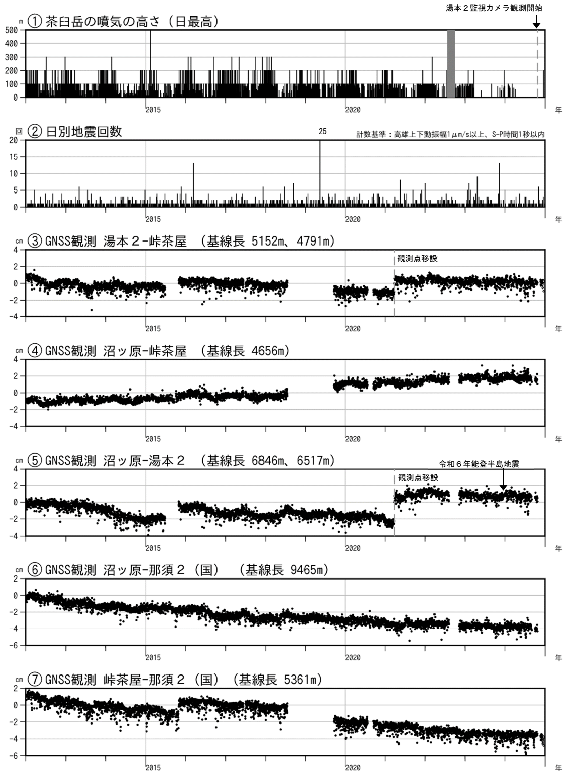
図4 那須岳 火山活動経過図（2012年1月1日～2024年12月31日）
