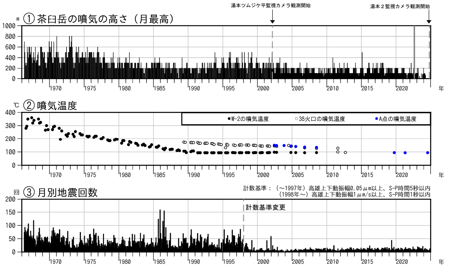
図3-1 那須岳 火山活動経過図（1966年6月～2024年12月）
